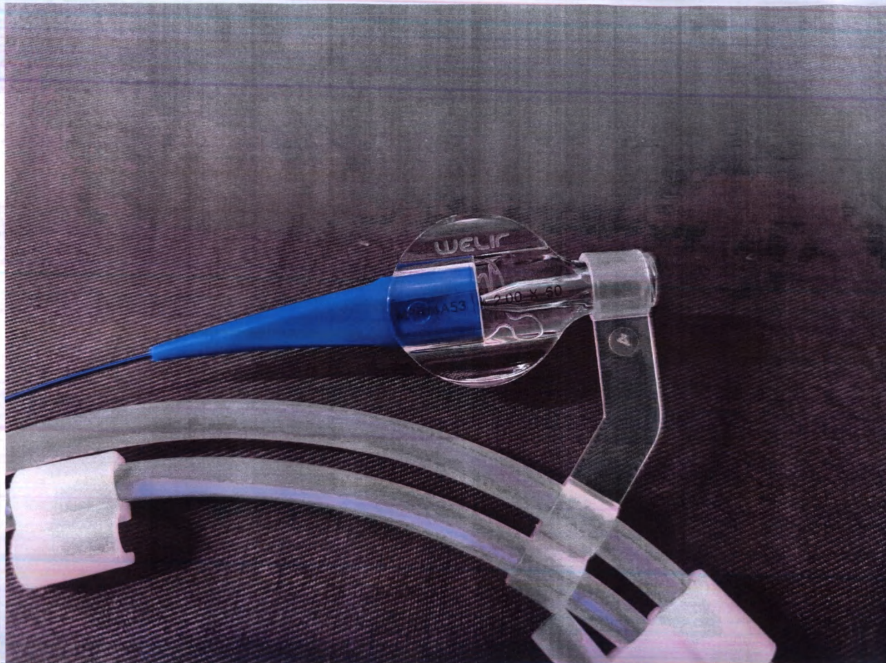
Рис. 21. Катетер дилатационный баллонный Mozec PTA Rx 0.014" для чрескожной транслюминальной ангиопластики (ЧТА), эффективная длина 150 см, диаметр x длина баллона 2,00 x 60 мм.
