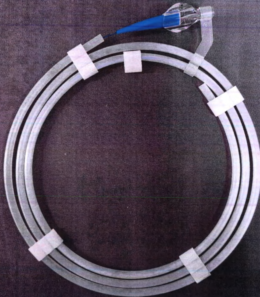
Рис. 15. Катетер дилатационный баллонный Mozec PTA Rx 0.014" для чрескожной транслюминальной ангиопластики (ЧТА), эффективная длина 150 см, диаметр x длина баллона 2,50 x 120 мм.
