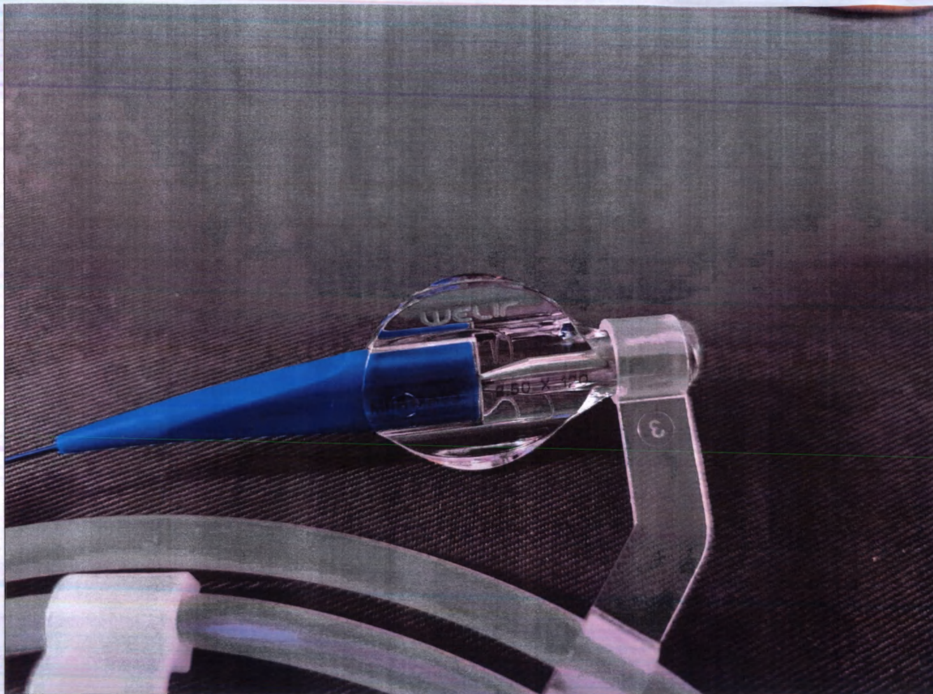
Рис. 16. Катетер дилатационный баллонный Mozec PTA Rx 0.014" для чрескожной транслюминальной ангиопластики (ЧТА), эффективная длина 150 см, диаметр x длина баллона 2,50 x 120 мм.
