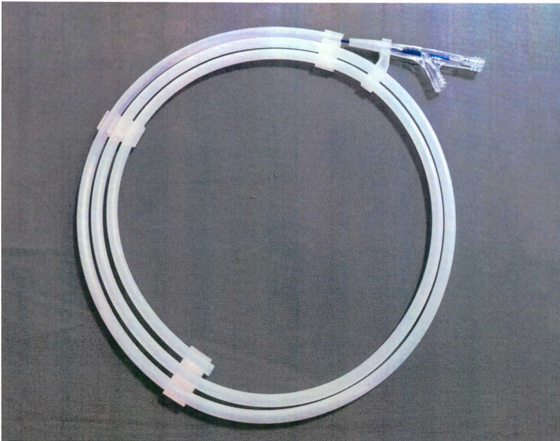
Рис. 12. Катетер баллонный дилатационный ПТА Shunmei для чрескожной транслюминальной ангиопластики Shun Sofer, размер баллона 7,0 x 200 мм, эффективная длина 40 см
