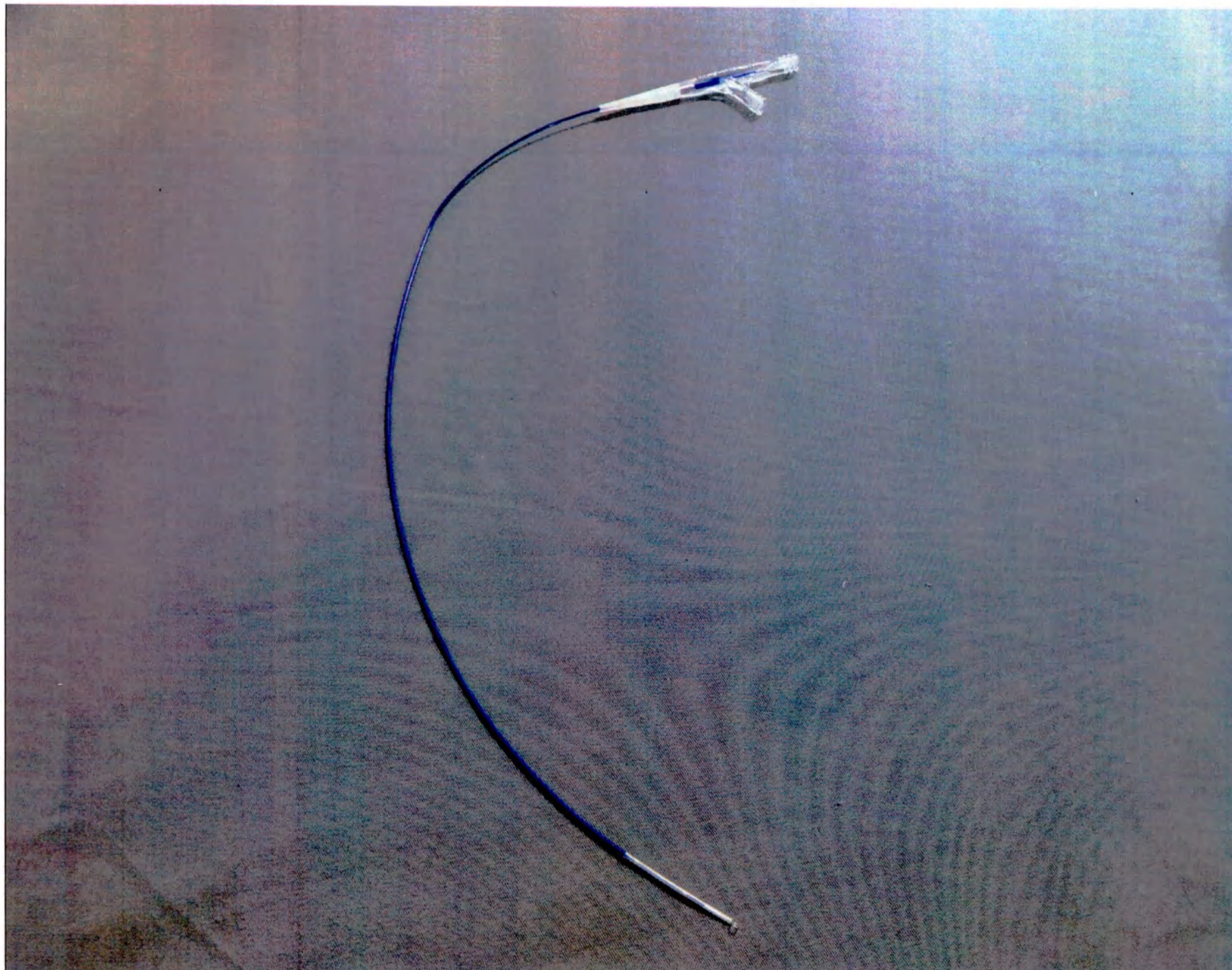
Рис. 4. Катетер баллонный дилатационный РТА Shunmei для чрескожной транслюминальной ангиопластики Shun Sofer, размер баллона 2,0 x 20 мм, эффективная длина 40 см
