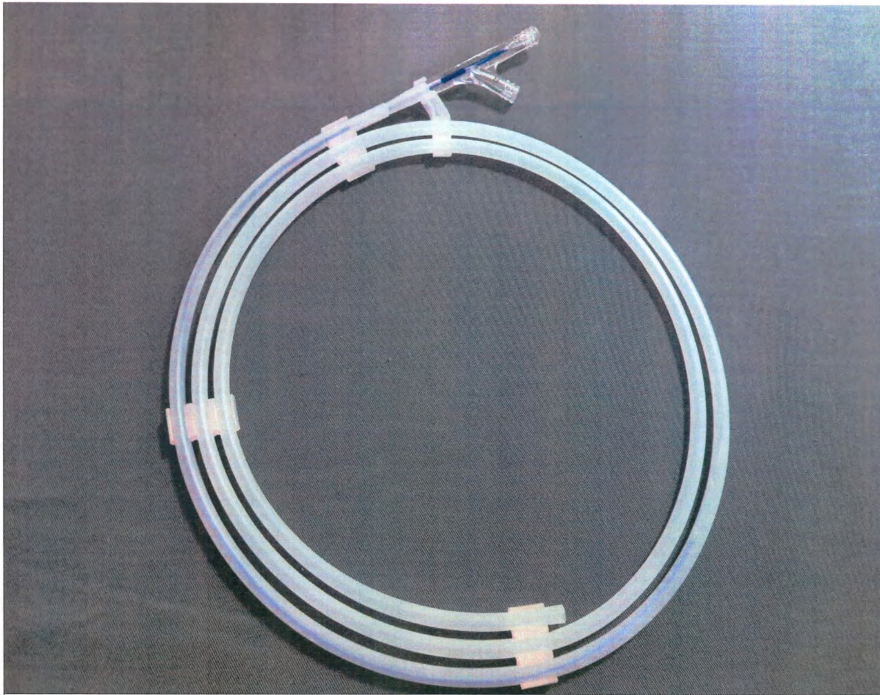
Рис. 3. Катетер баллонный дилатационный ПТА Shunmei для чрескожной транслюминальной ангиопластики Shun Sofer, размер баллона 2,0 x 20 мм, эффективная длина 40 см
