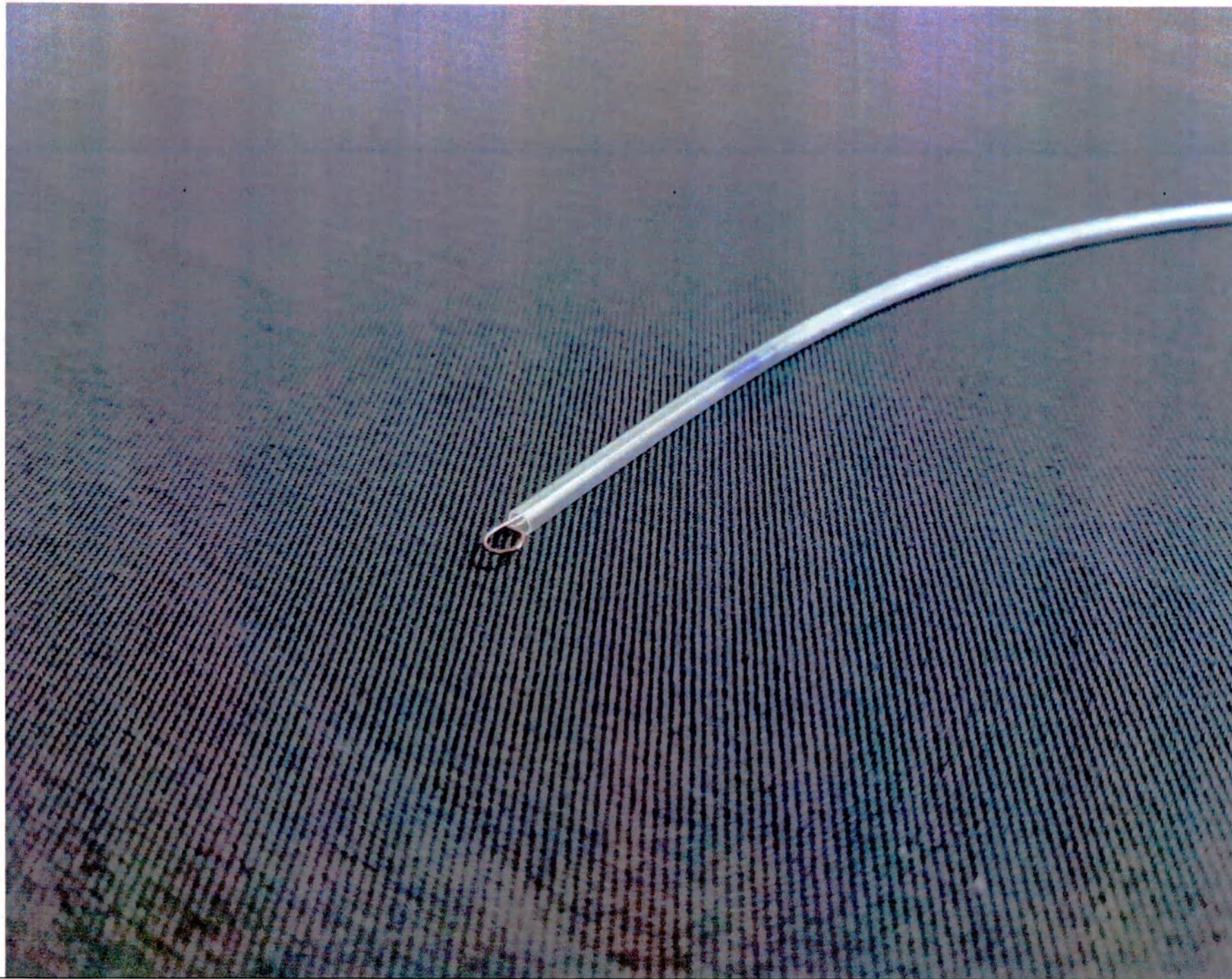
Рис. 13. Катетер баллонный дилатационный РТА Shunmei для чрескожной транслюминальной ангиопластики Shun Sofer, размер баллона 7,0 x 200 мм, эффективная длина 40 см
