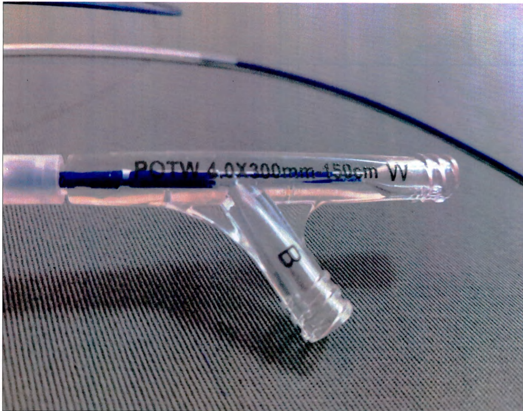
Рис. 10. Катетер баллонный дилатационный ПТА Shunmei для чрескожной транслюминальной ангиопластики Shun Sofer, размер баллона 4,0 x 300 мм, эффективная длина 150 см
