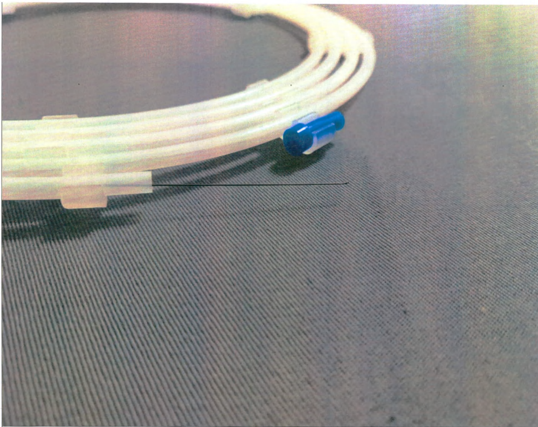
Рис. 12. Спираль отсоединяемая Shunmei на системе доставки (толкатель, длина 190 см) для эмболизации кровеносных сосудов, серия 14, диаметр x длина спирали: 2 x 20 мм
