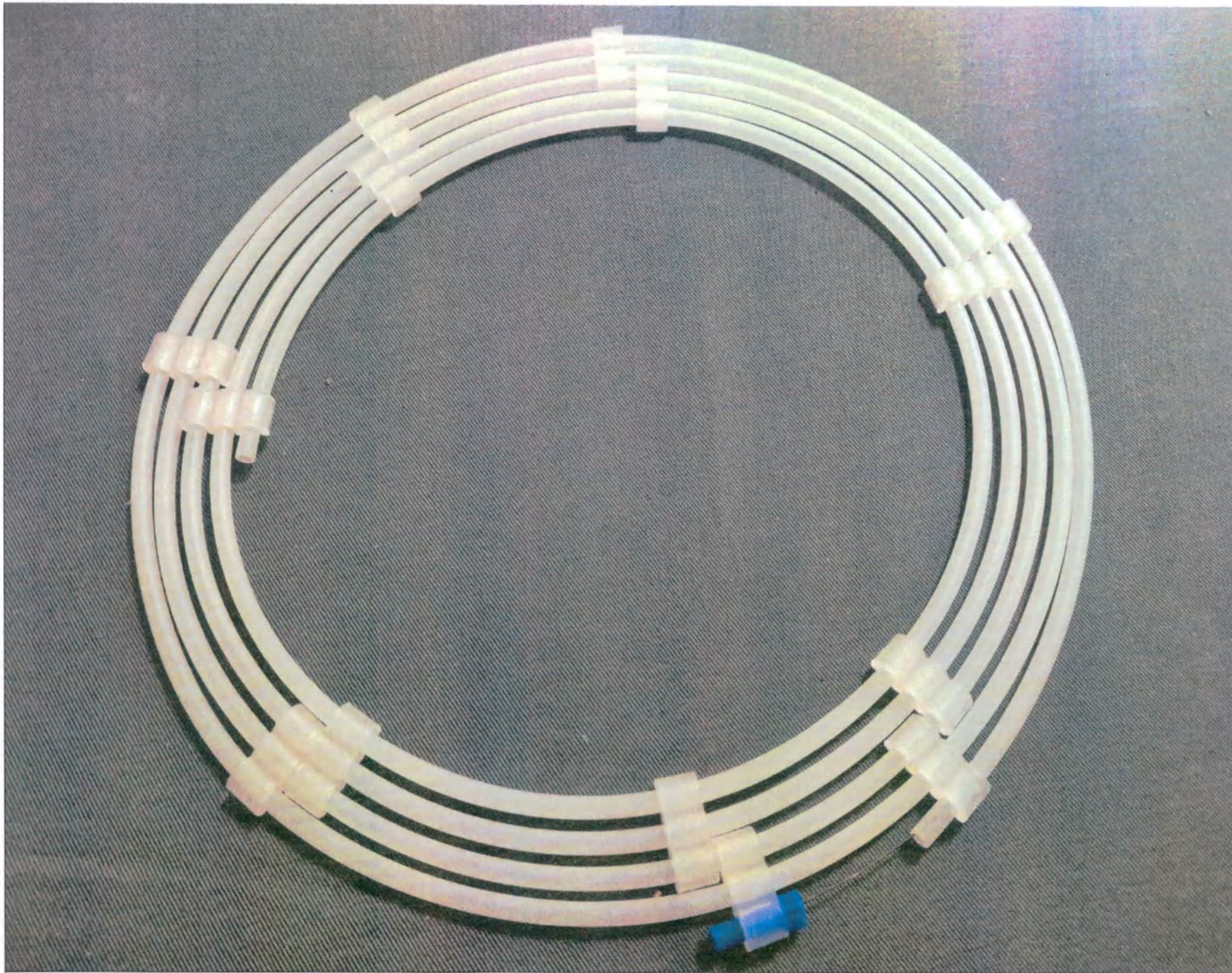
Рис. 6. Спираль отсоединяемая Shunmei на системе доставки (толкатель, длина 190 см) для эмболизации кровеносных сосудов, серия 10, диаметр x длина спирали: 20 x 500 мм
