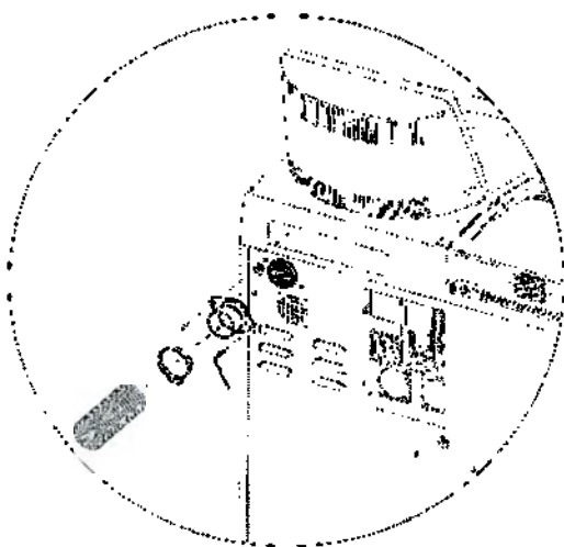
Установка адаптера вытяжной вентиляции
