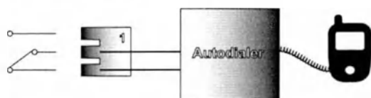
Подключение устройства автодозвона к разъему "Сигнализация 1"
