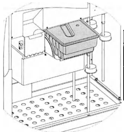
Лоток для использованного парафина, установленный над П1 и П2
