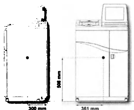
Положение центра тяжести (средняя загрузка реагентами)
