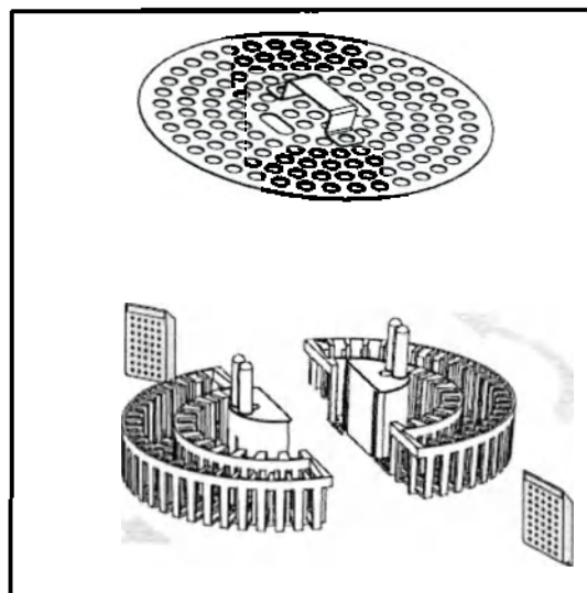
Загрузка кассет в секционную корзину
