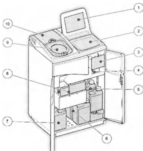
Excelsior AS (вид спереди, двери открыты)
