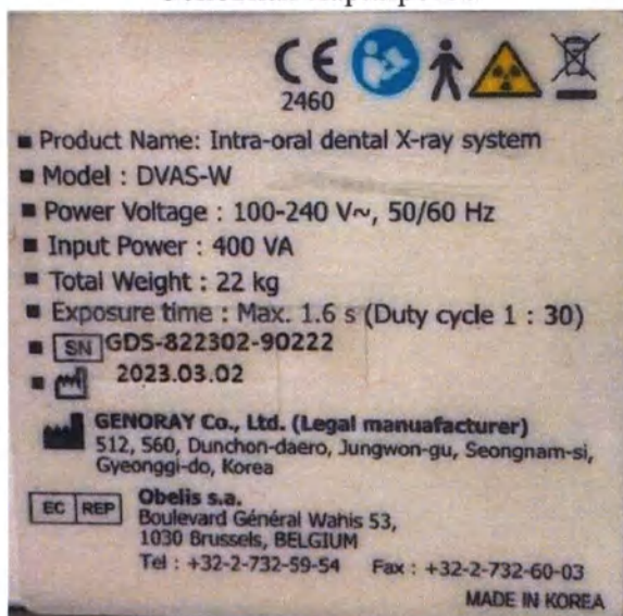
Основная маркировка
