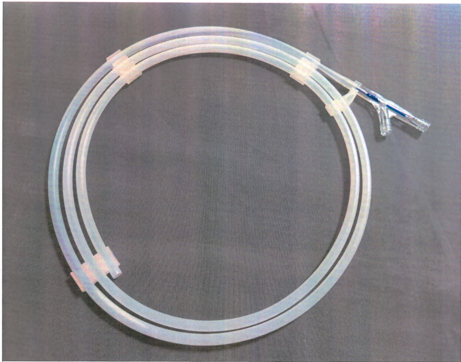
Рис. 14. Катетер баллонный дилатационный с лекарственным покрытием Shunmei для чрескожной транслуминальной ангиопластики периферических сосудов Shun Ocean, размер баллона (диаметр x длина) 7 мм × 20 мм, эффективная длина 40 см
