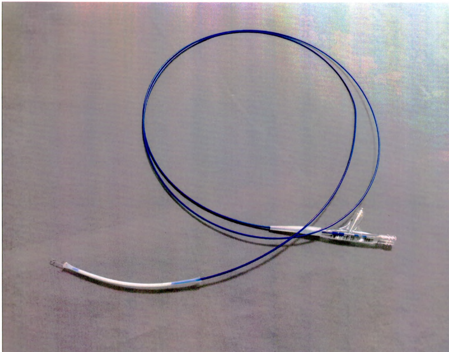
Рис. 10. Катетер баллонный дилатационный с лекарственным покрытием Shunmei для чрескожной транслюминальной ангиопластики периферических сосудов Shun Ocean, размер баллона (диаметр x длина) 5 мм × 60 мм, эффективная длина 150 см
