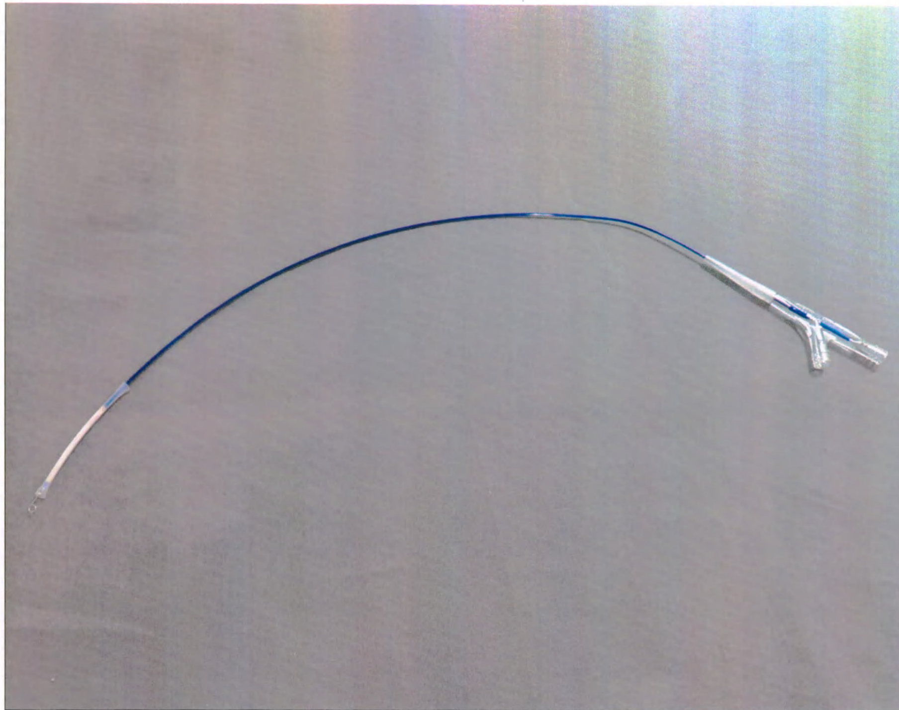
Рис. 15. Катетер баллонный дилатационный с лекарственным покрытием Shunmei для чрескожной транслуминальной ангиопластики периферических сосудов Shun Ocean, размер баллона (диаметр x длина) 7 мм × 20 мм, эффективная длина 40 см
