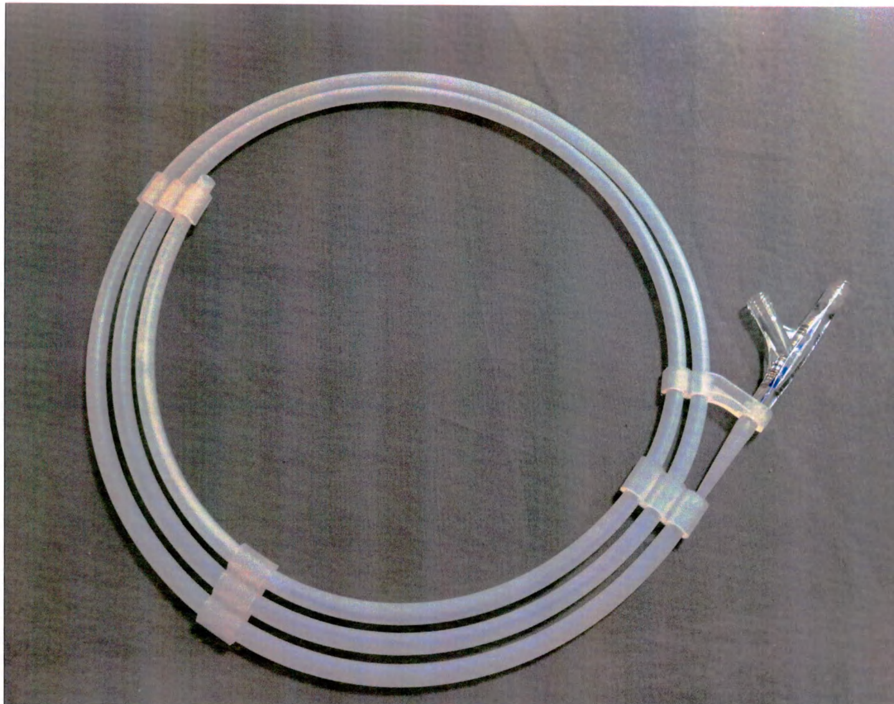
Рис. 8. Катетер баллонный дилатационный с лекарственным покрытием Shunmei для чрескожной транслуминальной ангиопластики периферических сосудов Shun Ocean, размер баллона (диаметр x длина) 5 мм × 60 мм, эффективная длина 150 см
