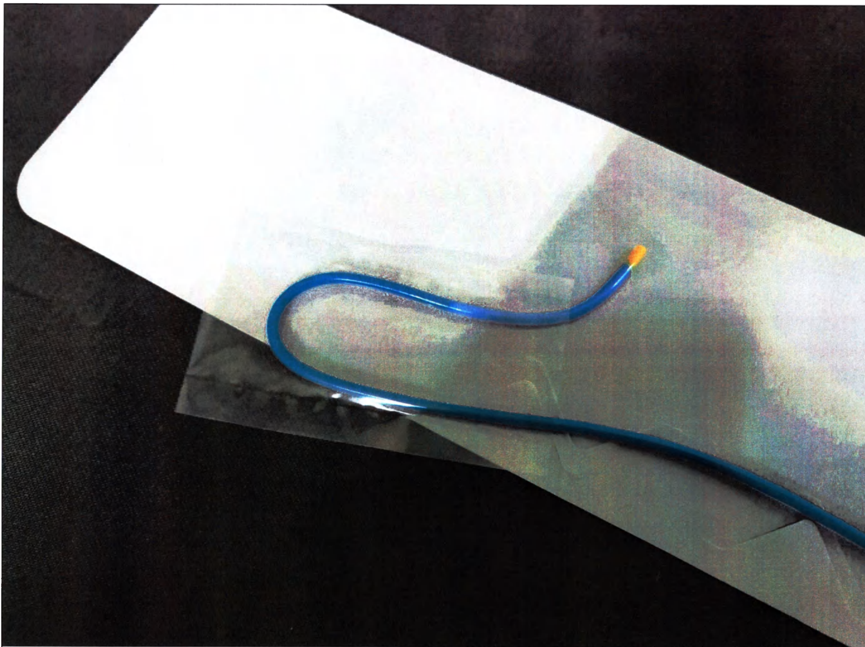
Рис. 36. Катетер внутрисосудистый диагностический CONVEYOR, SIM2, диаметр 6F, длина 100 см
