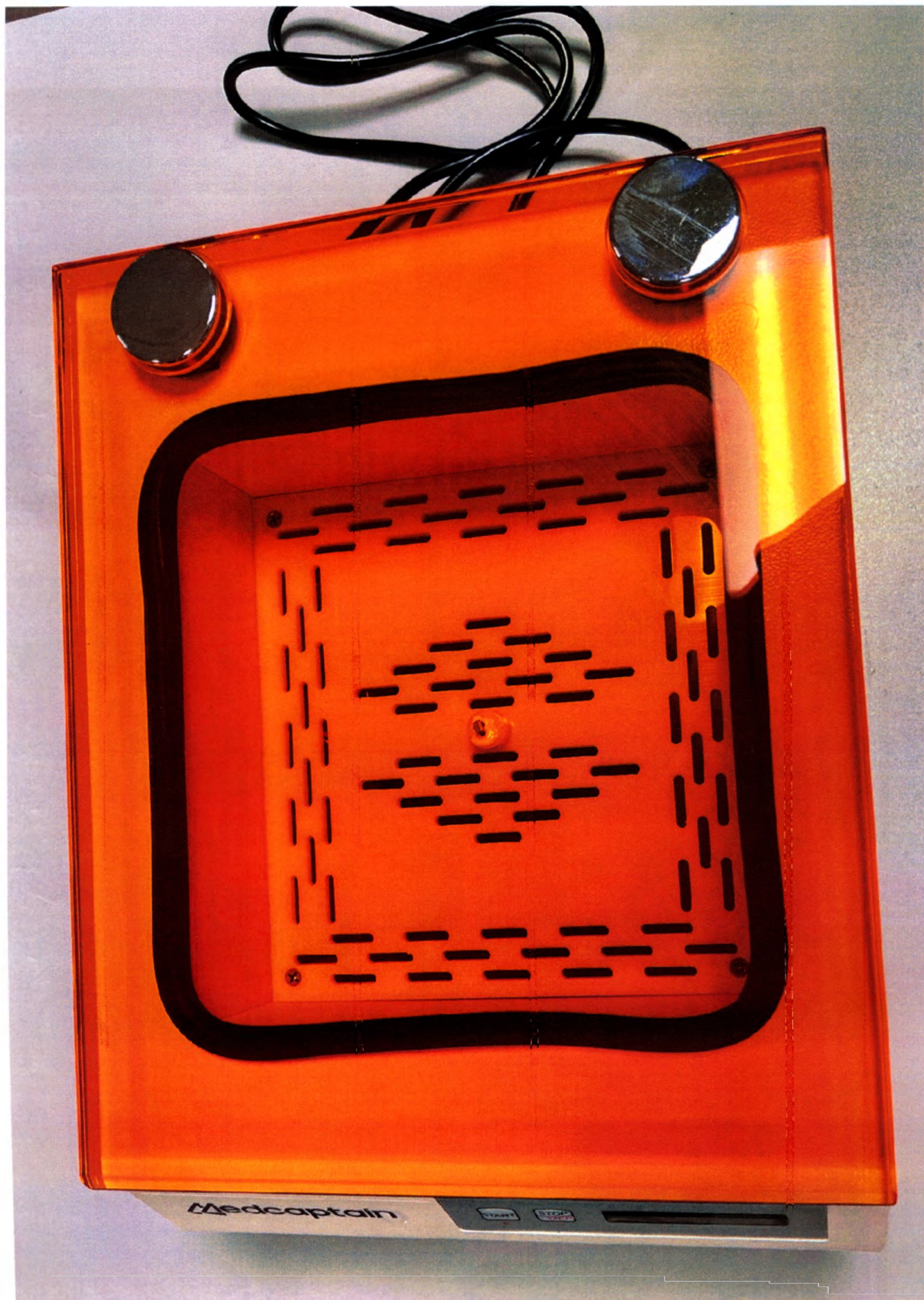
Вид сверху Инкубатор FYQ из МИ «Инкубатор FYQ для карт гелевых для иммуногематологических исследований методом колоночной агглютинации для диагностики in vitro»
