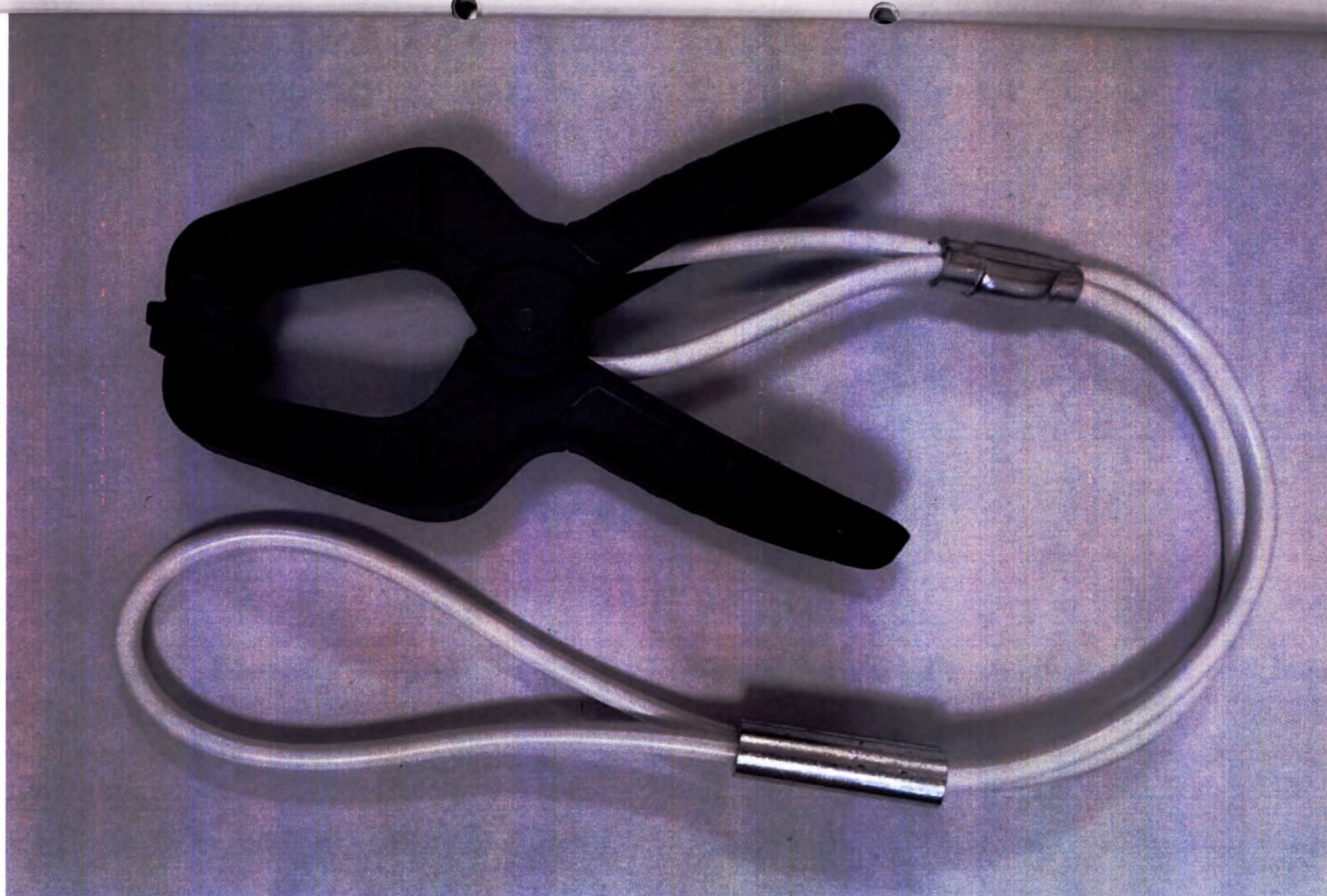
Общий вид зажима для воздуховода (YC010100001)
