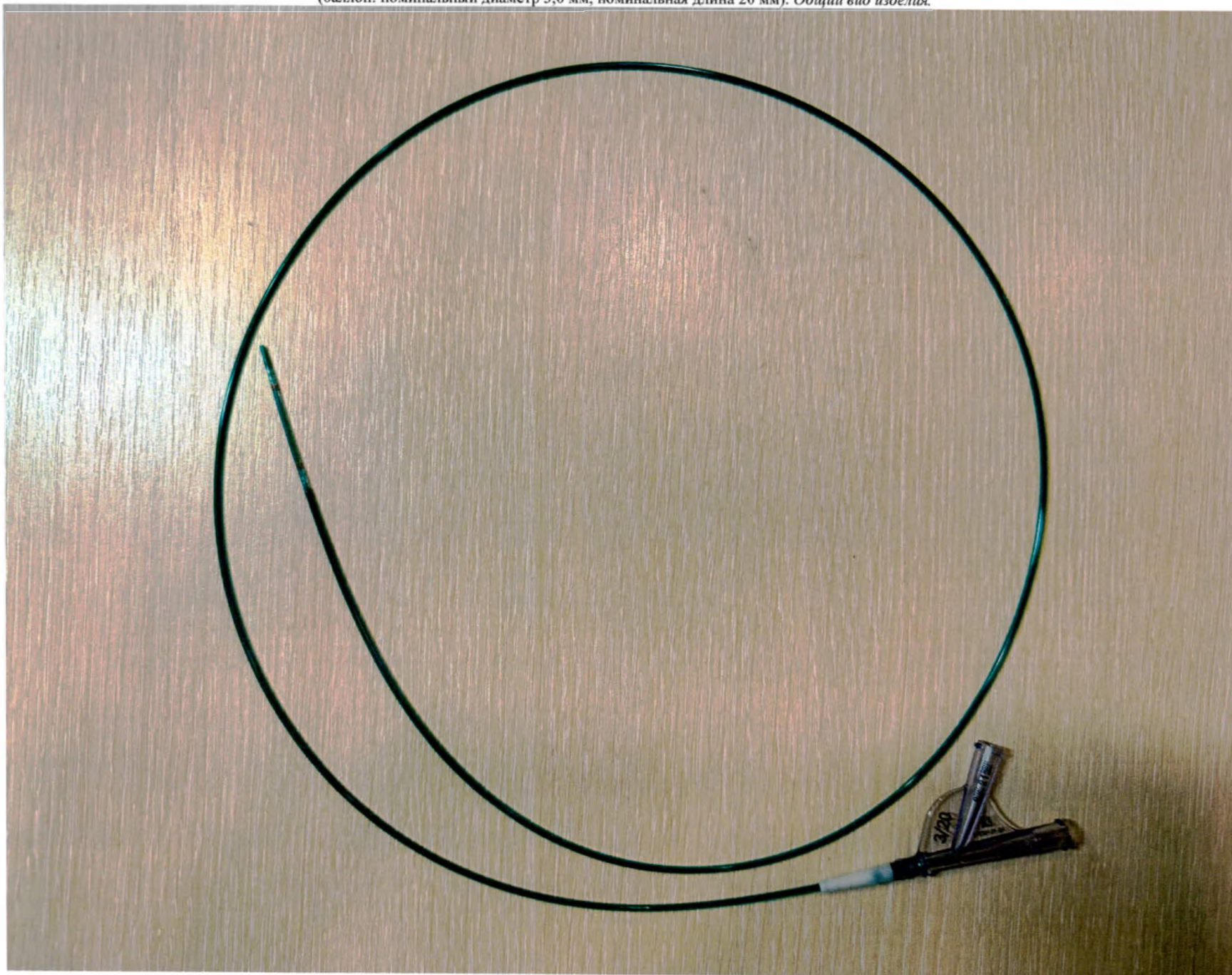
Катетер периферический расширяющий Passeo-35 Xeo рабочей длиной 90 см (баллон: номинальный диаметр 3,0 мм, номинальная длина 20 мм). Общий вид изделия.
