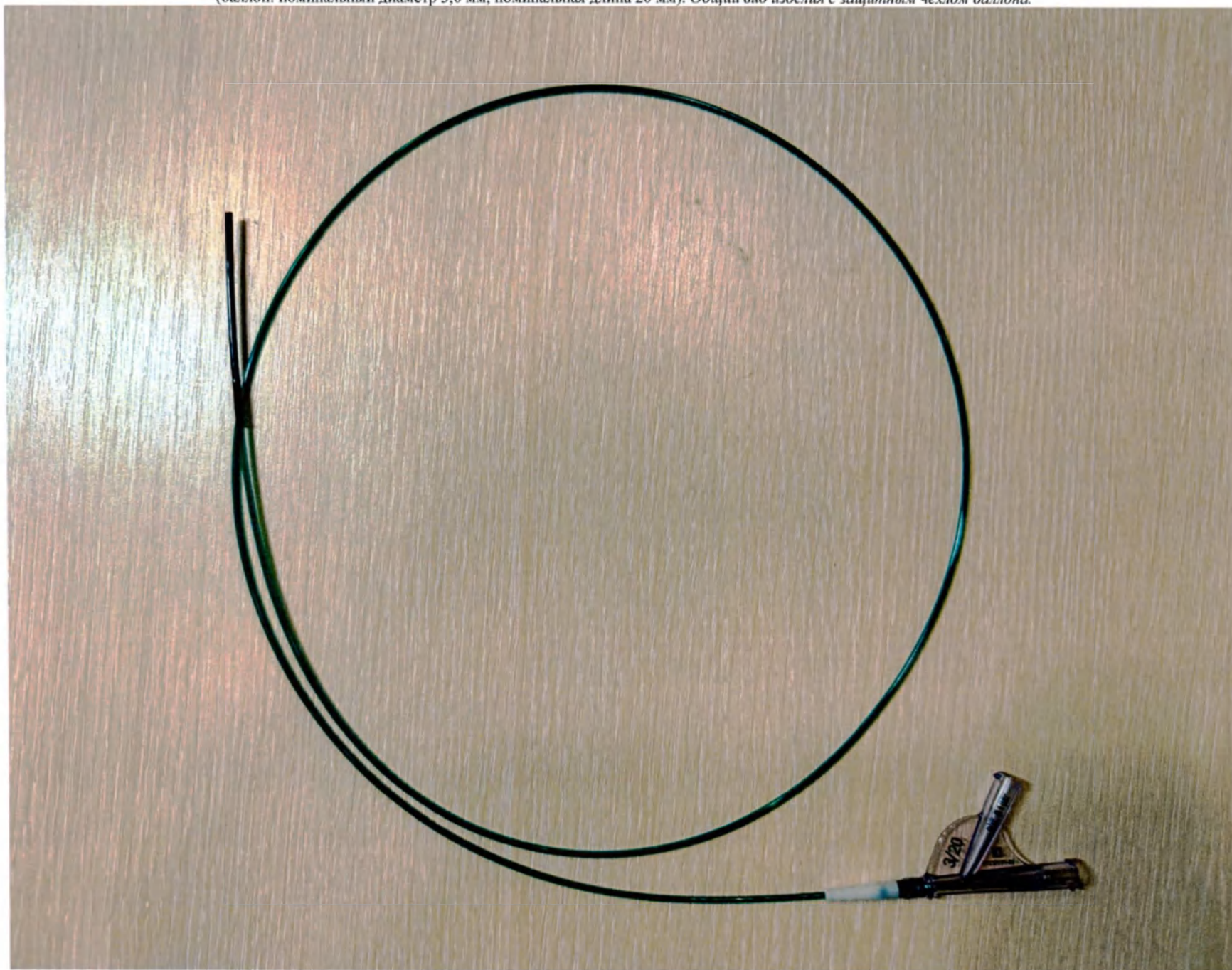
Катетер периферический расширяющий Passeo-35 Хео рабочей длиной 90 см (баллон: номинальный диаметр 3,0 мм, номинальная длина 20 мм). Общий вид изделия с защитным чехлом баллона.
