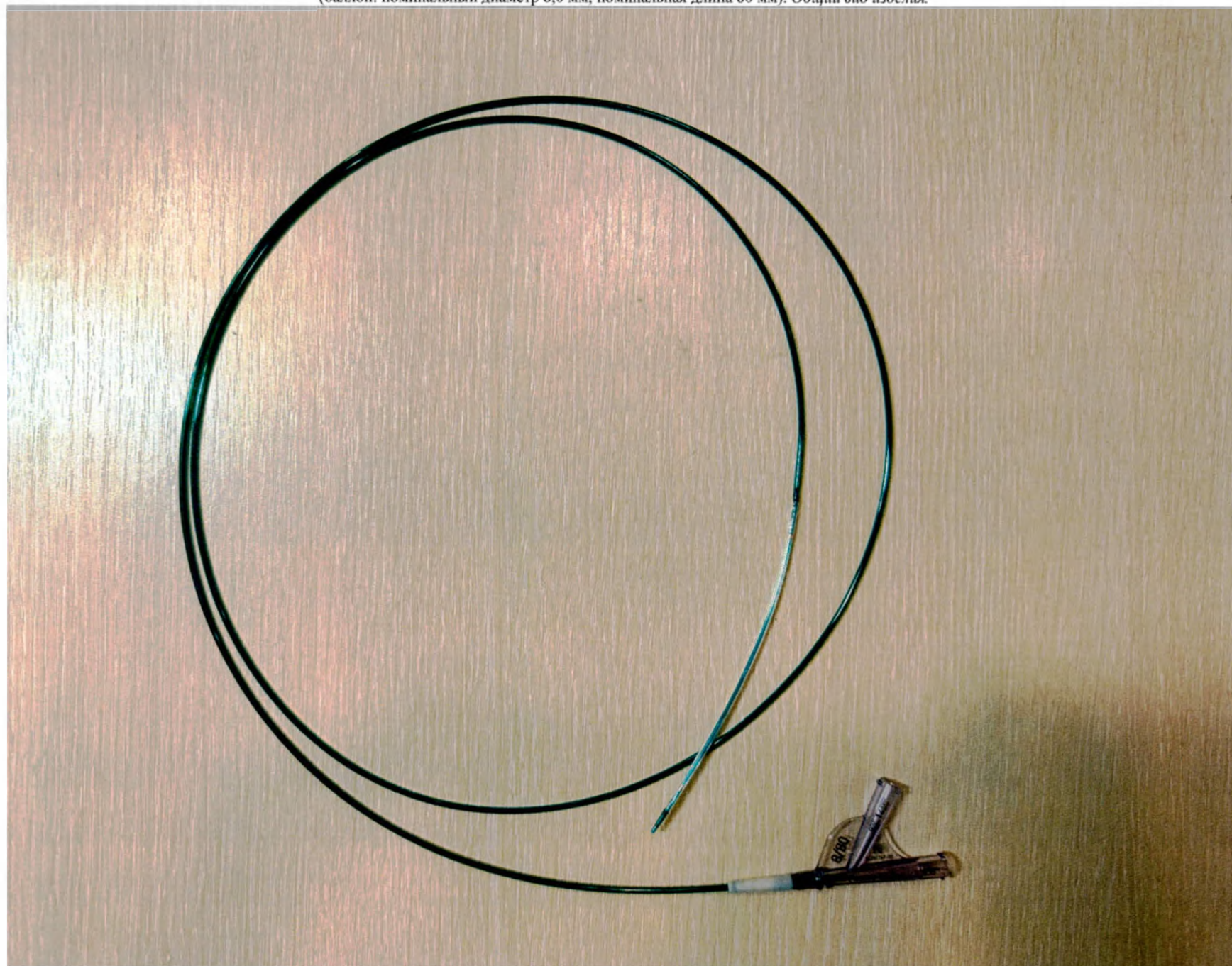
Катетер периферический расширяющий Passeo-35 Хео рабочей длиной 130 см (баллон: номинальный диаметр 8,0 мм, номинальная длина 80 мм). Общий вид изделия.
