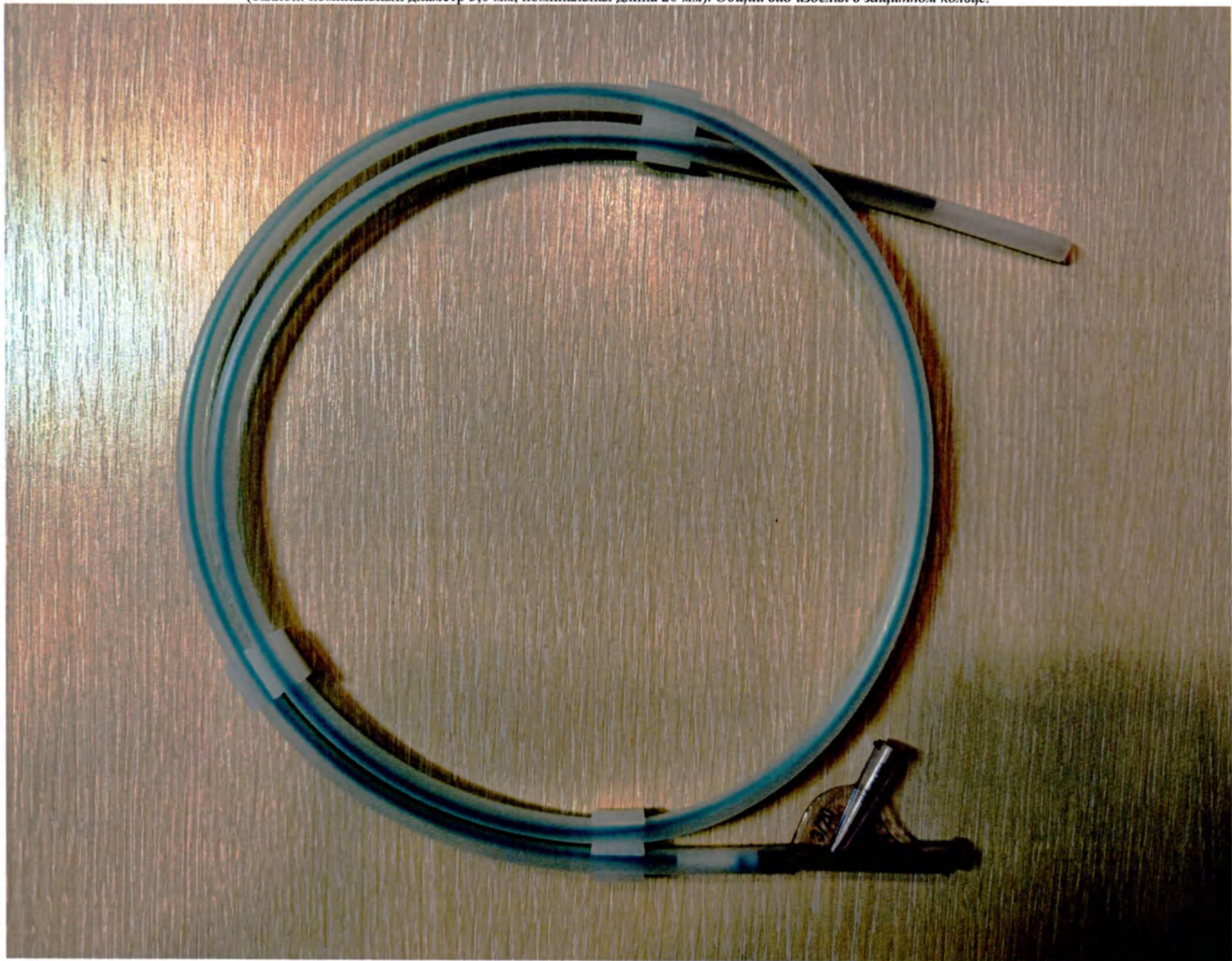
Катетер периферический расширяющий Passeo-35 Хео рабочей длиной 90 см (баллон: номинальный диаметр 3,0 мм, номинальная длина 20 мм). Общий вид изделия в защитном кольце.
