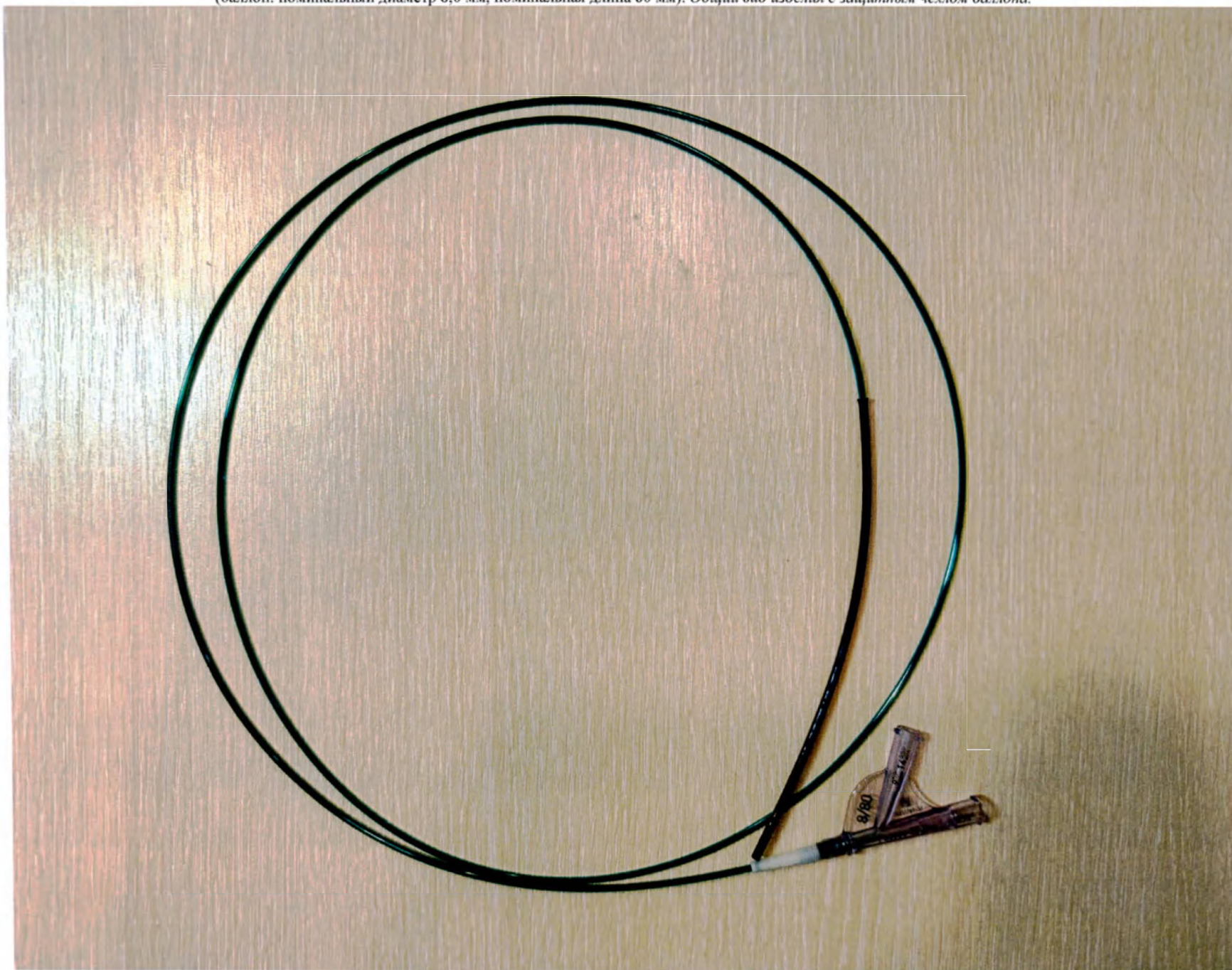
Катетер периферический расширяющий Passeo-35 Хео рабочей длиной 130 см (баллон: номинальный диаметр 8,0 мм, номинальная длина 80 мм). Общий вид изделия с защитным чехлом баллона.
