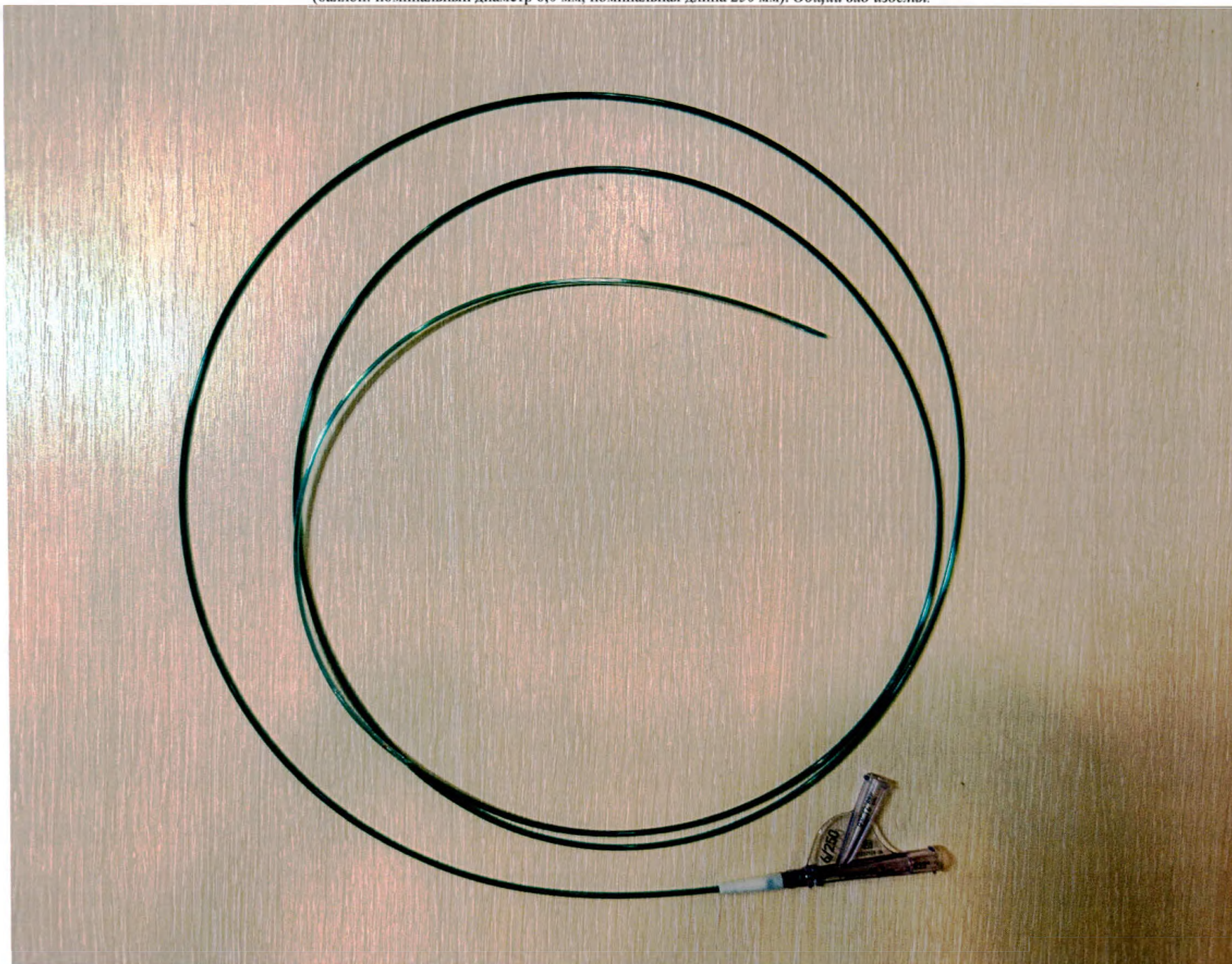
Катетер периферический расширяющий Passeo-35 Xeo рабочей длиной 170 см (баллон: номинальный диаметр 6,0 мм, номинальная длина 250 мм). Общий вид изделия.
