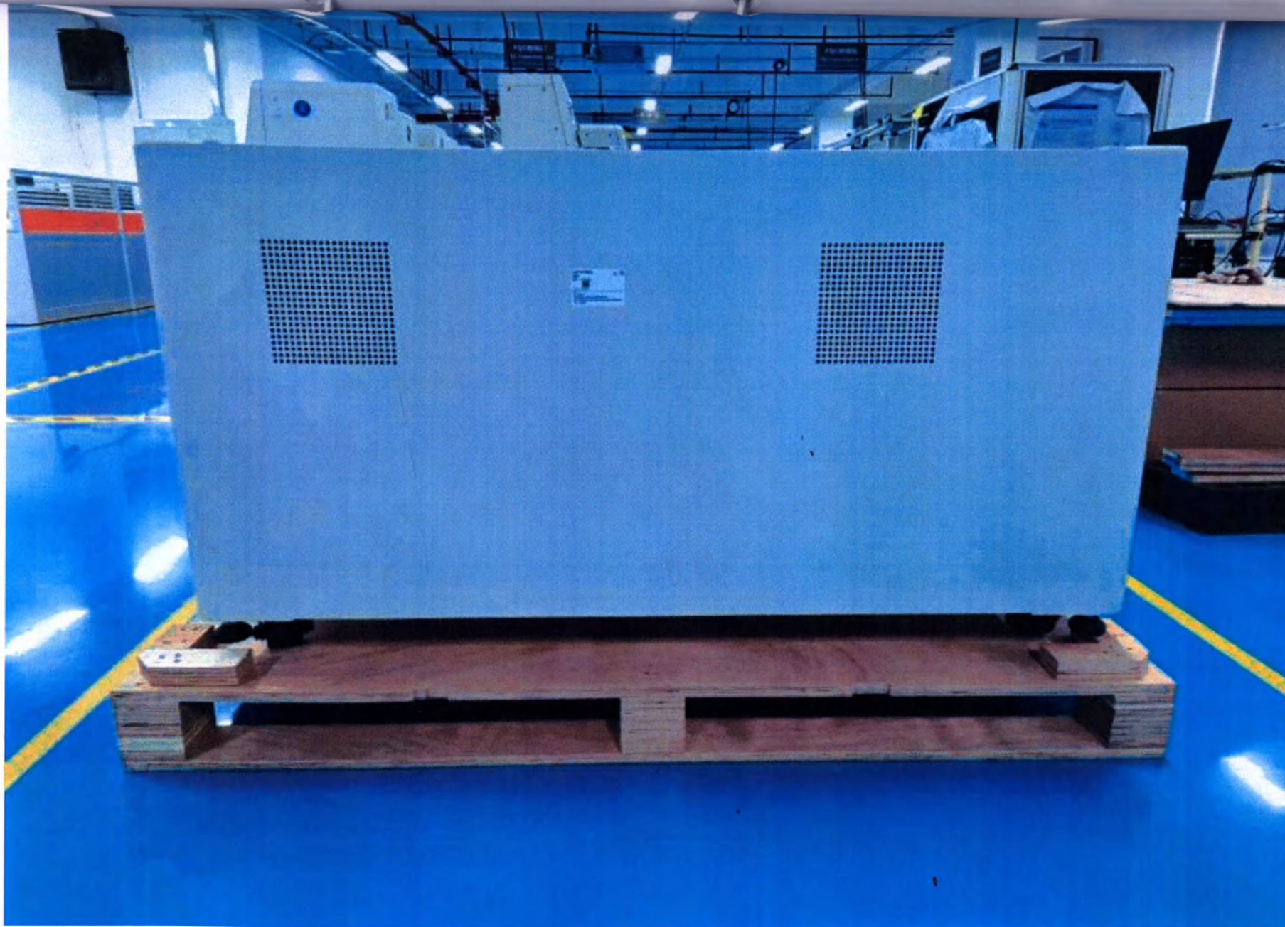
Шкаф для анализатора (вид сзади)
