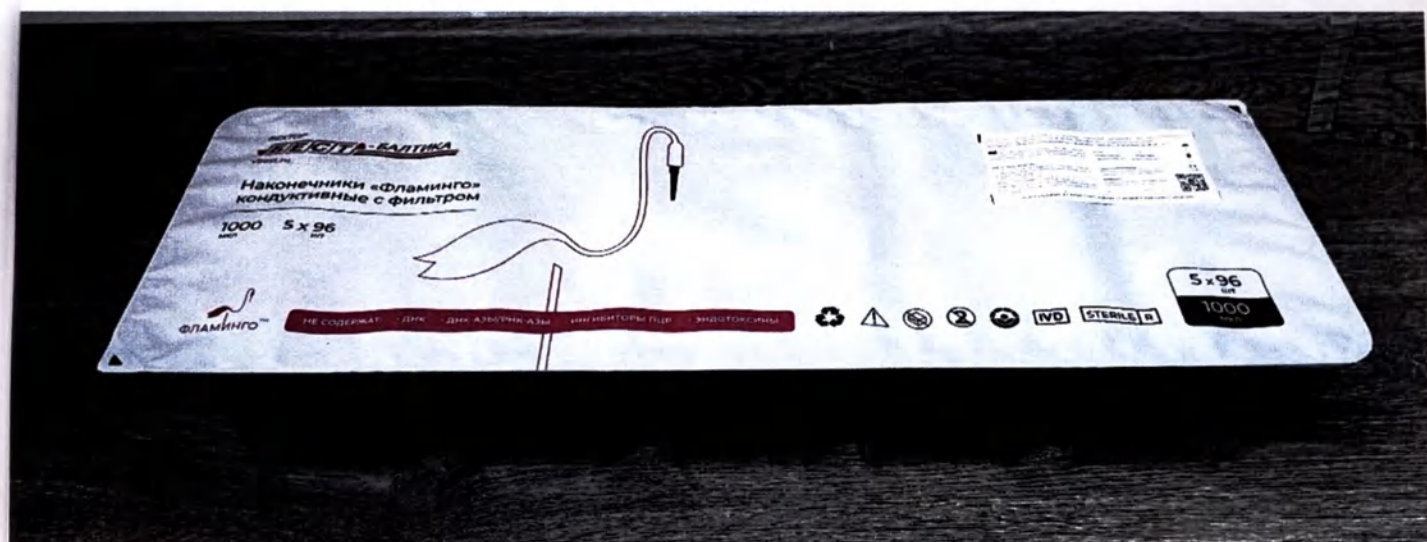
Рисунок 14 – Наконечники «Фламинго» кондуктивные с фильтром, 1000 мкл, 5 штативов по 96 шт./уп.
