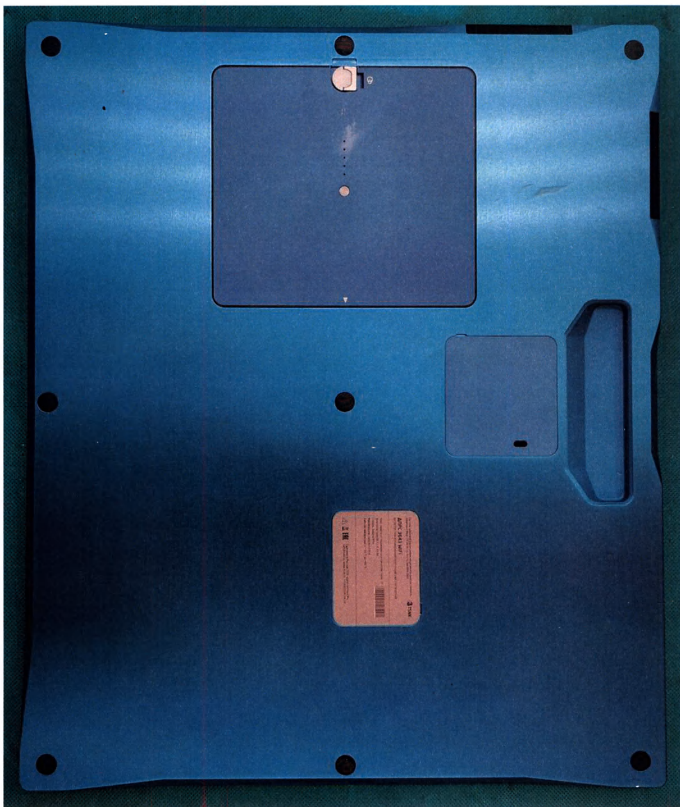
Аппарат медицинский рентгенодиагностический переносной «МИРАН» по ТУ 26.60.11-003-17942806-2022 артикул Б: детектор рентгеновский ДПРС 3643 WiFi
