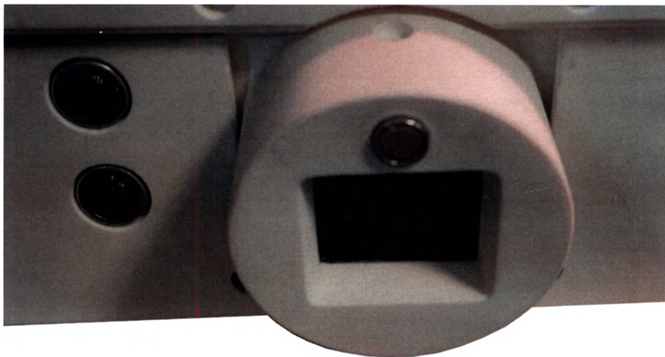
Аппарат медицинский рентгенодиагностический переносной «МИРАН» по ТУ 26.60.11-003-17942806-2022 артикул Б: коллиматор
