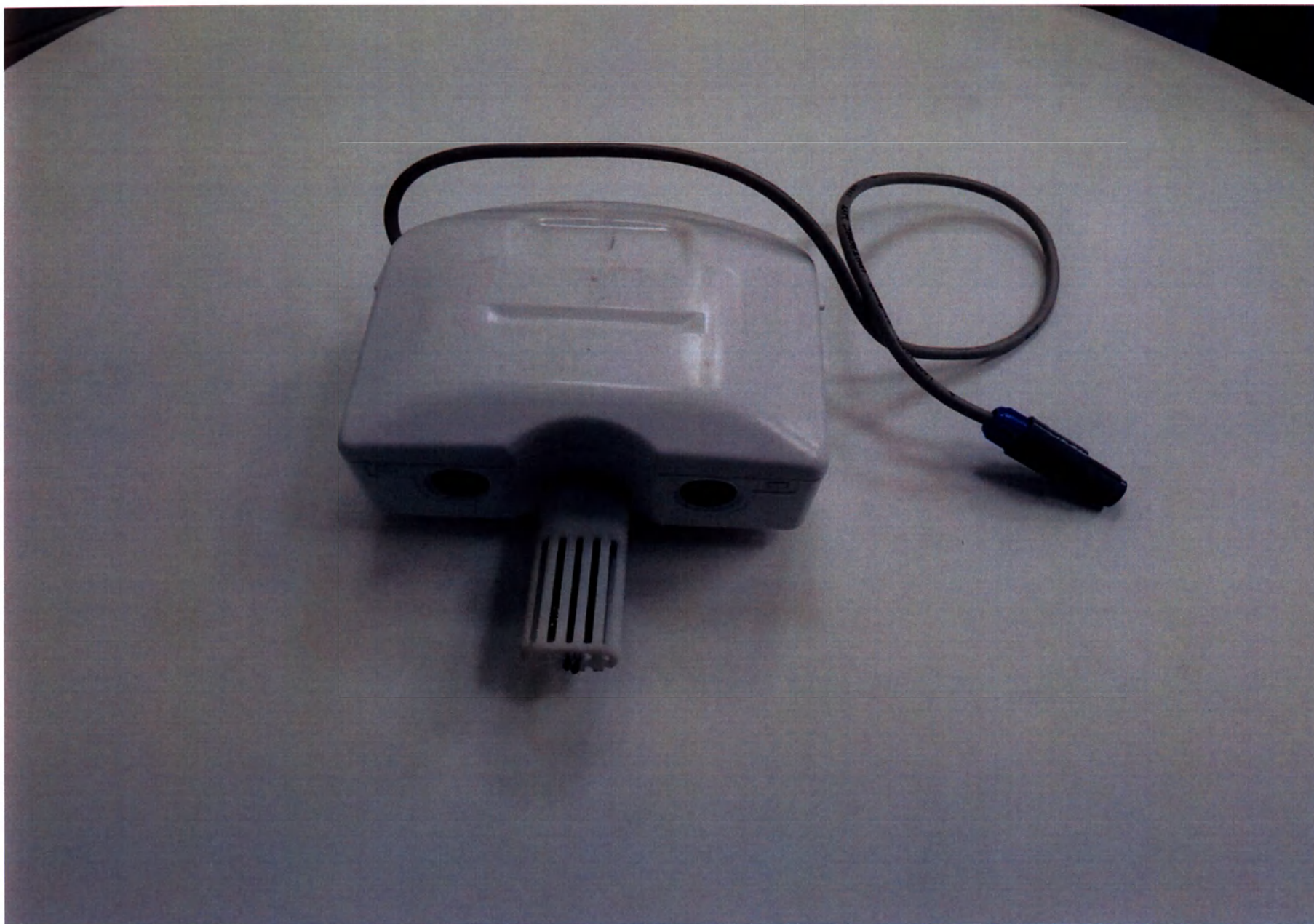
(INC200-003) Блок датчиков
