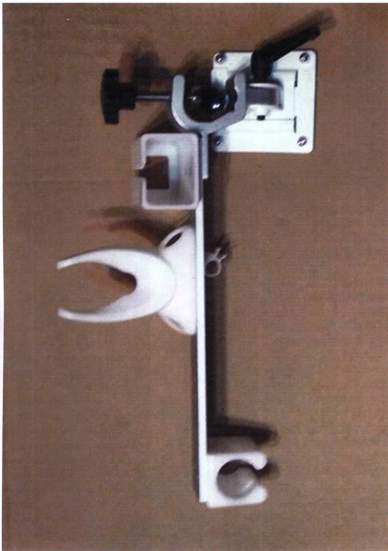
Кронштейн Рulon
