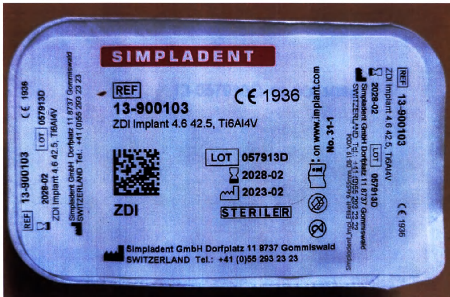
Индивидуальная упаковка Имплантата одноэтапного Simpladent на примере варианта исполнения Имплантат одноэтапный ZDI
