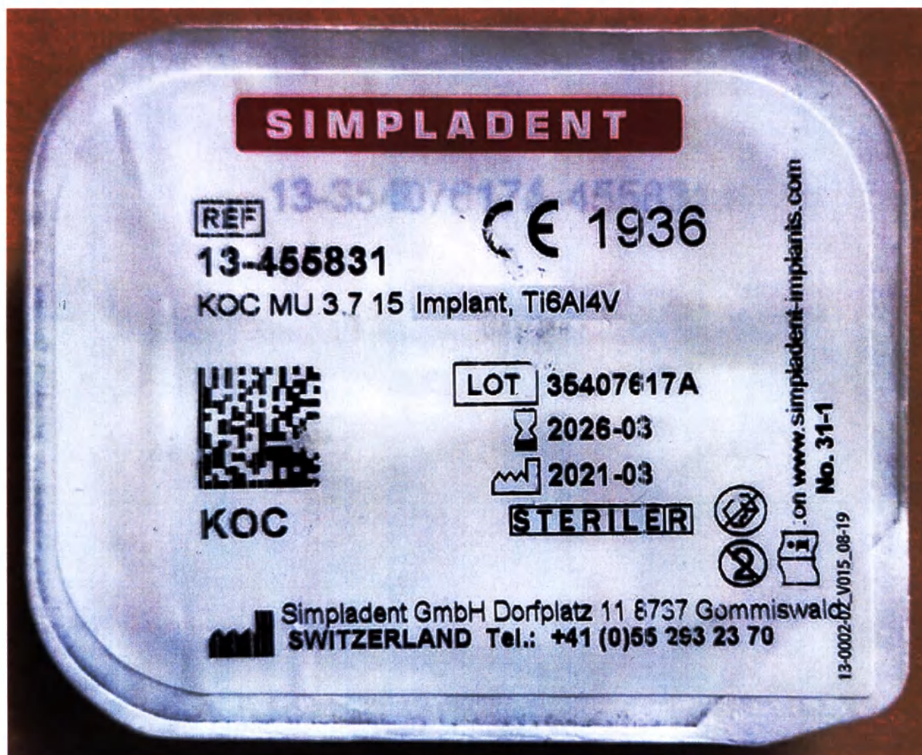
Индивидуальная упаковка Имплантата одноэтапного Simpladent на примере варианта исполнения Имплантат одноэтапный KOC MU
