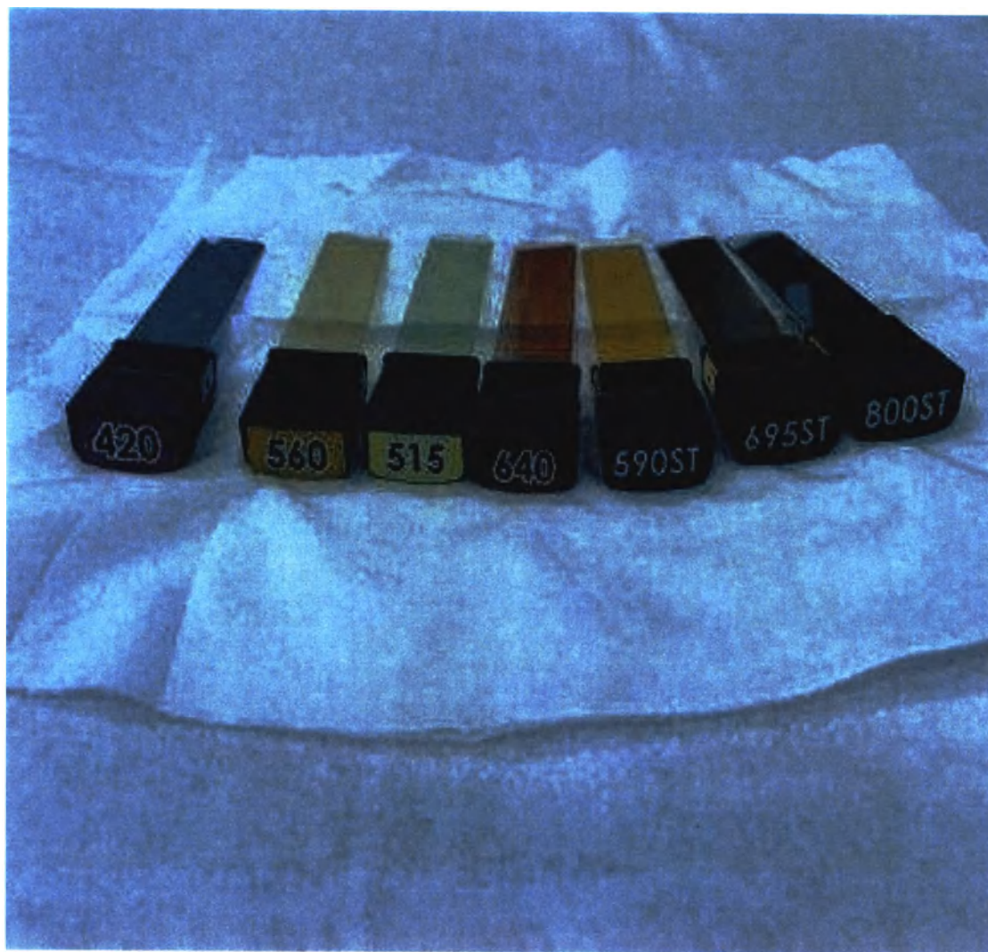
Фильтр 420 нм, фильтр 515 нм, фильтр 560 нм, фильтр 640 нм, фильтр 590 нм ST, фильтр 695 нм ST, фильтр 800 нм ST
