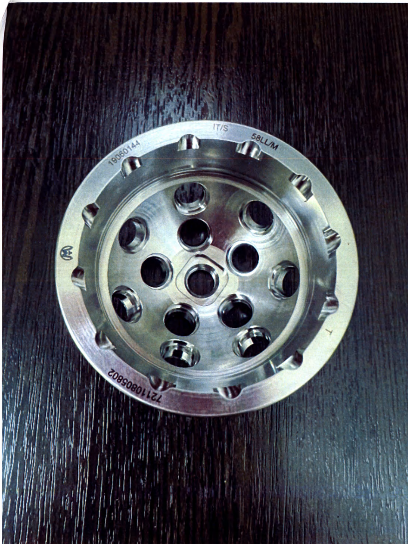
Рисунок 4. Вид снизу Компонента вертлужного (чашки) Ti Plasma многодырчатого, размер 58LL/M – 1 шт.
