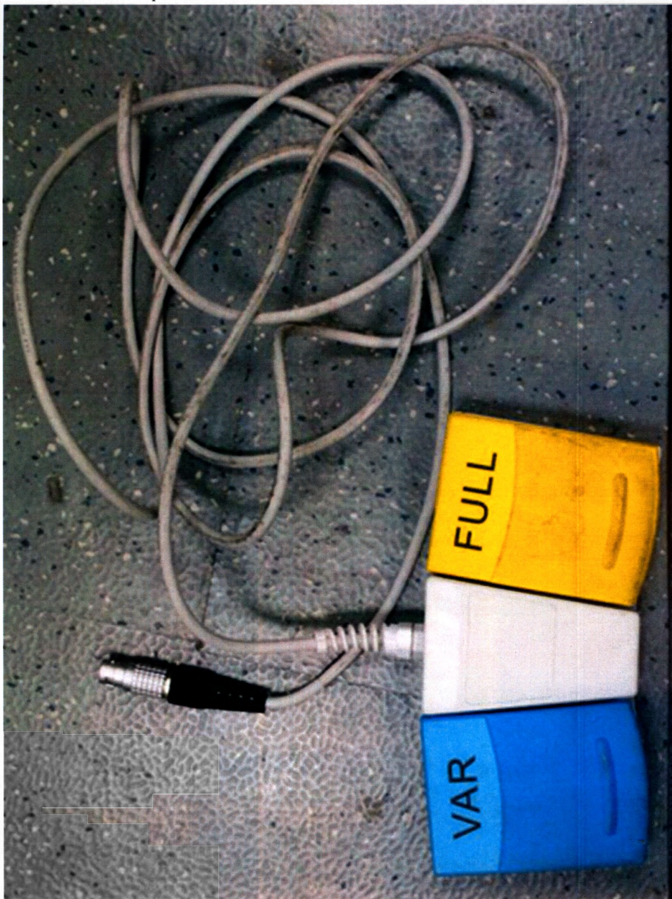
2. Ножной переключатель модели FSW2 с кабелем. Общий вид.
