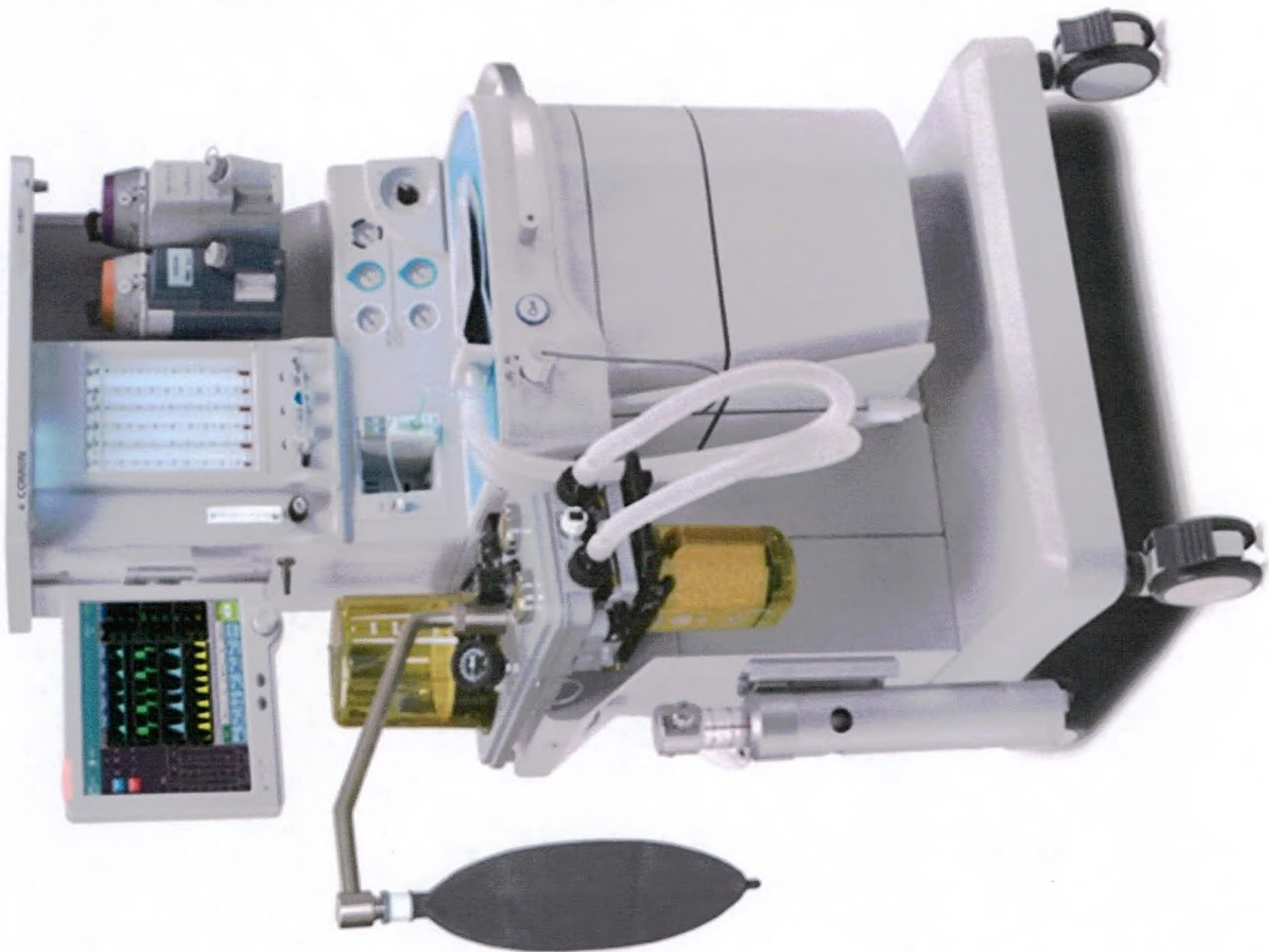
Аппарат наркозно-дыхательный серии АХ, вариант исполнения. АХ-600, основной блок (в сборе)
