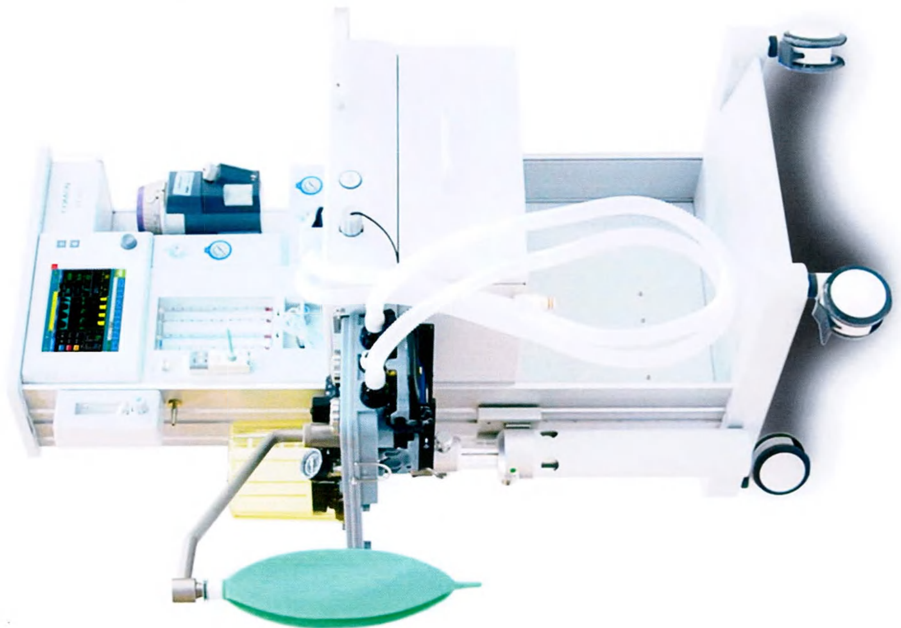
Аппарат наркозно-дыхательный серии АХ, вариант исполнения. АХ-400, АХ-400А, основной блок (в сборе)
