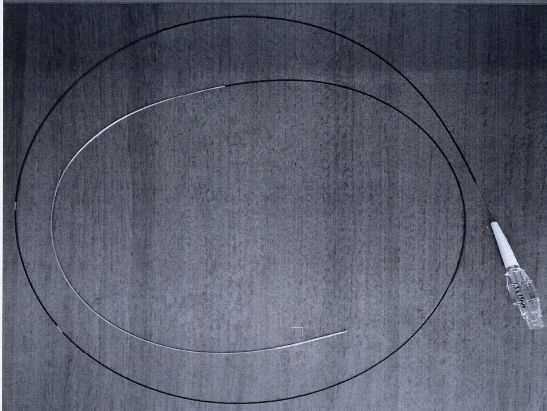
Рис.5. Фотографическое изображение МИ: «Катетер баллонный дилатационный для коронарной ангиопластики, варианты исполнения: Fast Track. Катетер Fast Track VM-FTII. Изображение МИ без упаковки.
