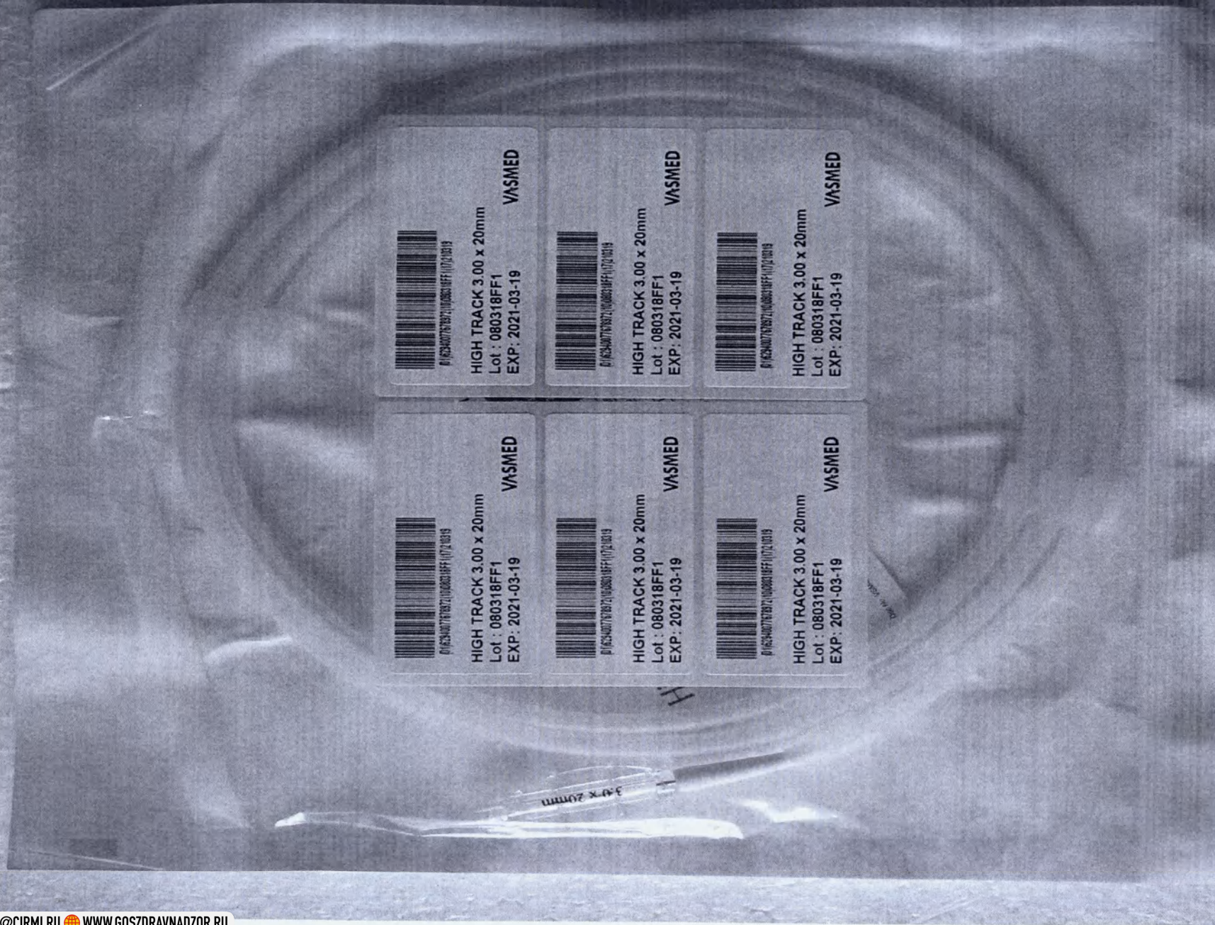
Рис.21. Фотографическое изображение МИ: «Катетер баллонный для коронарной ангиопластики, варианты исполнения: High Track. Катетер High VM-HT-300-20, размер баллона: 3,00 мм x 20 мм. Изображение блистерной упаковки (лицевая сторона)
