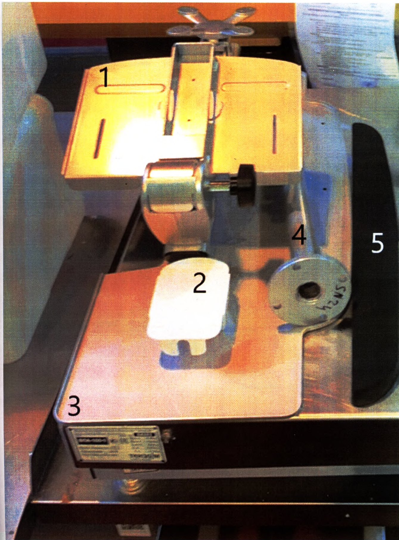
Монтажное место для монитора и клавиатуры (1 - Подставка для монитора; 2 - Панель кронштейна; 3 - Подставка под клавиатуру; 4 – Держатель; 5 - Стопор пластиковый)
