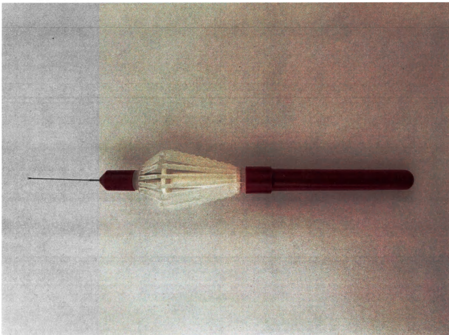
Рисунок 26 – Ножницы офтальмологические одноразовые Vitreo Line в варианте исполнения Vitreo Line SS-27
