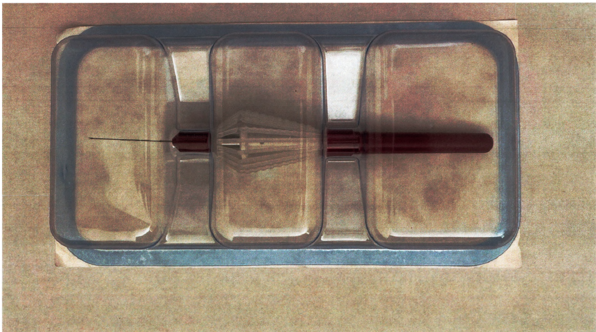
Рисунок 24 – Ножницы офтальмологические одноразовые Vitreo Line в варианте исполнения Vitreo Line SS-27 в индивидуальной упаковке
