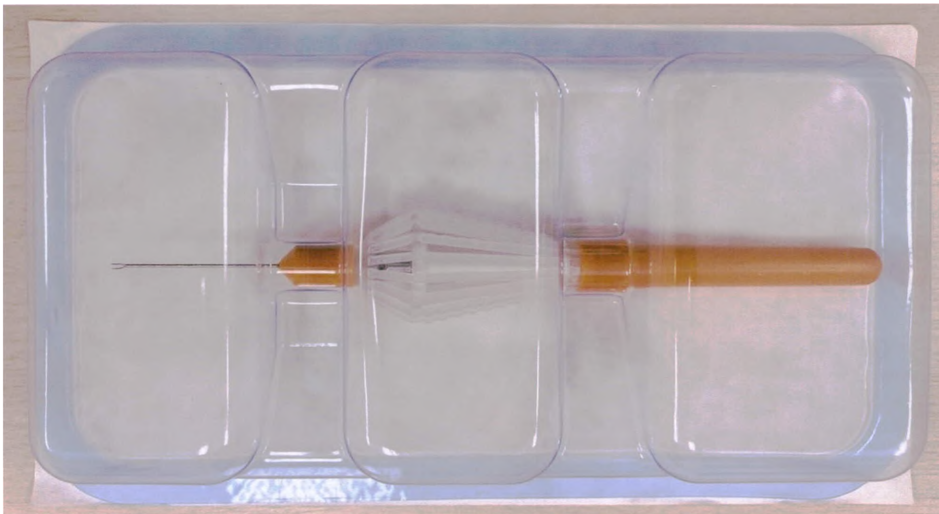
Рисунок 33 – Пинцет офтальмологический стерильный одноразового использования Vitreo Line FJ-23 в индивидуальной упаковке
