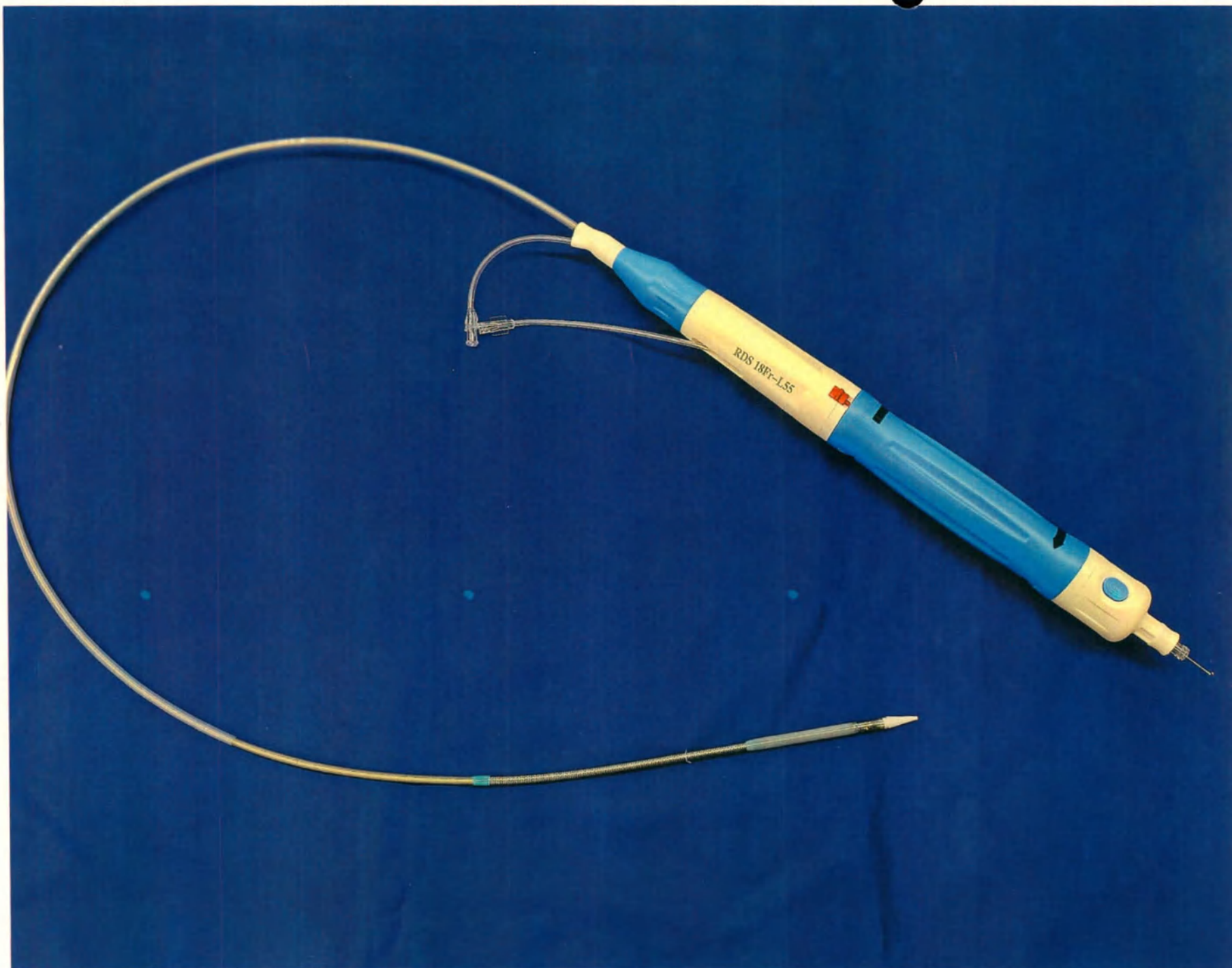
Фотография 2 – Общий вид Системы доставки для имплантации аортального клапана VenusA-Pro™, модель: RDS 18Fr-L55
