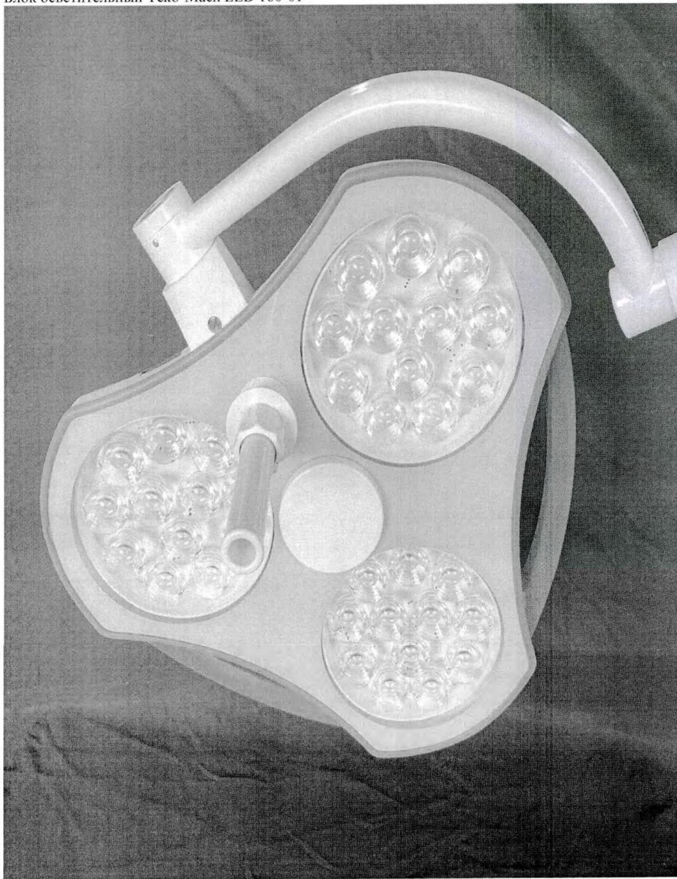
Блок осветительный Teko-Mach LED 160-01
