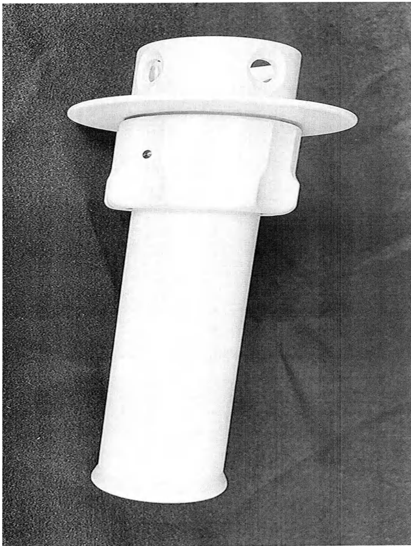
Рукоятка стерилизуемая
