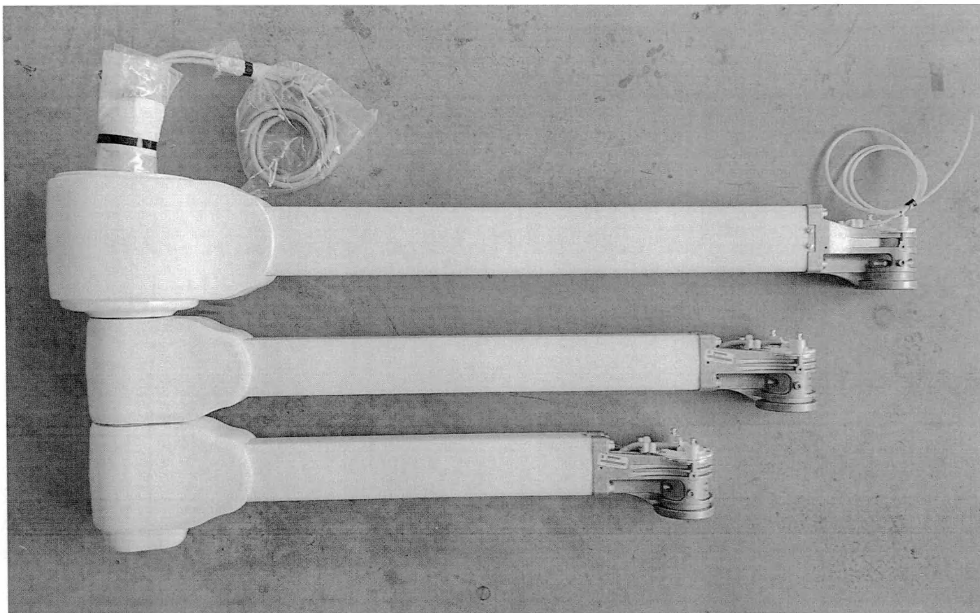
Замок центральный для 3-х плеч
