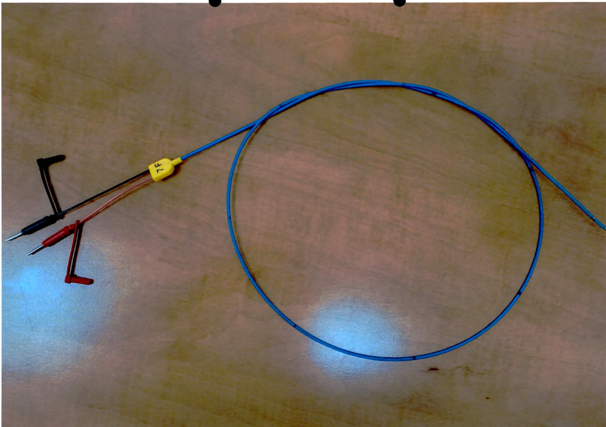
Фотография 7 – Общий вид Electroда для временной кардиостимуляции эндокардиального ESM4P010-115
