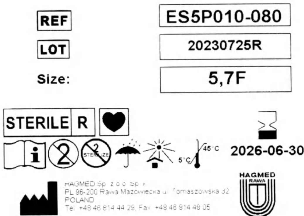
Рисунок 5 – Макет маркировки групповой (транспортной) упаковки
