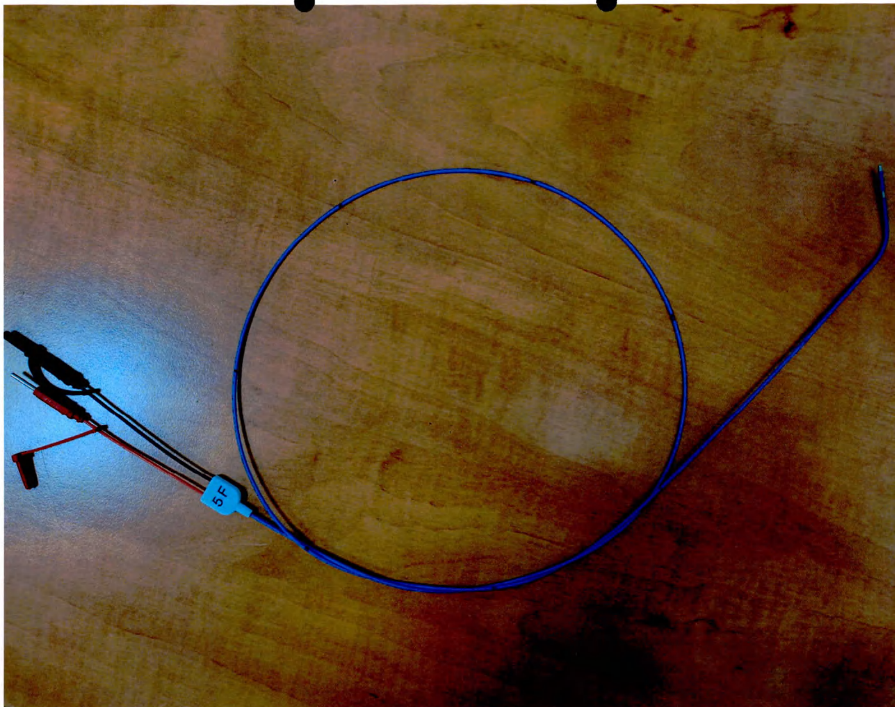
Фотография 8 – Общий вид Electroда для временной кардиостимуляции эндокардиального ES2Z010-115
