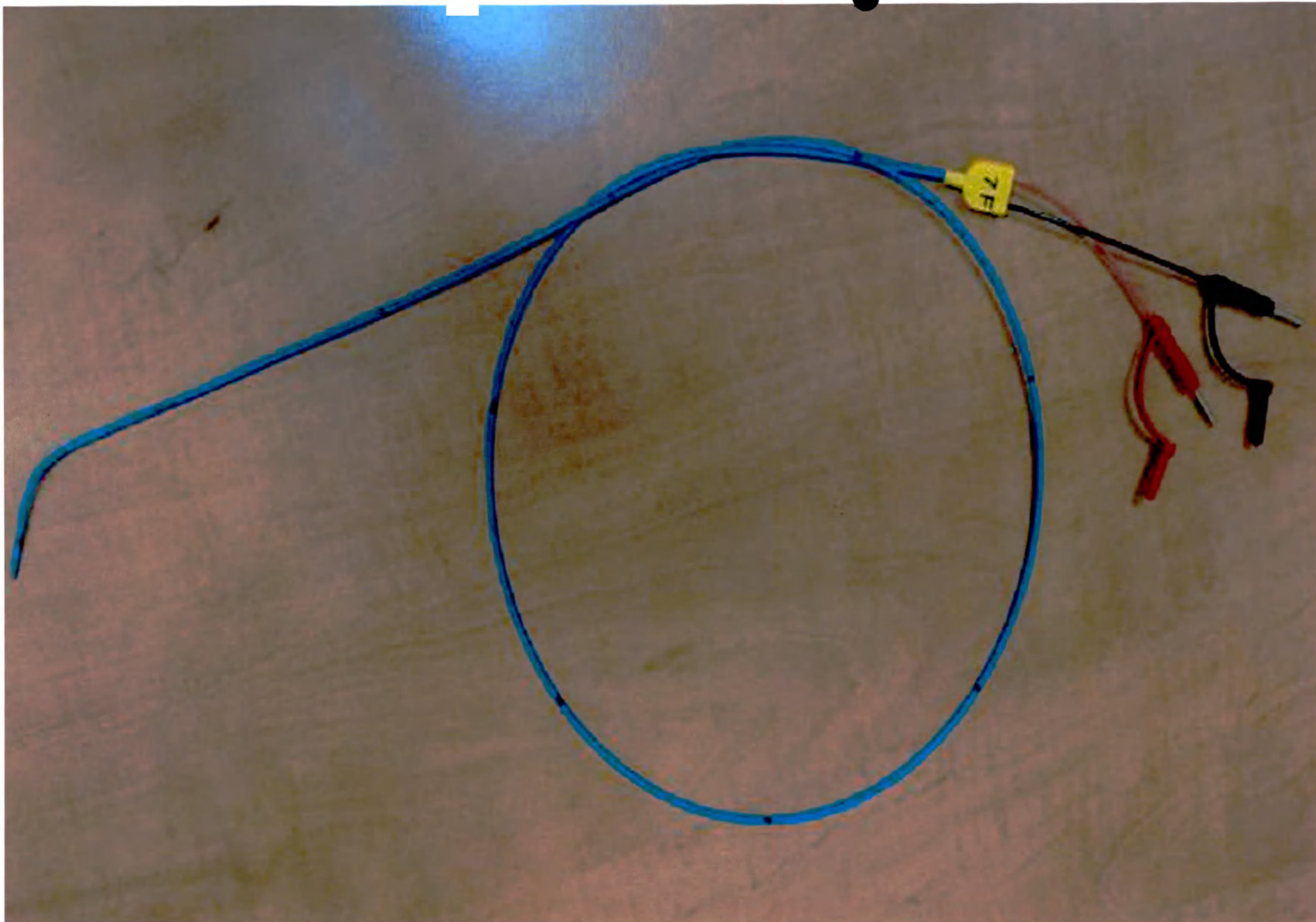
Фотография 3 – Общий вид Electroда для временной кардиостимуляции эндокардиального ESM4Z010-115
