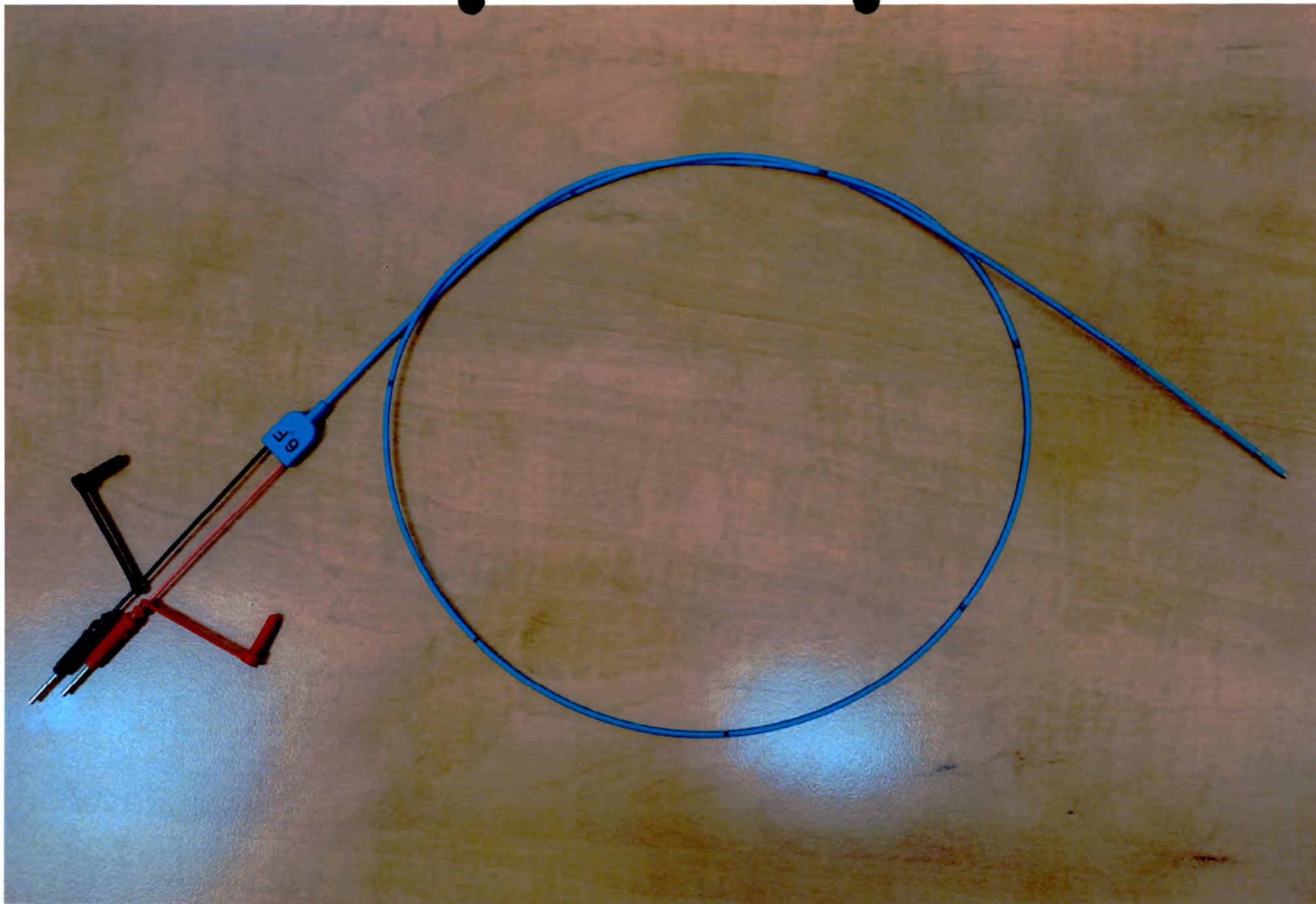
Фотография 6 – Общий вид Electroда для временной кардиостимуляции эндокардиального ESM3P010-115
