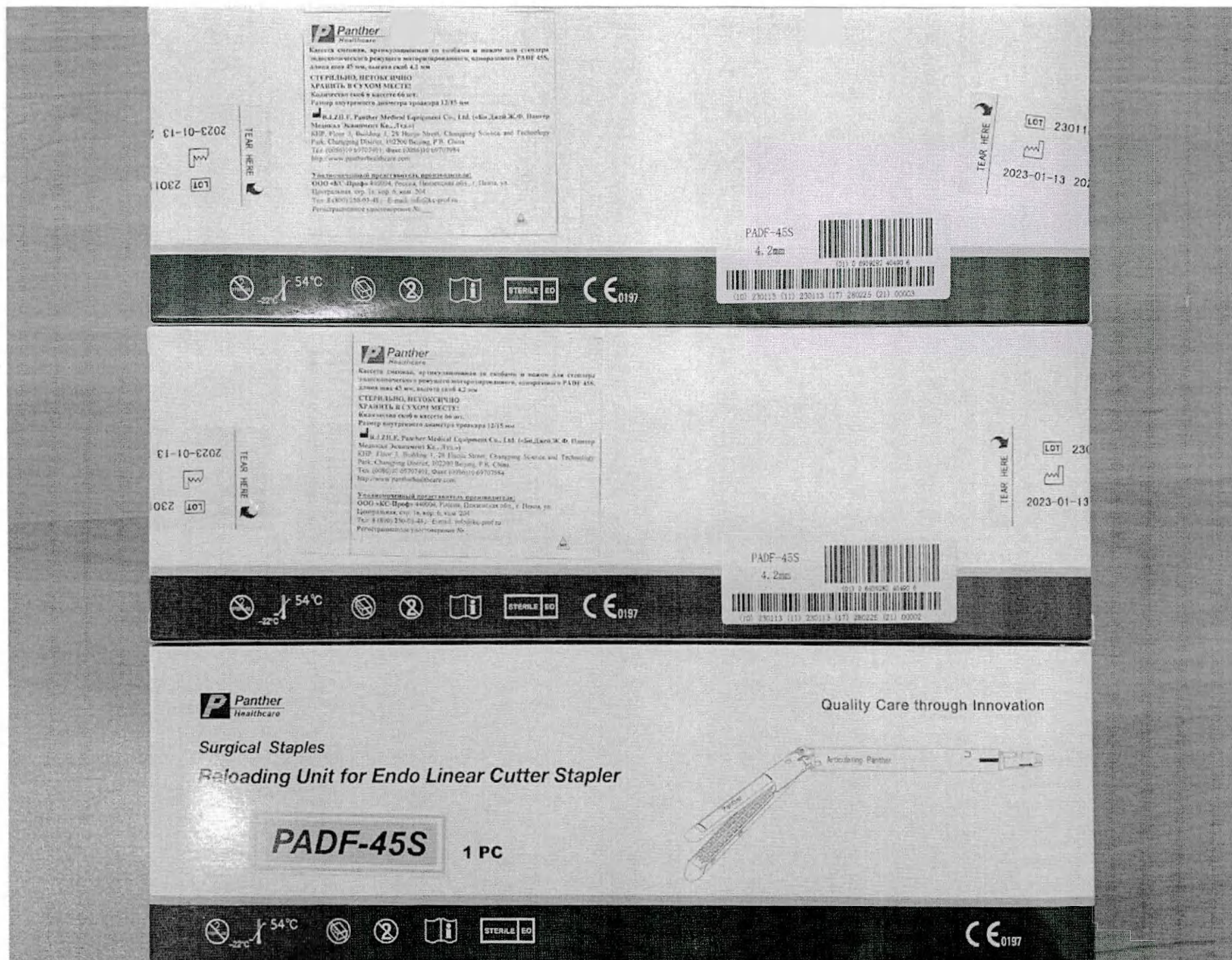
Рис. 47 Кассета сменная, артикуляционная со скобами и ножом для степлера эндоскопического режущего моторизированного, одноразового PADF-45S, длина шва 45 мм, высота скоб 4,2 мм, вторичная упаковка
