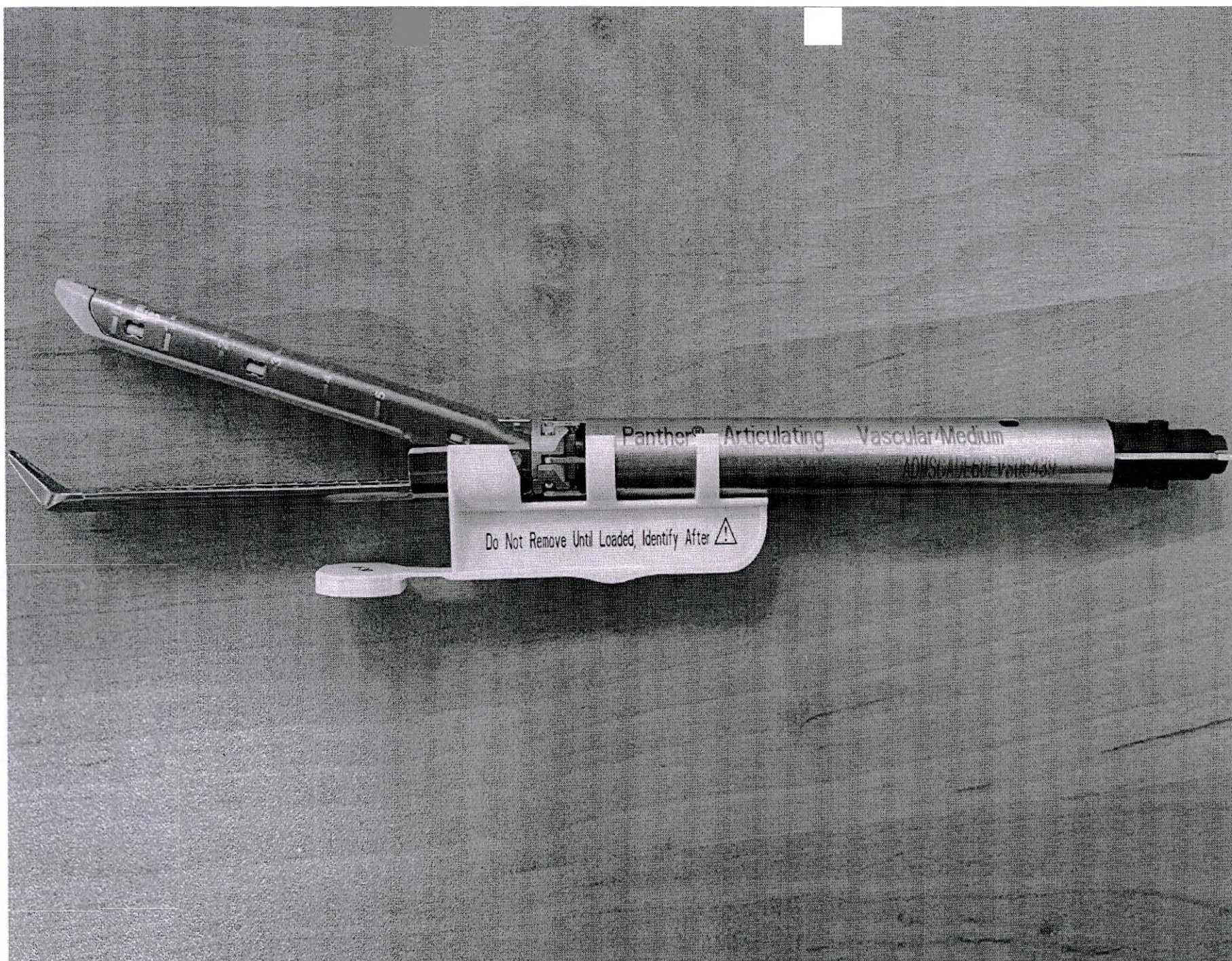
Рис. 46 Общий вид изделия
