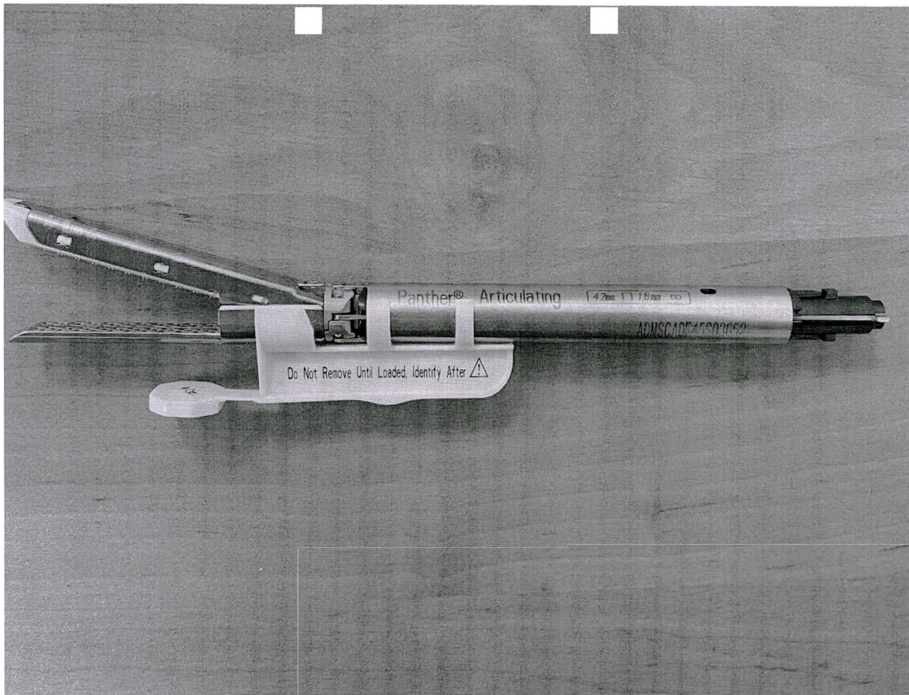
Рис. 52 Общий вид изделия
