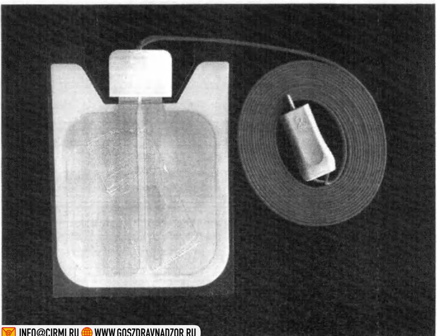
Нагревательный элемент отоплительной системы с номинальной мощностью: 70 Вт, составной, кабель 3 м (припуск 818-072)
