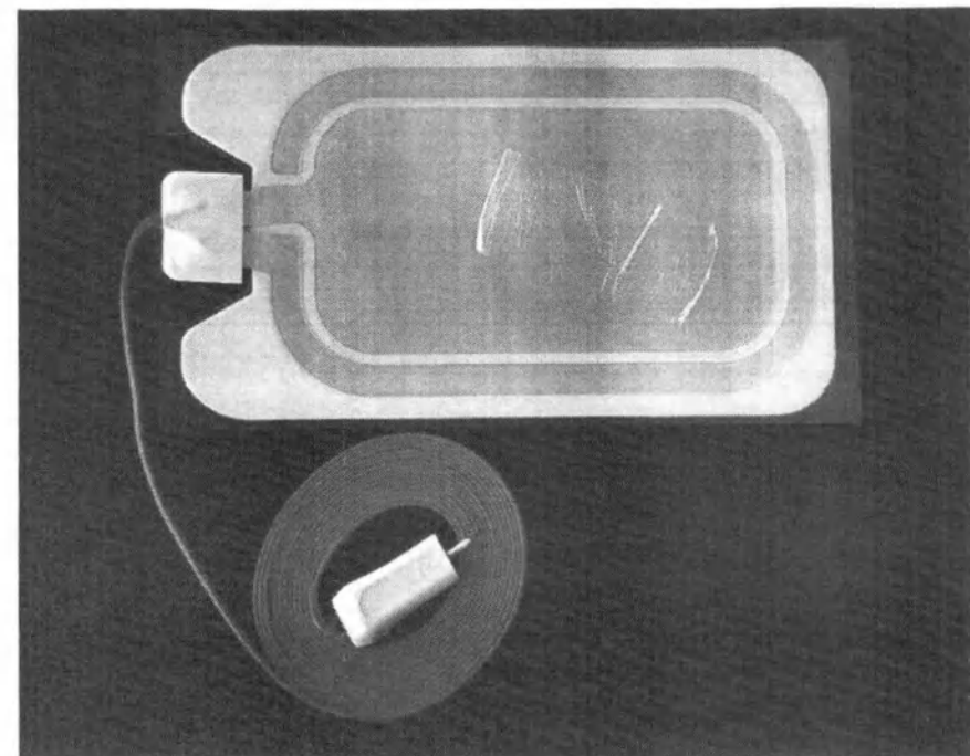
Нейтральные электроды одноразовые с принадлежностями: Нейтральный электрод одноразовый, 160 см 2 , составной, кабель 3 м, EASY (артикул 818-162)
