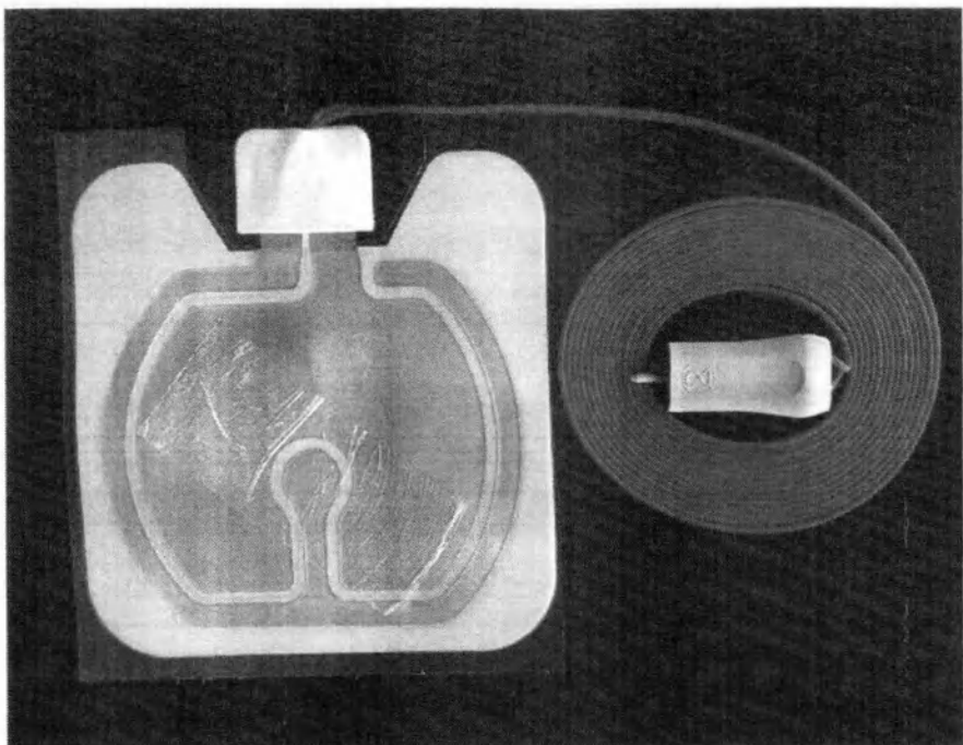
Нагревательный элемент отоплительной системы с номинальной мощностью: 70 Вт, составной, кабель 3 м, ЕАНВ (припуск 818-072)
