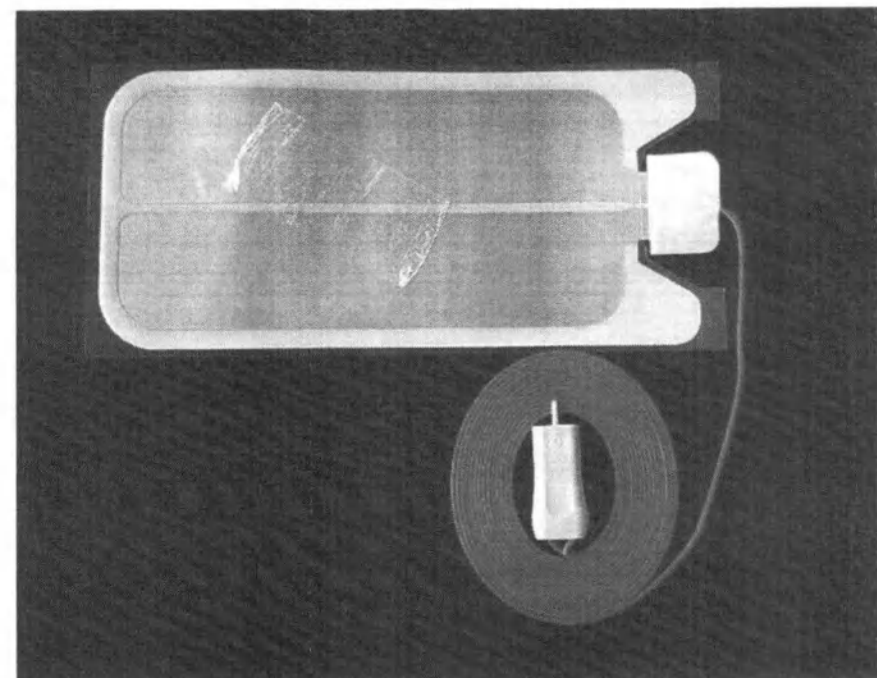
Нейтральные электроды одноразовые с принадлежностями: Нейтральный электрод одноразовый, 140 см 2 , составной, кабель 3 м (артикул 818-141)
