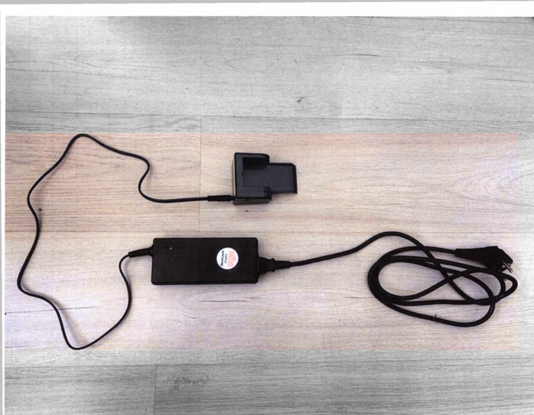
Цифровая портативная рентгеновская система ADX6000 (Зарядное устройство с сетевым шнуром, адаптером и подставкой)
