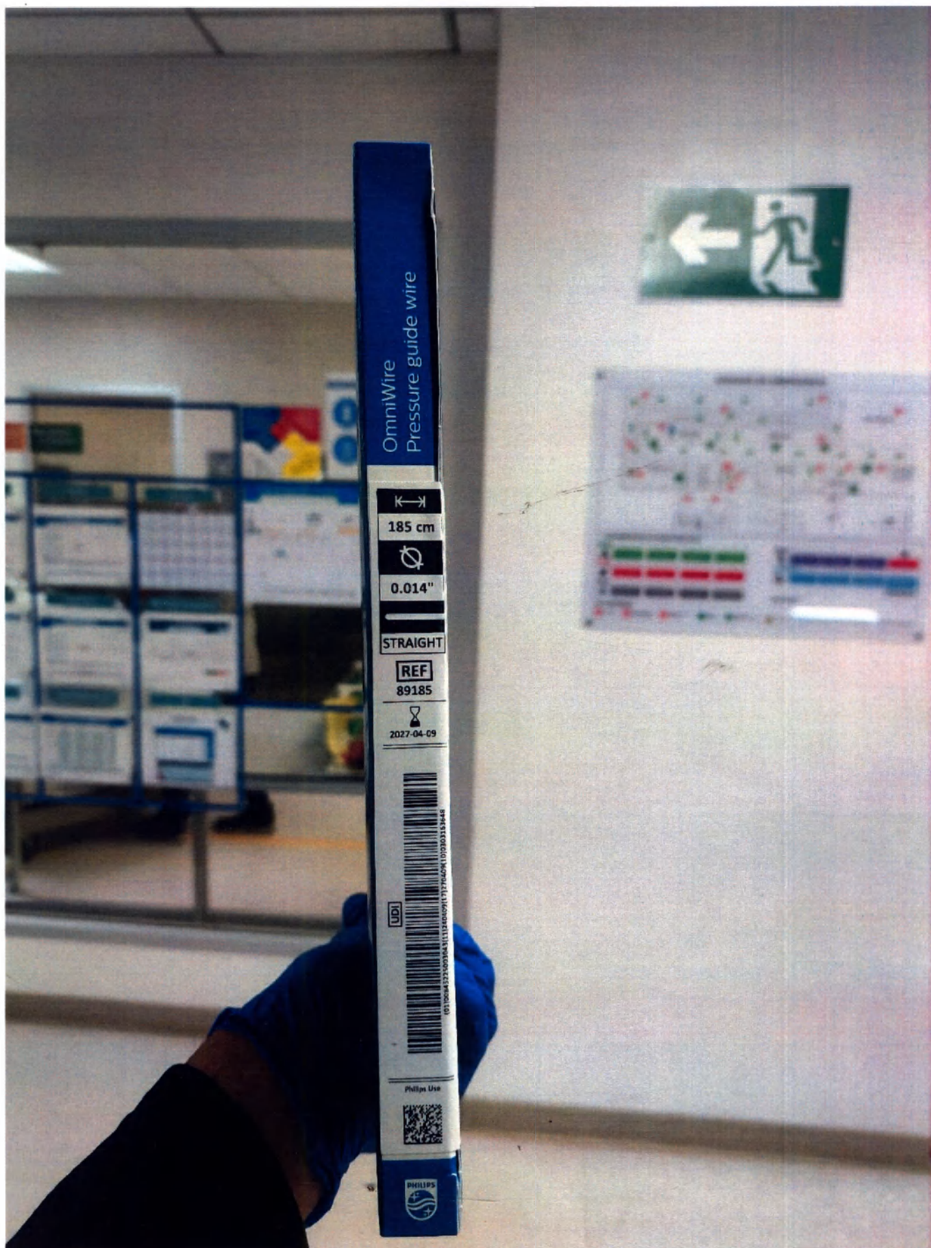
1.2 Проводник с датчиком давления OmniWire, длина 185 см, диаметр 0.36 мм, с прямым наконечником, с устройством для вращения. Упаковка.- вид сбоку
