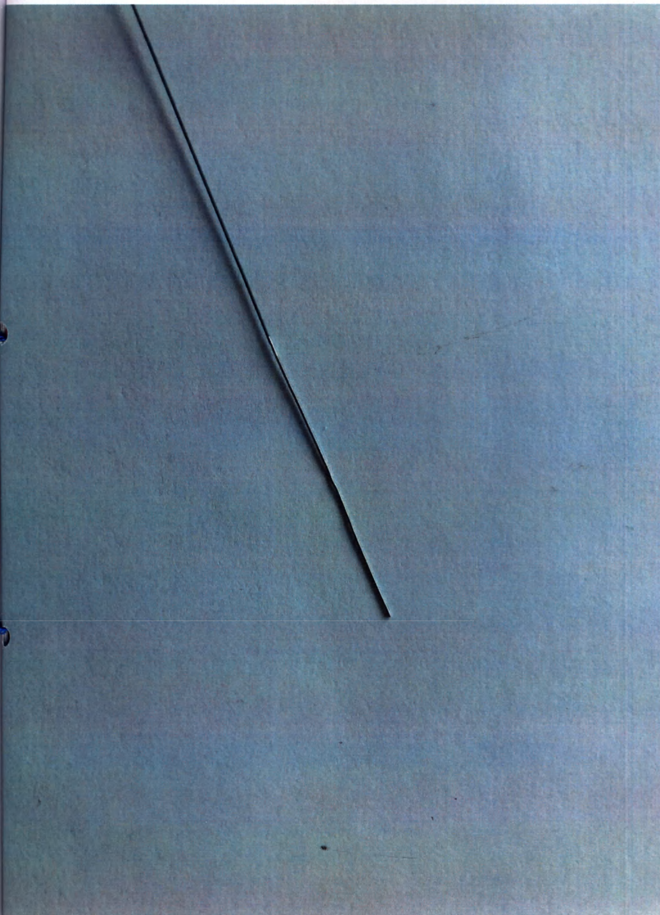
6 Проводник с датчиком давления OmniWire, длина 185 см, диаметр 0.36 мм, с прямым наконечником. наконечник проводника.
