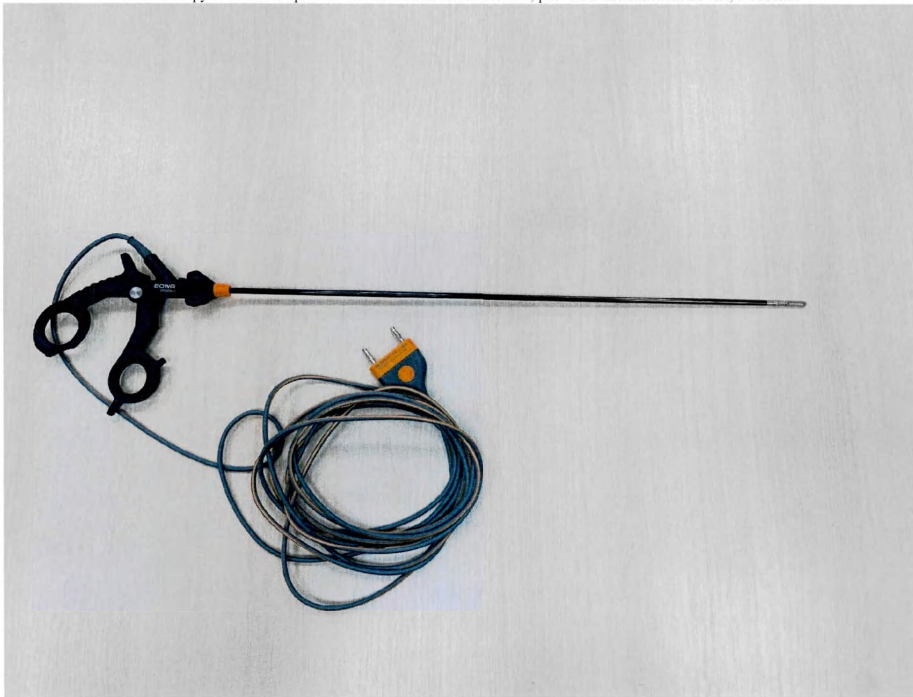
1.23. Инструмент биполярный ERGOeco окончатый 360 мм, разъем 2-контактный 28 мм, в составе
