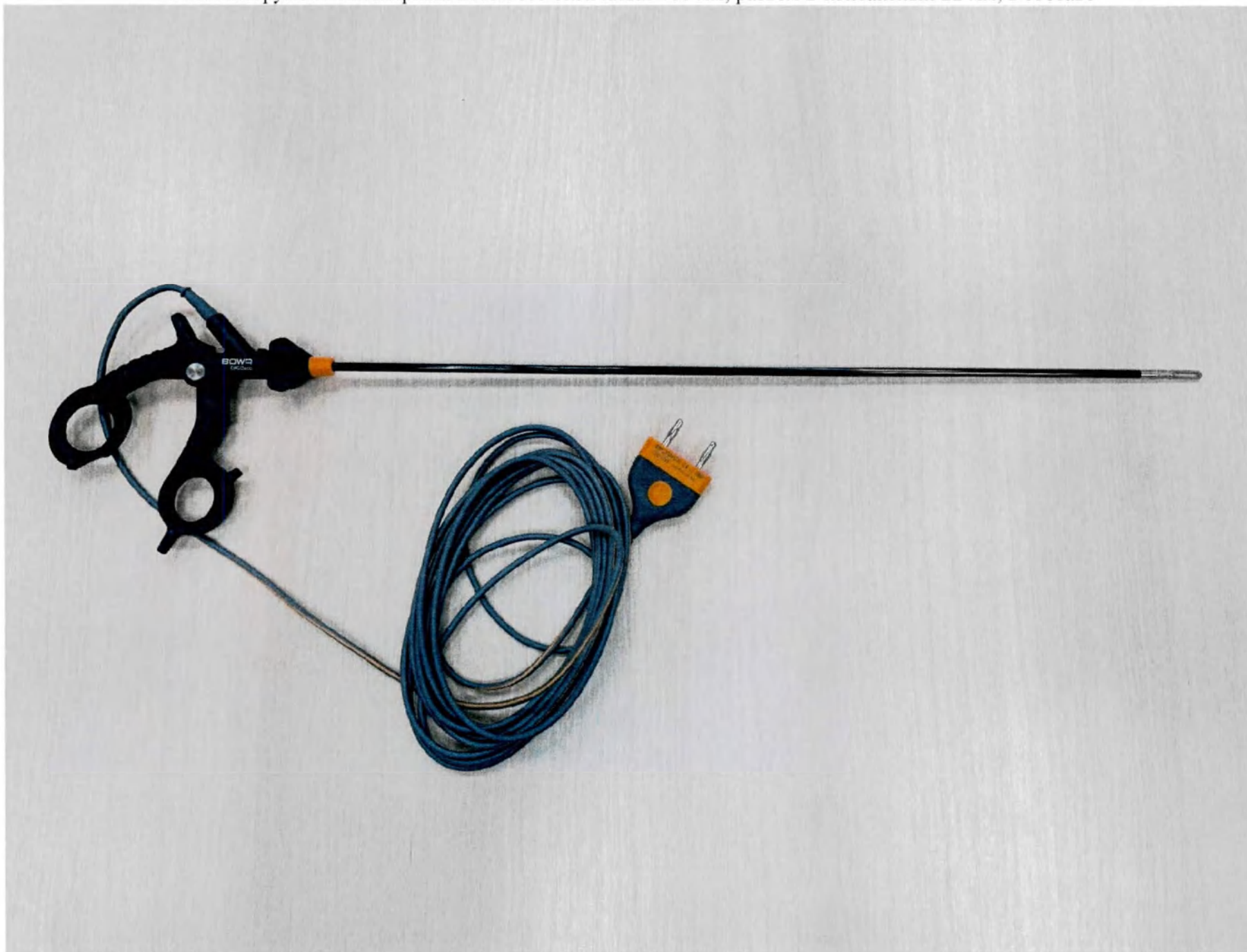
1.18. Инструмент биполярный ERGOeco окончатый 460 мм, разъем 2-контактный 22 мм, в составе
