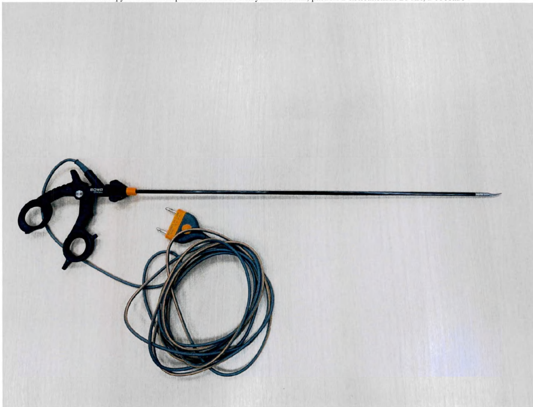
1.20. Инструмент биполярный ERGOeco Maryland 460 мм, разъем 2-контактный 28 мм, в составе
