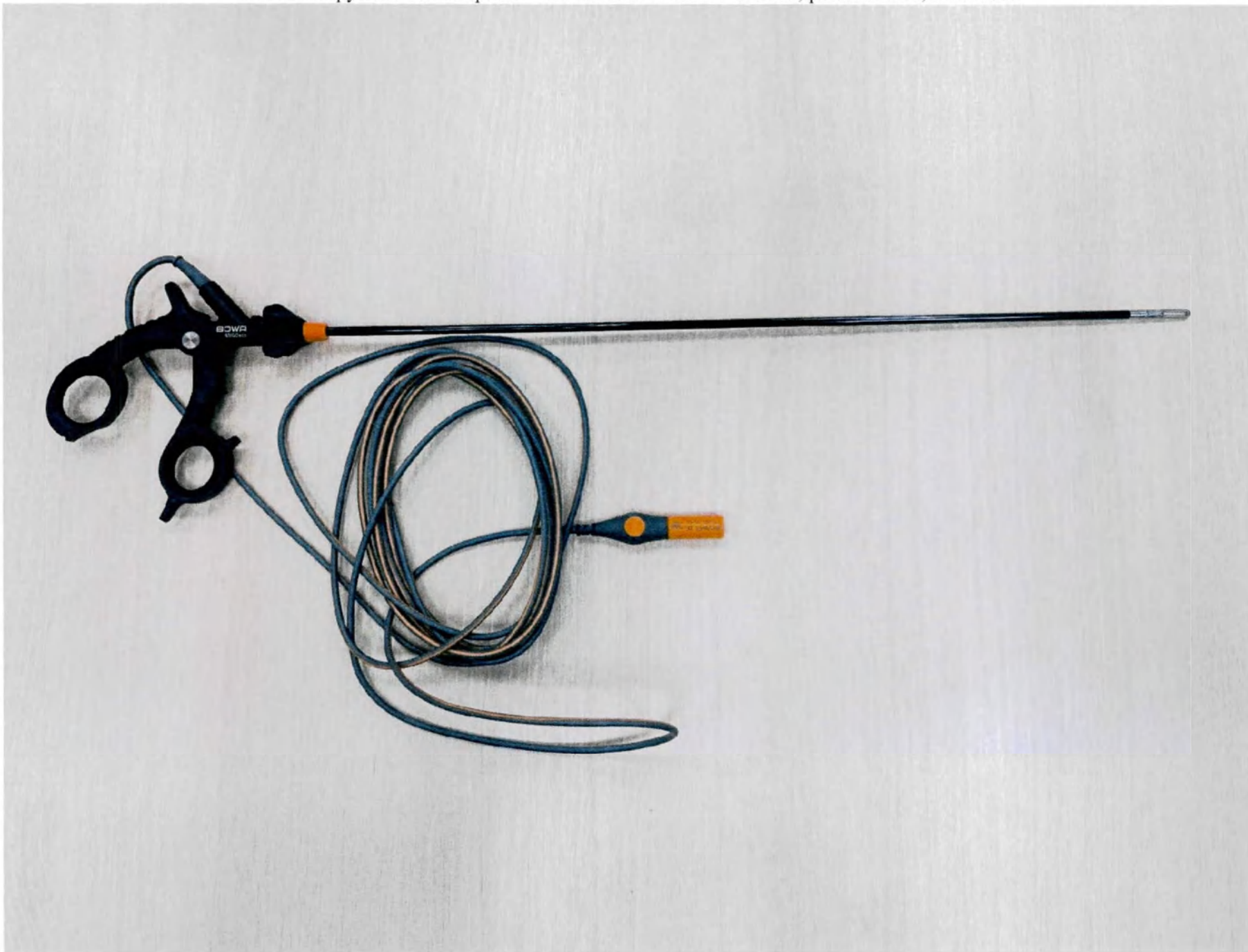
1.12. Инструмент биполярный ERGOeco окончатый 460 мм, разъем Erbe, в составе
