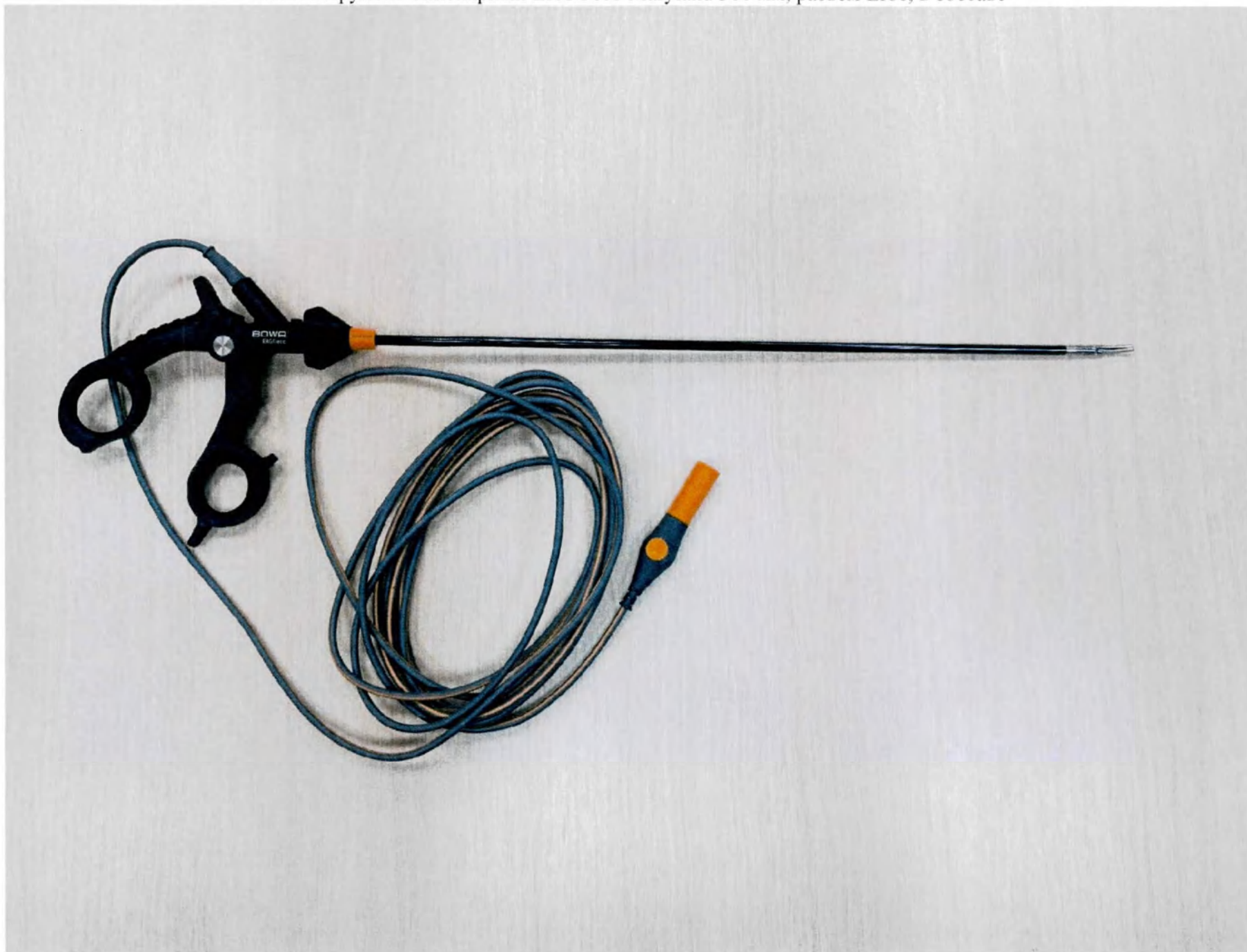
1.7. Инструмент биполярный ERGOeco Maryland 360 мм, разъем Erbe, в составе
