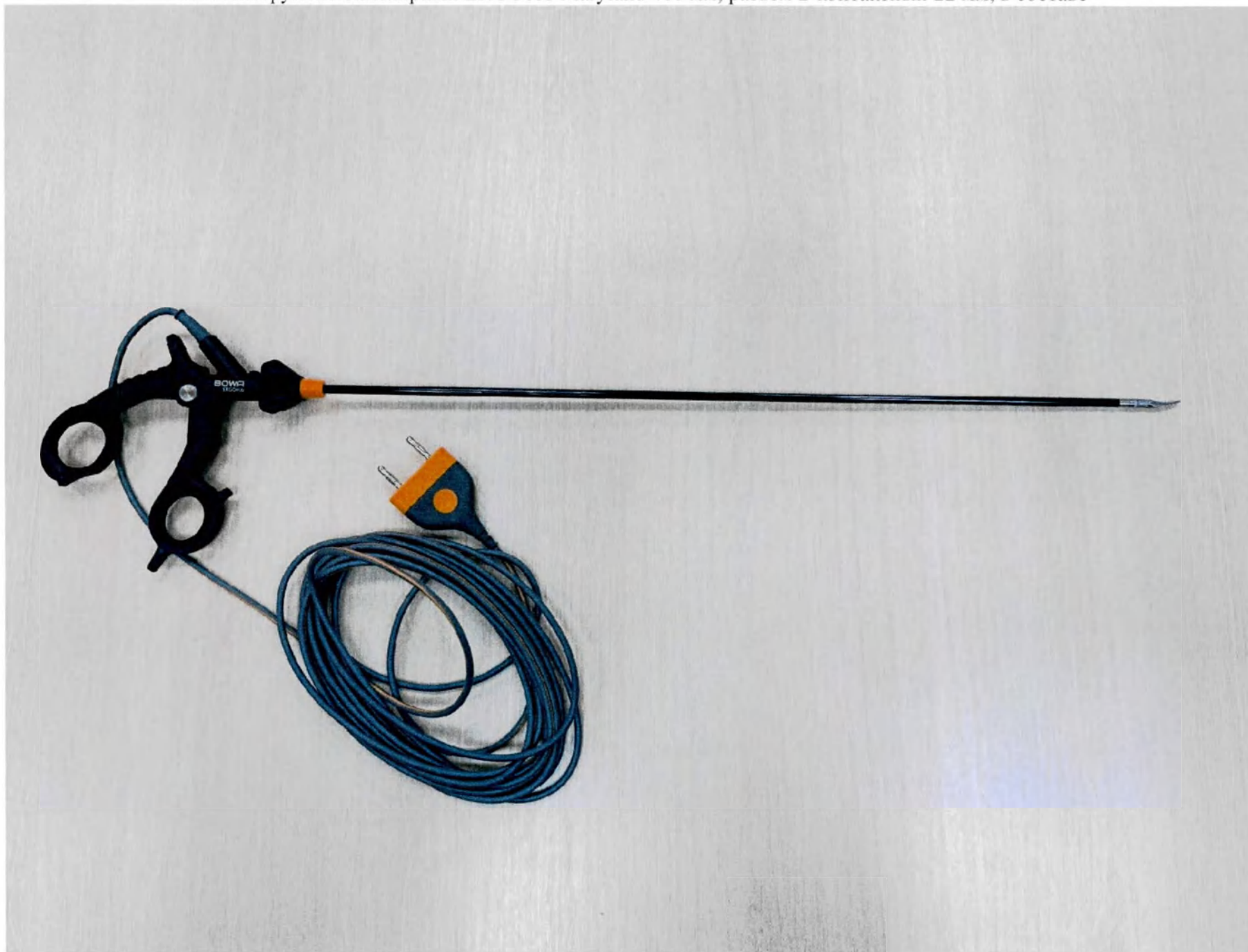
1.14. Инструмент биполярный ERGOeco Maryland 460 мм, разъем 2-контактный 22 мм, в составе
