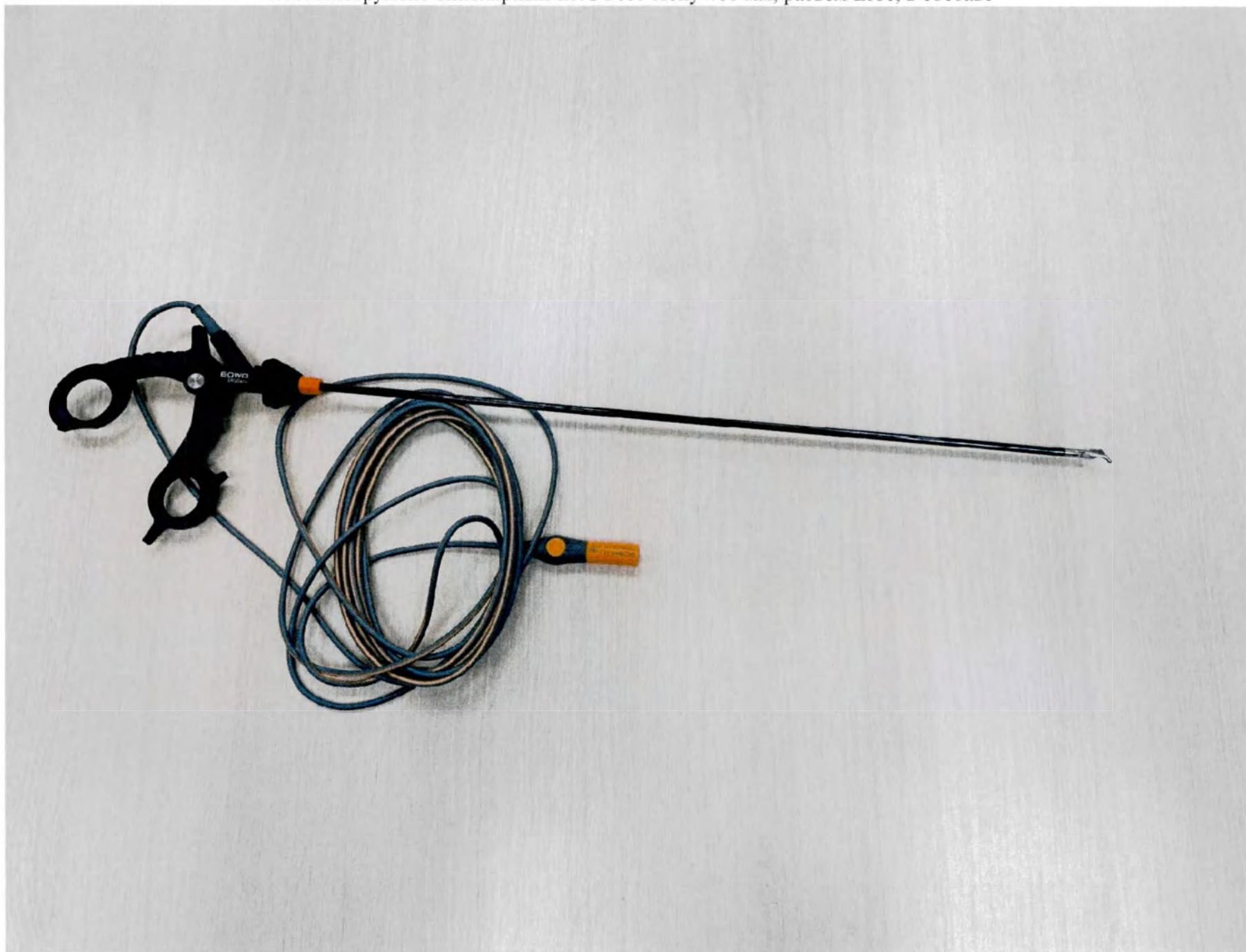
1.10. Инструмент биполярный ERGOeco Kelly 460 мм, разъем Erbe, в составе
