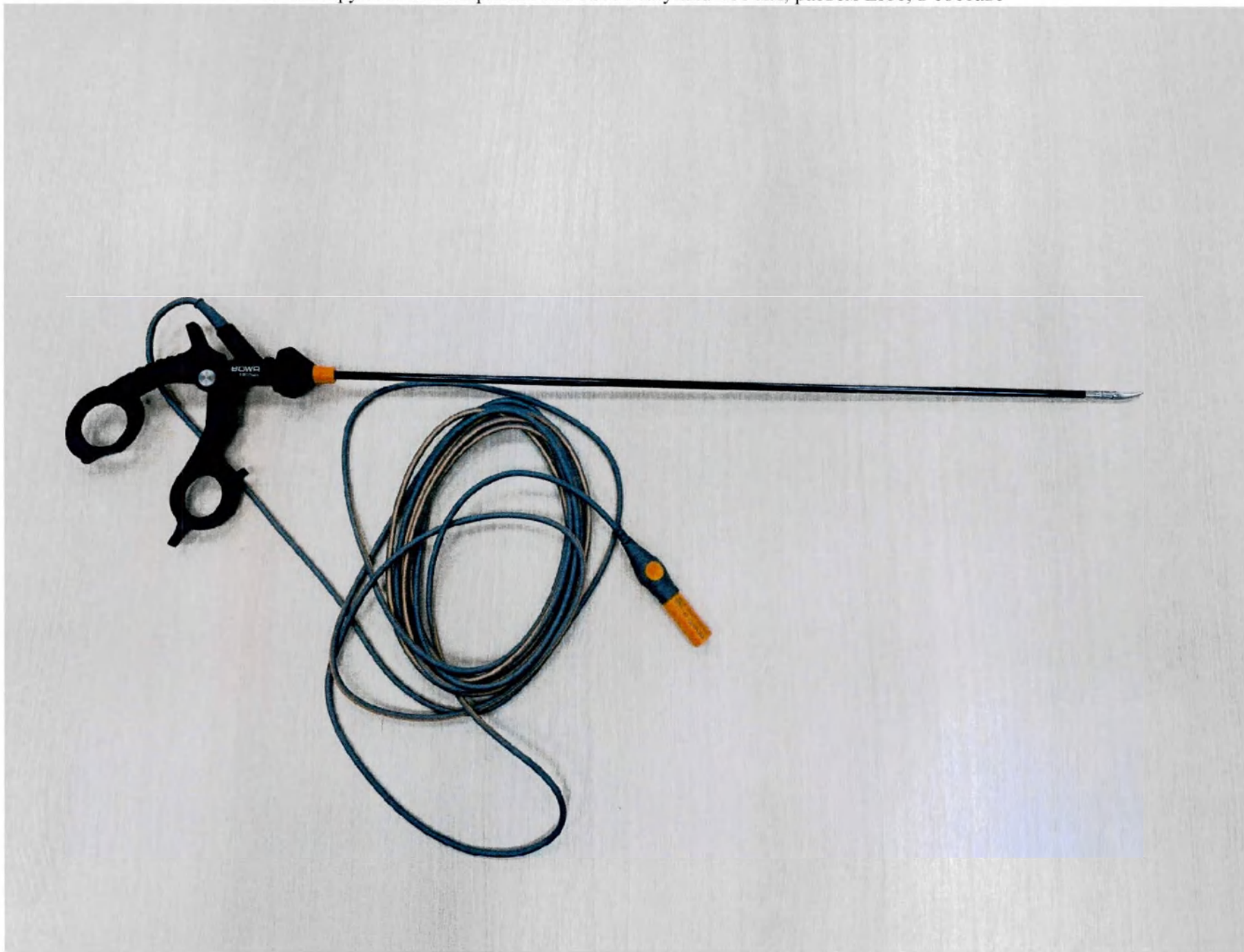
1.8. Инструмент биполярный ERGOeco Maryland 460 мм, разъем Erbe, в составе
