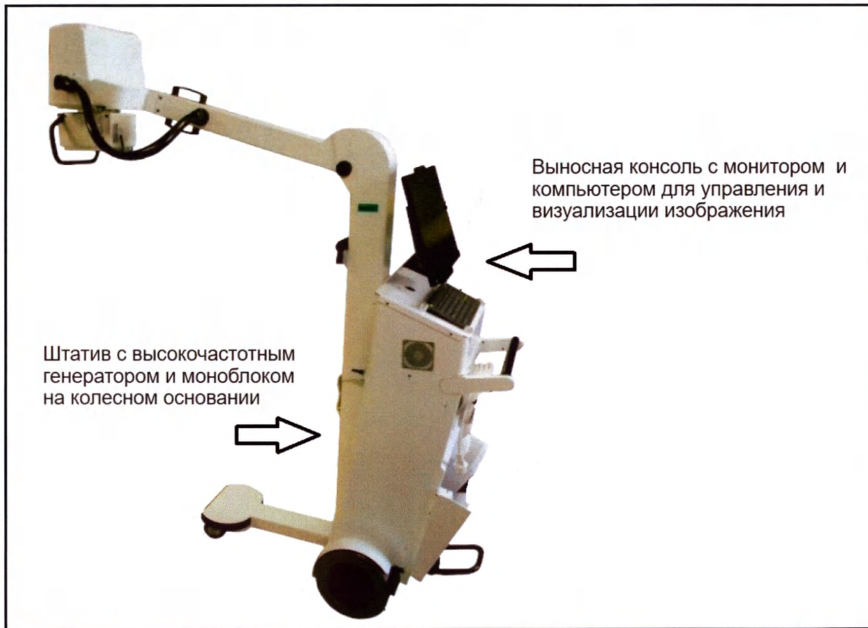
Исполнение 2: Аппарат рентгеновский передвижной Mobildrive с высокочастотным генератором в составе (общий вид)
