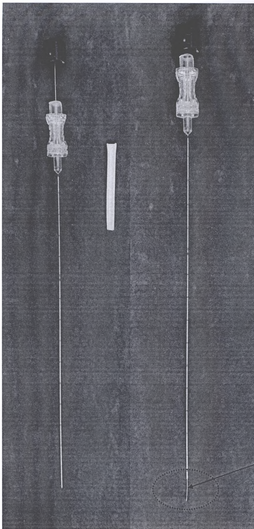
Общий вид медицинского изделия: Маркер для визуализации местоположения опухоли «ПКМед» одноразовый стерильный по TV 32.50.50-001-43254975-2020
