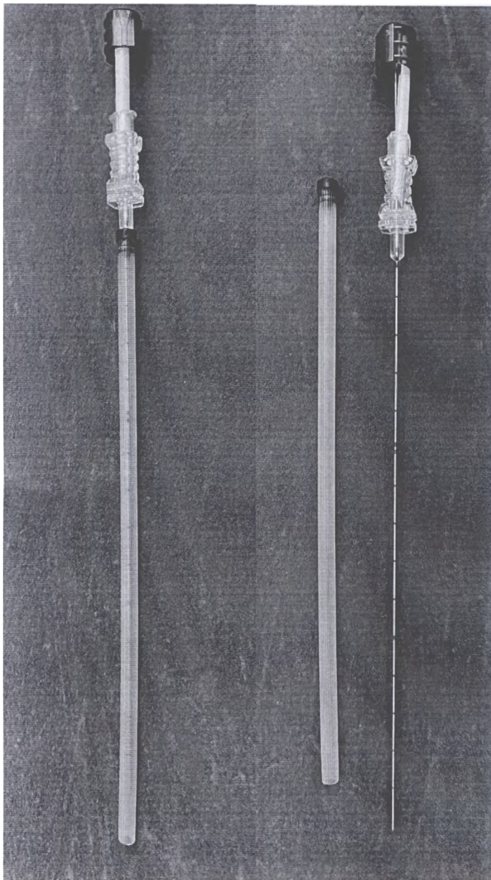
Общий вид медицинского изделия: Маркер для визуализации местоположения опухоли «ПКМед» одноразовый стерильный по ТУ 32.50.50-001-43254975-2020
