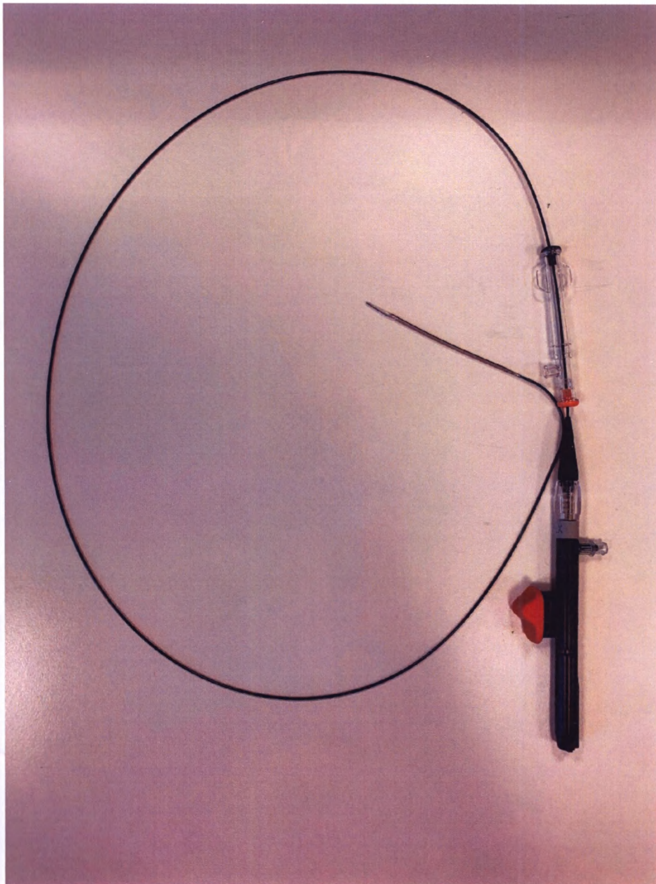
Рисунок 8. Система направленной атерэктомии HawkOne, вариант исполнения H1-LX-INT
