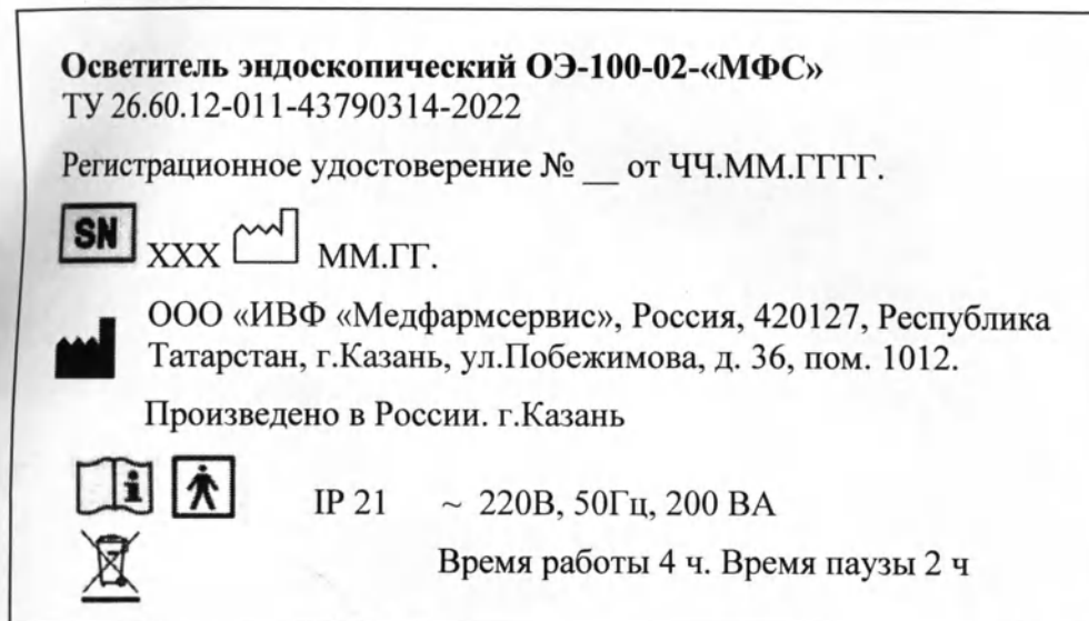
Рис. 2.1. Маркировочная табличка на задней стенке блока осветителя*
