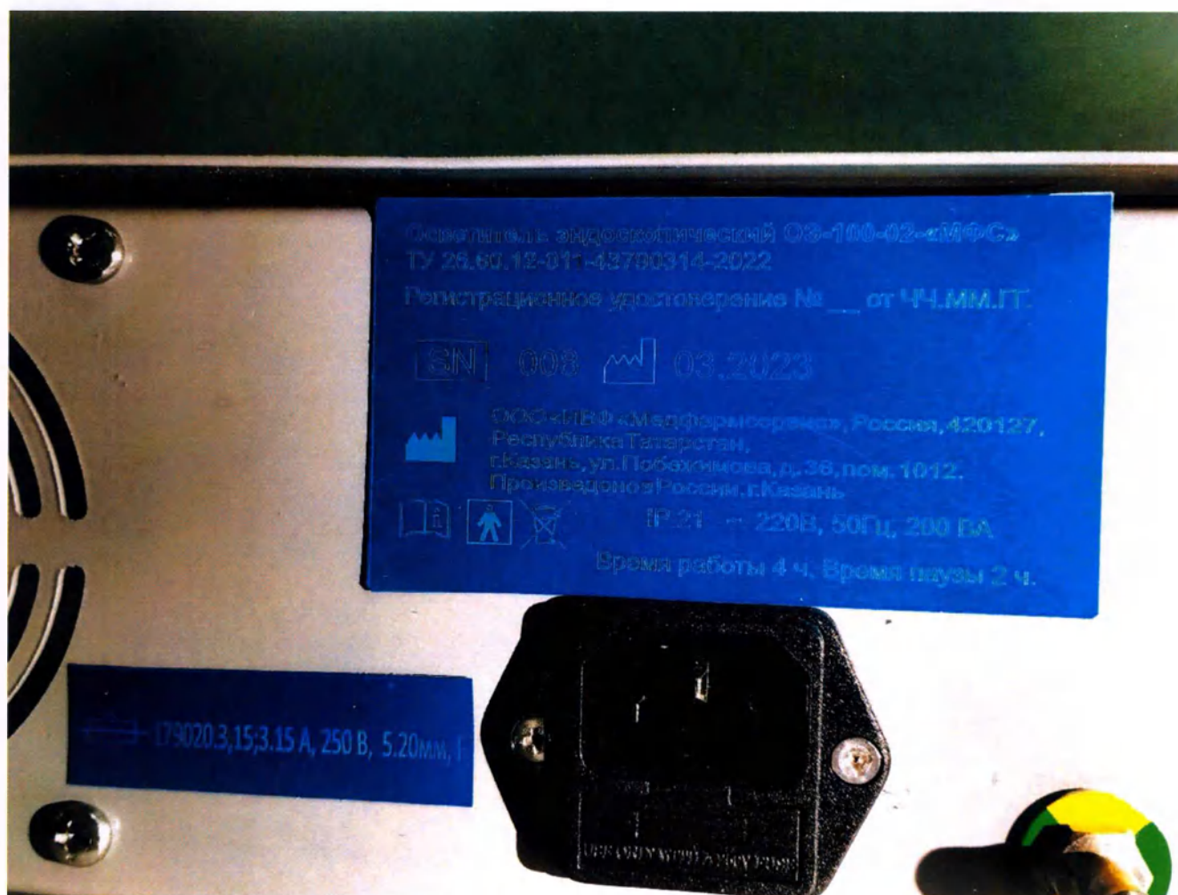
Фото 6. Общий вид маркировки изделия. Блок осветителя эндоскопического ОЭ-100-02-«МФС»
