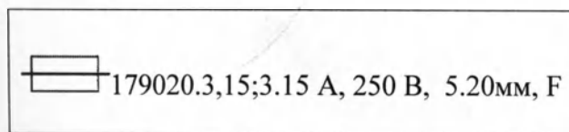
Рис.2.2. Маркировочная табличка на задней стенке блока осветителя (место расположения: на корпусе осветителя, рядом с предохранителем)
