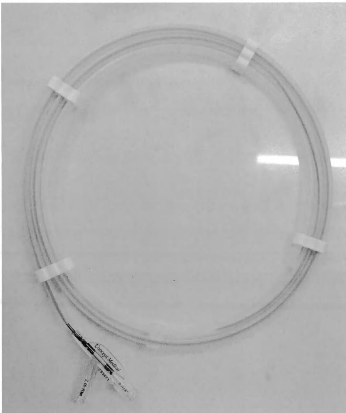
Общий вид изделия в защитном диспенсере (защитный круговой лоток) на примере «Катетер баллонный для ЧТА покрытый сиролимусом Magic Touch PTA (0.018"OTW) /Magic Touch PTA Sirolimus Coated PTA Balloon Catheter (0.018"OTW)», вариант исполнения: CPT18200080, Диаметр баллона 2.00 мм, Длина баллона 80 мм, Эффективная длина катетера 120 см 1
