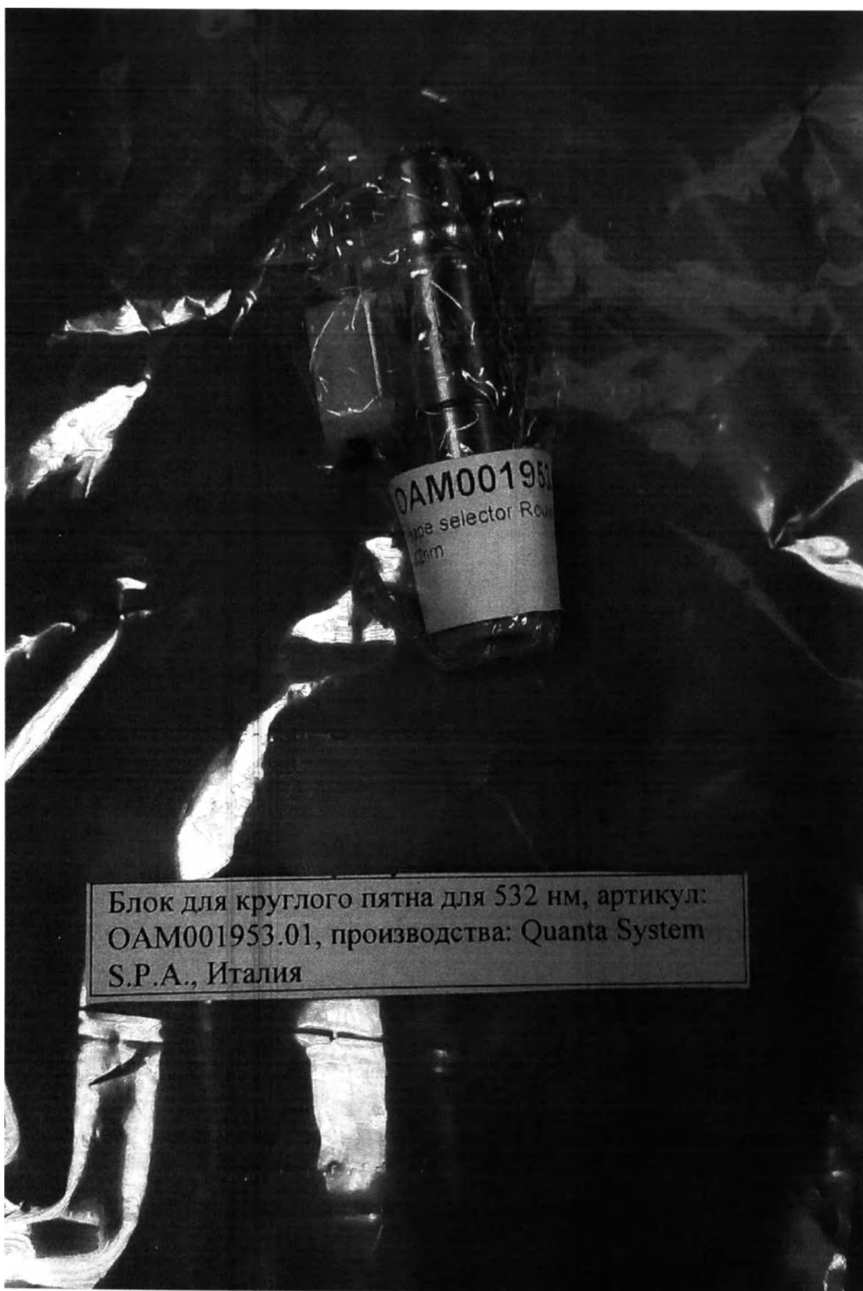
Блок для круглого пятна для 532 нм, артикул: OAM001953.01
