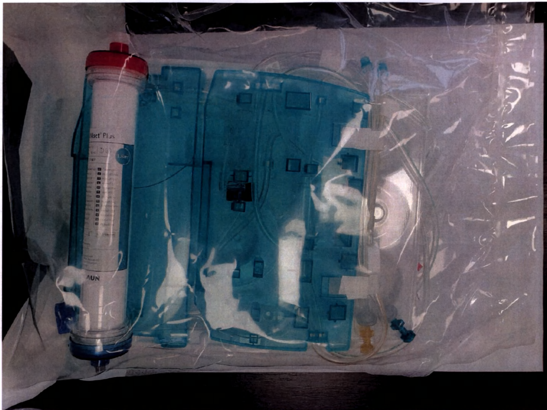
Рис.3. Набор кровопроводящих магистралей OMNIset® Plus с гемофильтром OMNIfilter® 1,6 м2, к аппарату для экстракорпоральной очистки крови OMNI®.
