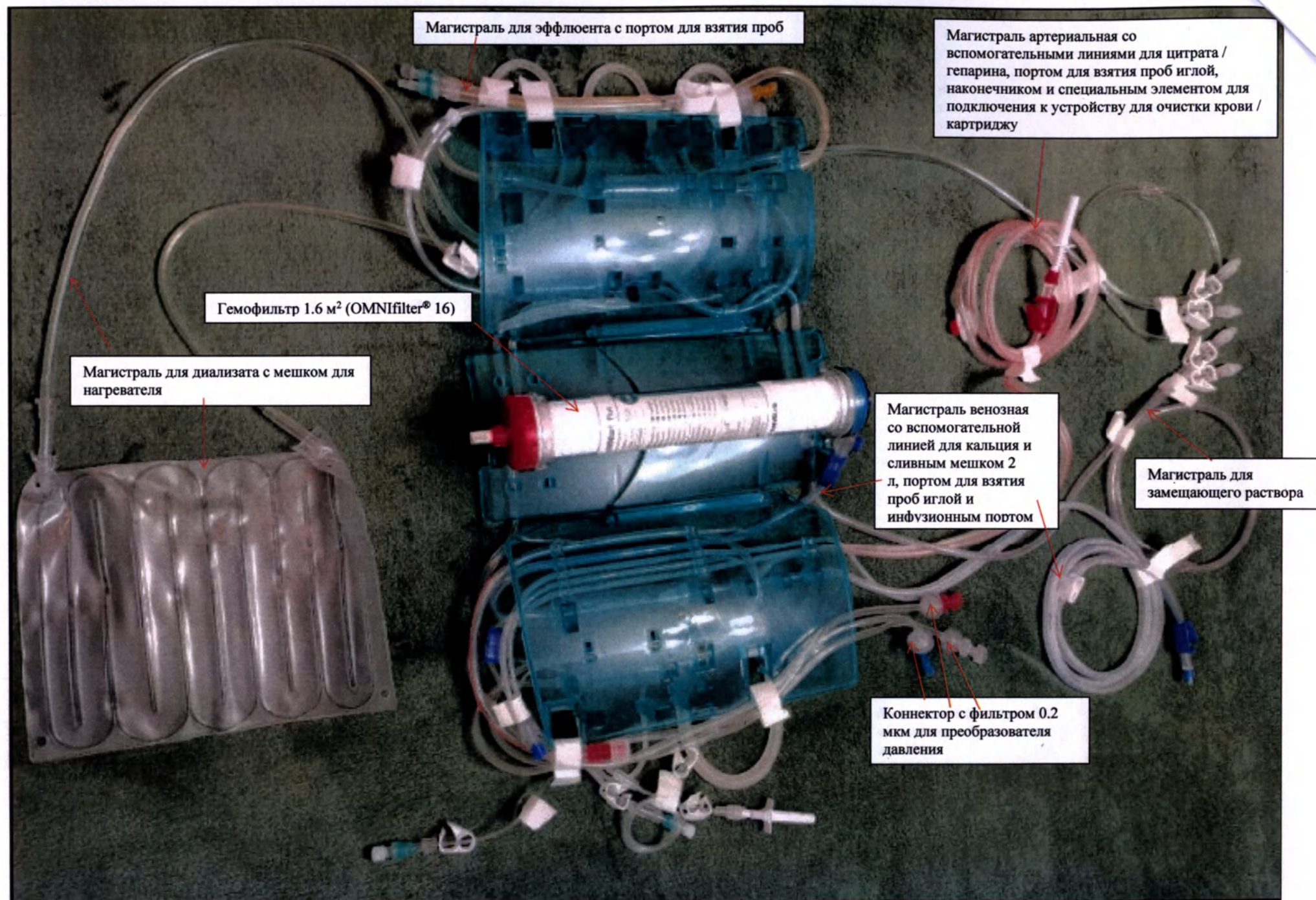
Рис 4. Набор кровопроводящих магистралей OMNIset® Plus с гемофильтром OMNIfilter® 1,6 м 2 , к аппарату для экстракорпоральной очистки крови OMNI®.
