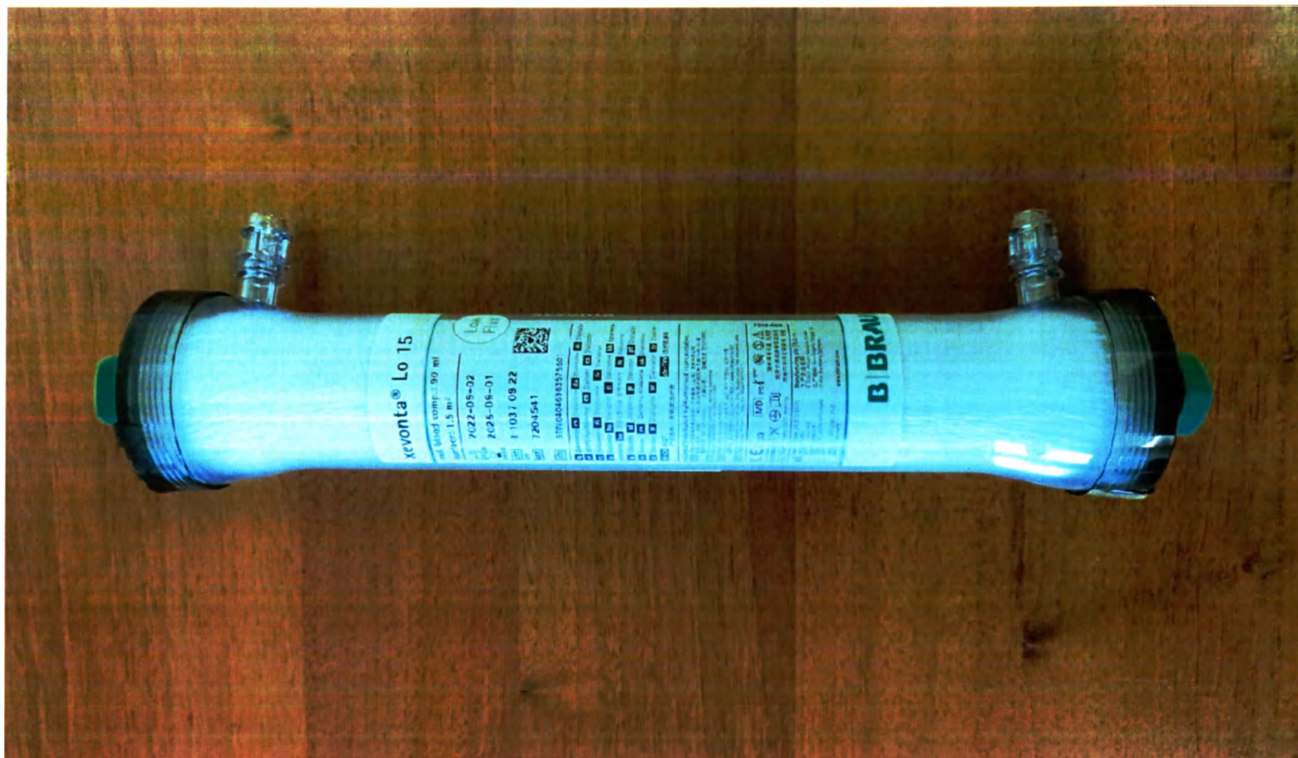
Рисунок 2 – Диализатор Ксевонта (кевонта) низкотоочный Lo 15 без индивидуальной упаковки
