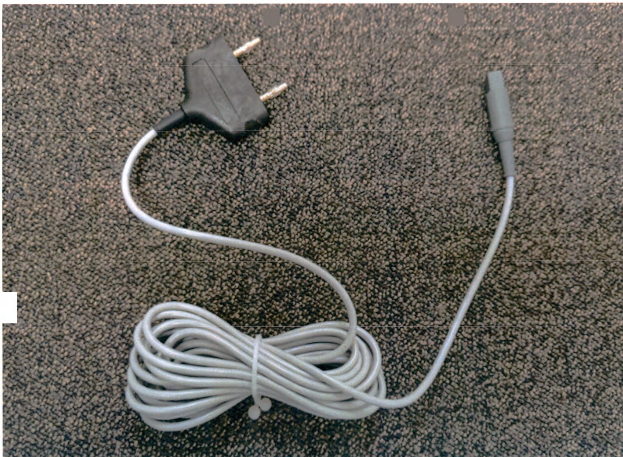
Кабель (из состава «Биполярный пинцет модульный»). Общий вид
