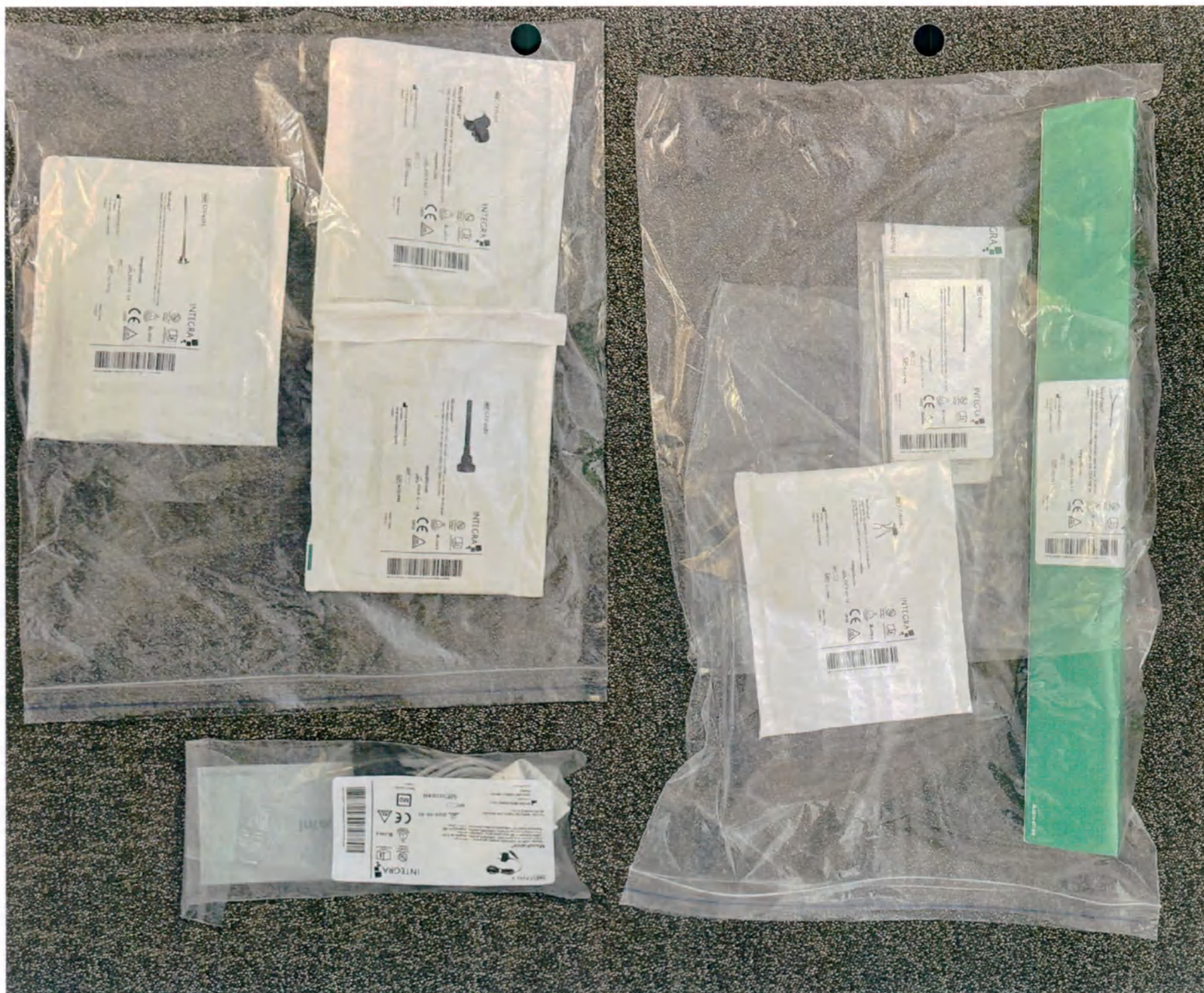
Биполярный пинцет модульный (в составе: Биполярный пинцет модульный в составе: Рукоятка угловая, Трубка прямая, Наконечник пинцета фенестрированный; Троакары в составе: Наконечник троакара, Головка, Корпус). Общий вид изделия в упаковке
