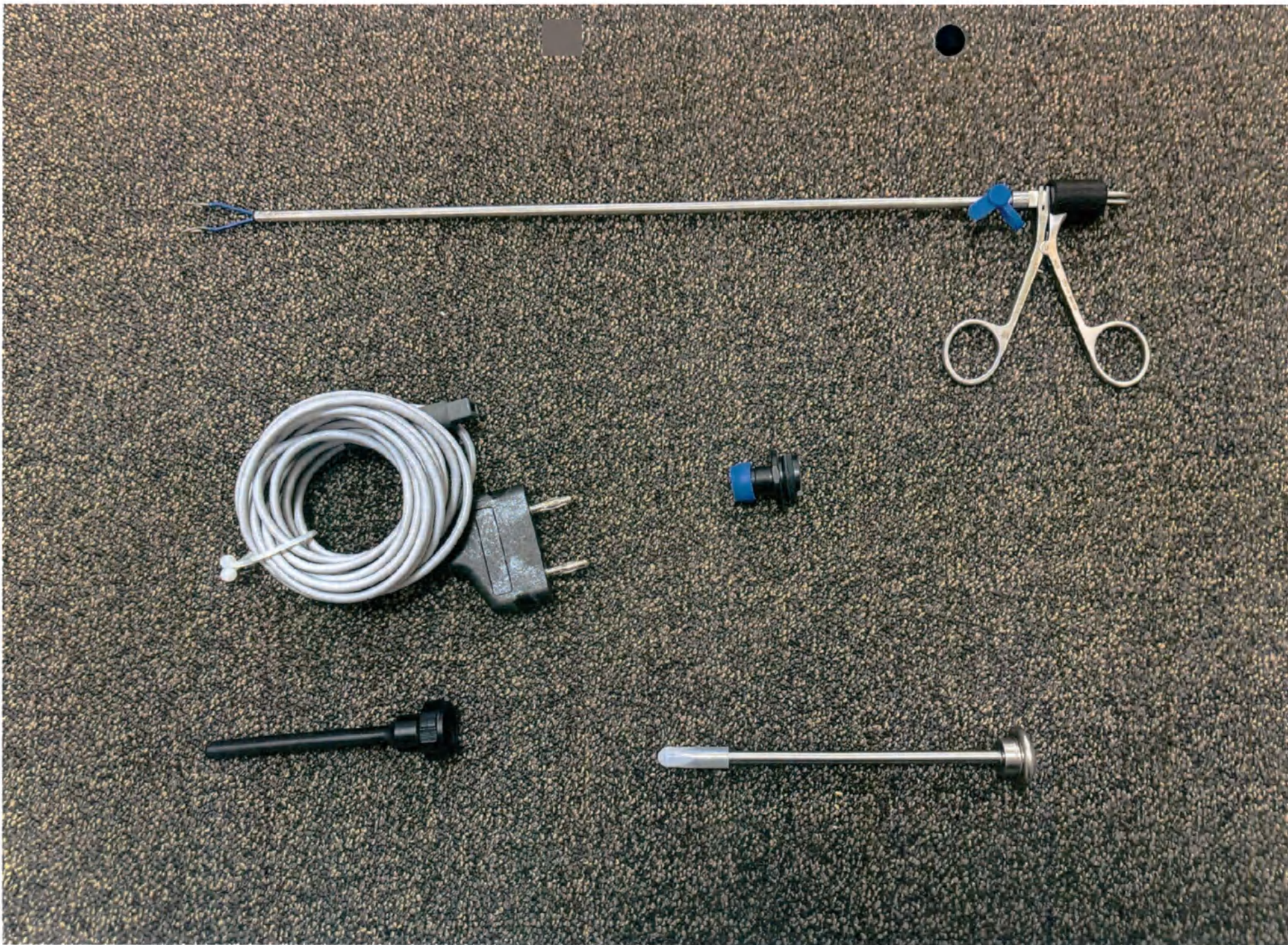
Биполярный пинцет Botella (в составе: Биполярный пинцет Botella, Кабель, Троакары в составе: Наконечник троакара, Головка, Корпус). Общий вид изделия без упаковки
