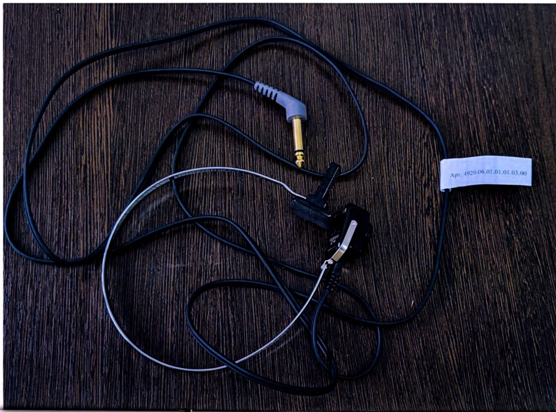
Костный вибратор с соединительным кабелем Radioear B71W, арт. 4920.06.01.01.01.03.00
