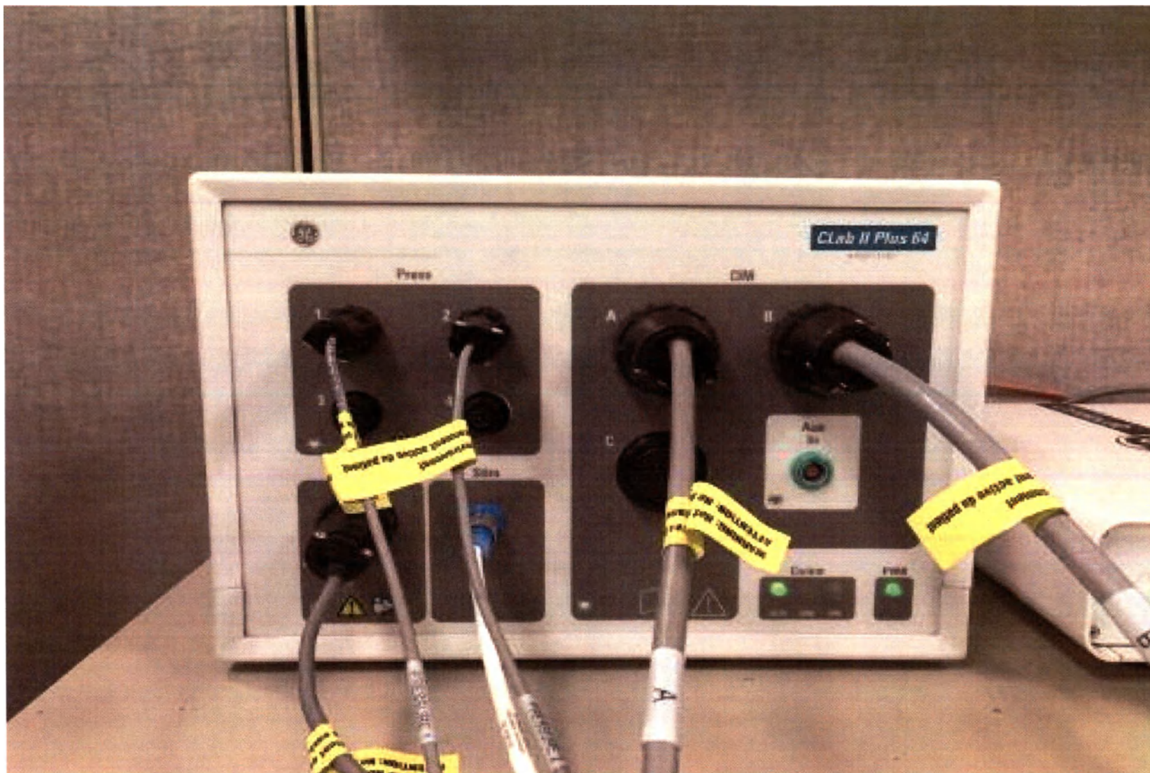
Фото 69. Кабели для усилителя электрофизиологических сигналов
