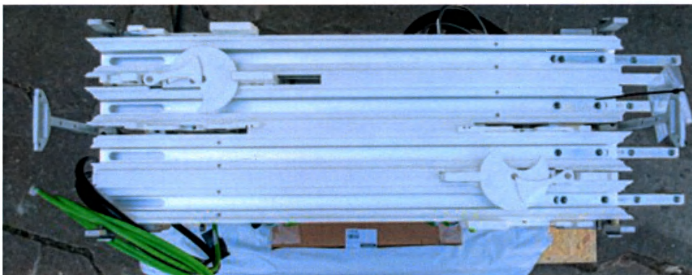
Транспортная линия с направляющим механизмом, 625 мм
