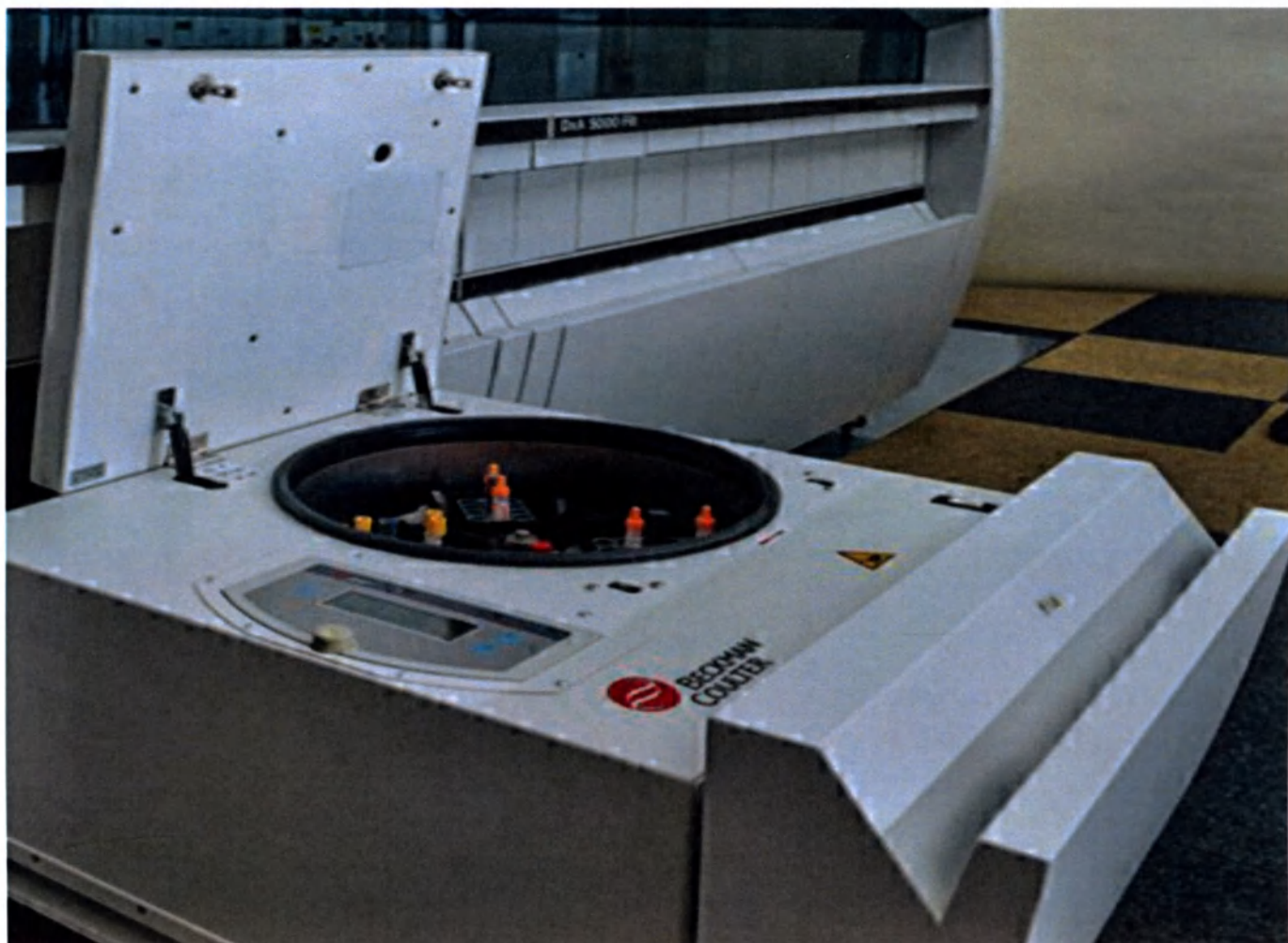
Модуль центрифугирования с одной центрифугой (DxA Automation System Centrifuge)
