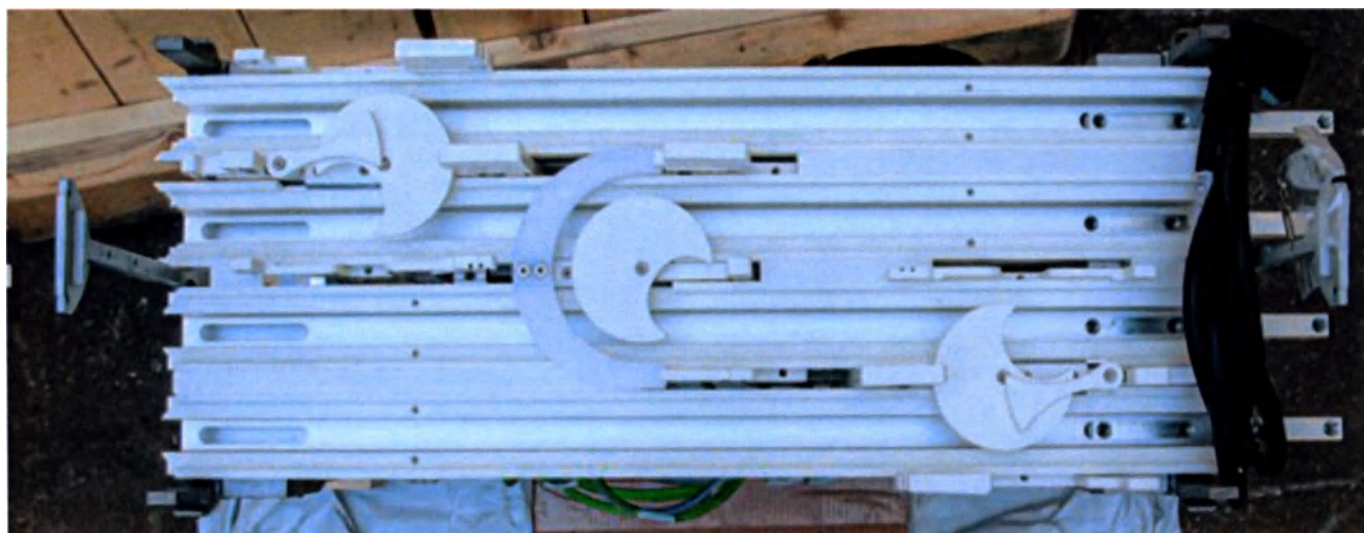
Транспортная линия с разворотным механизмом, 625 мм
