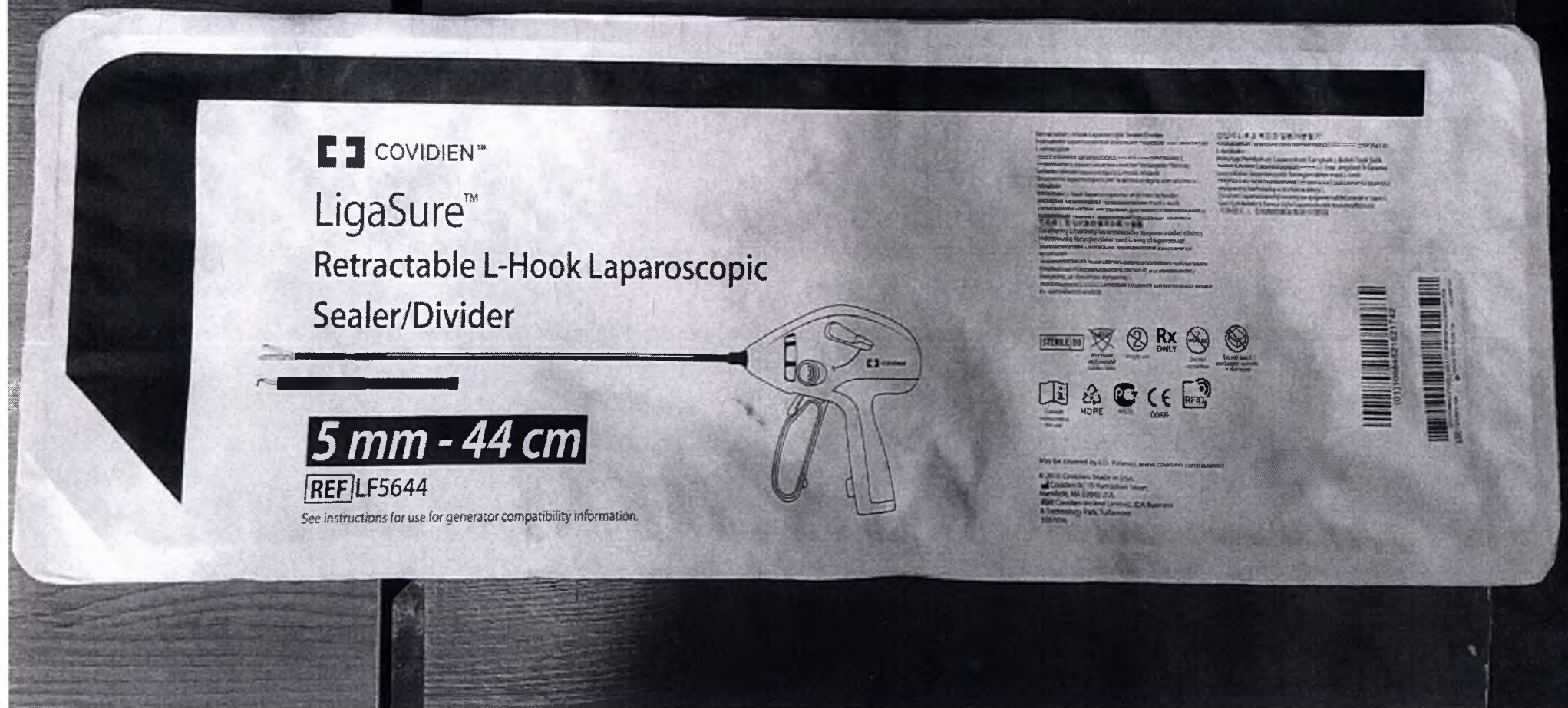
Фото 8. Лапароскопический инструмент LigaSure для электролигирования и разделения тканей с выдвижным Г-образным крючком диаметр стержня 5 мм, длина стержня 44 см; — Маркировка
