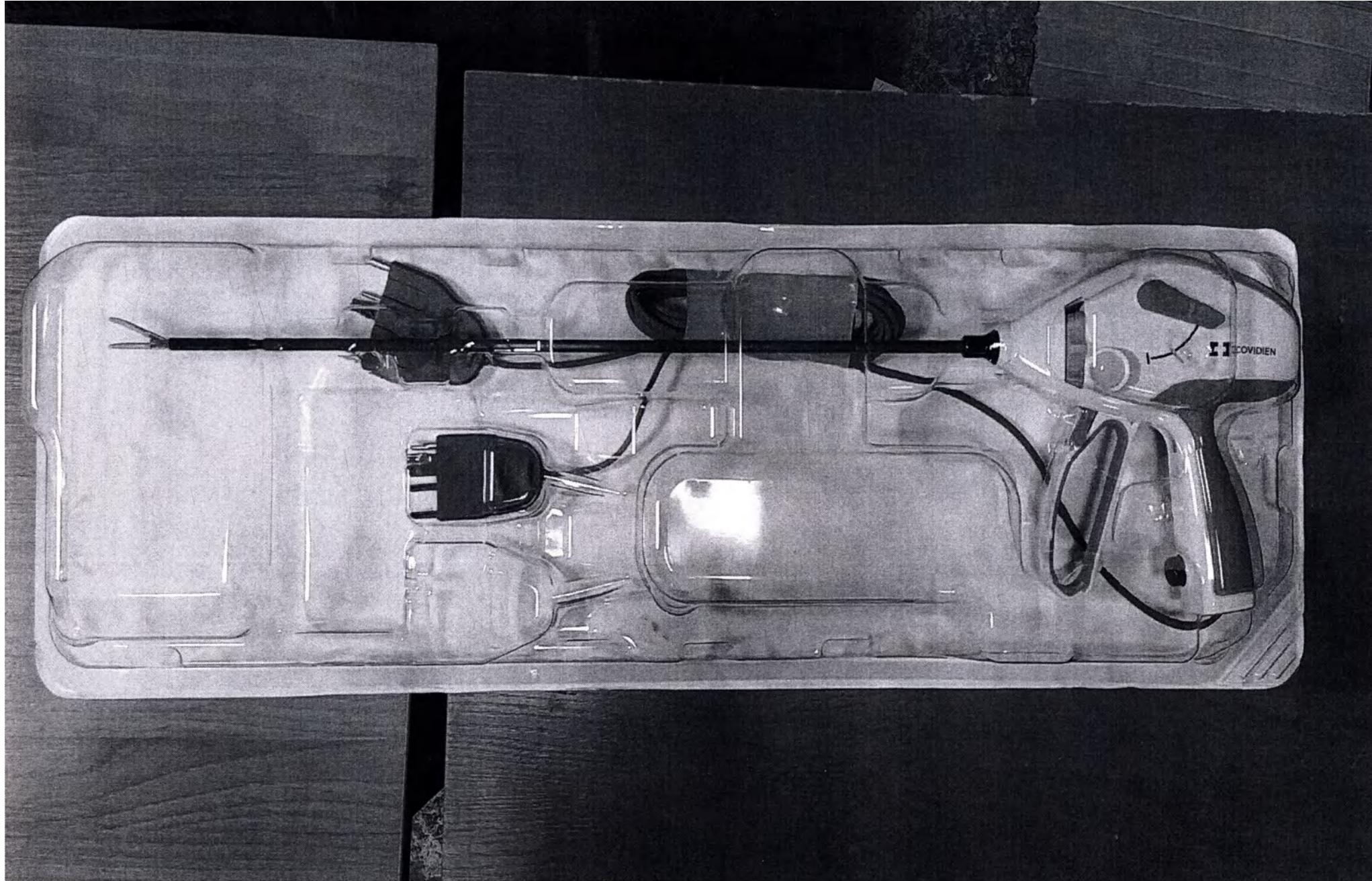
Фото 7. Лапароскопический инструмент LigaSure для электролигирования и разделения тканей с выдвижным Г-образным крючком диаметр стержня 5 мм, длина стержня 44 см; — В упаковке
