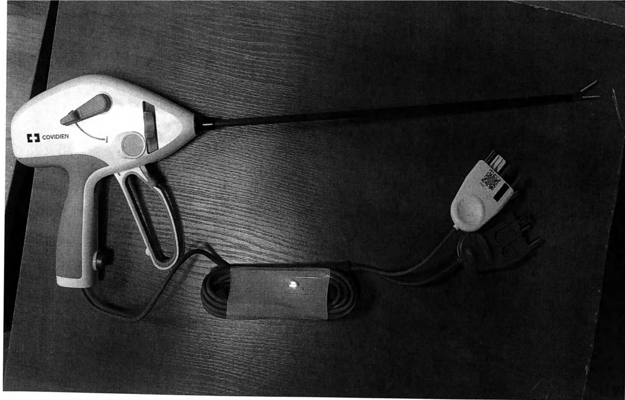
Фото 1. Лапароскопический инструмент LigaSure для электролигирования и разделения тканей с выдвижным Г-образным крючком диаметр стержня 5 мм, длина стержня 37 см; — Без упаковки
