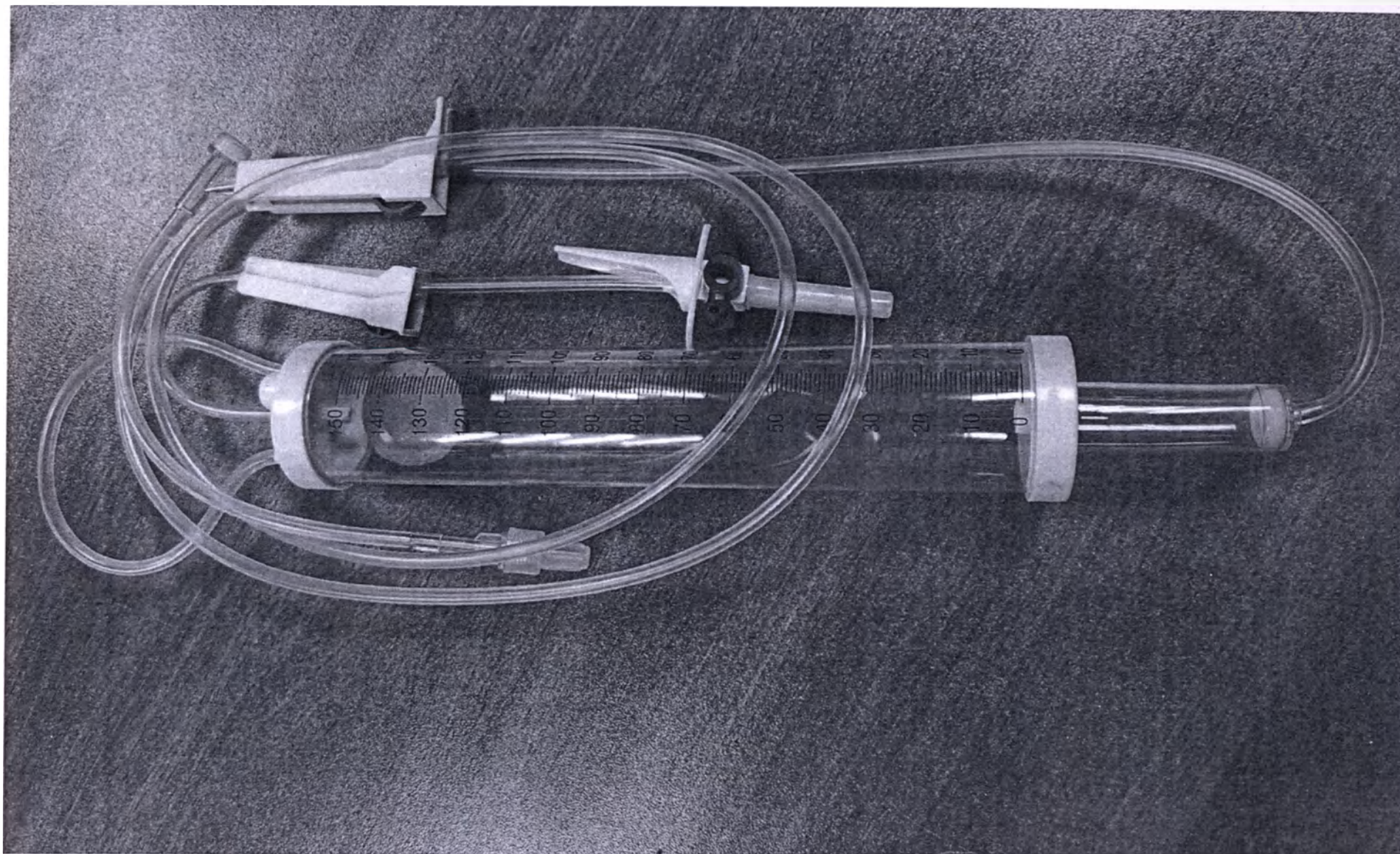
Устройство инфузионное с пластиковым шипом, с коннектором типа Луер-Лок, длина трубки 160 см, со встроенным воздуховодом и воздушным фильтром, с роликовым регулятором скорости потока, без иглы, с прозрачной трубкой, с Y-портом, с мерным сосудом с инъекционным портом, с маленькой капельной камерой. Изделие без упаковки.
