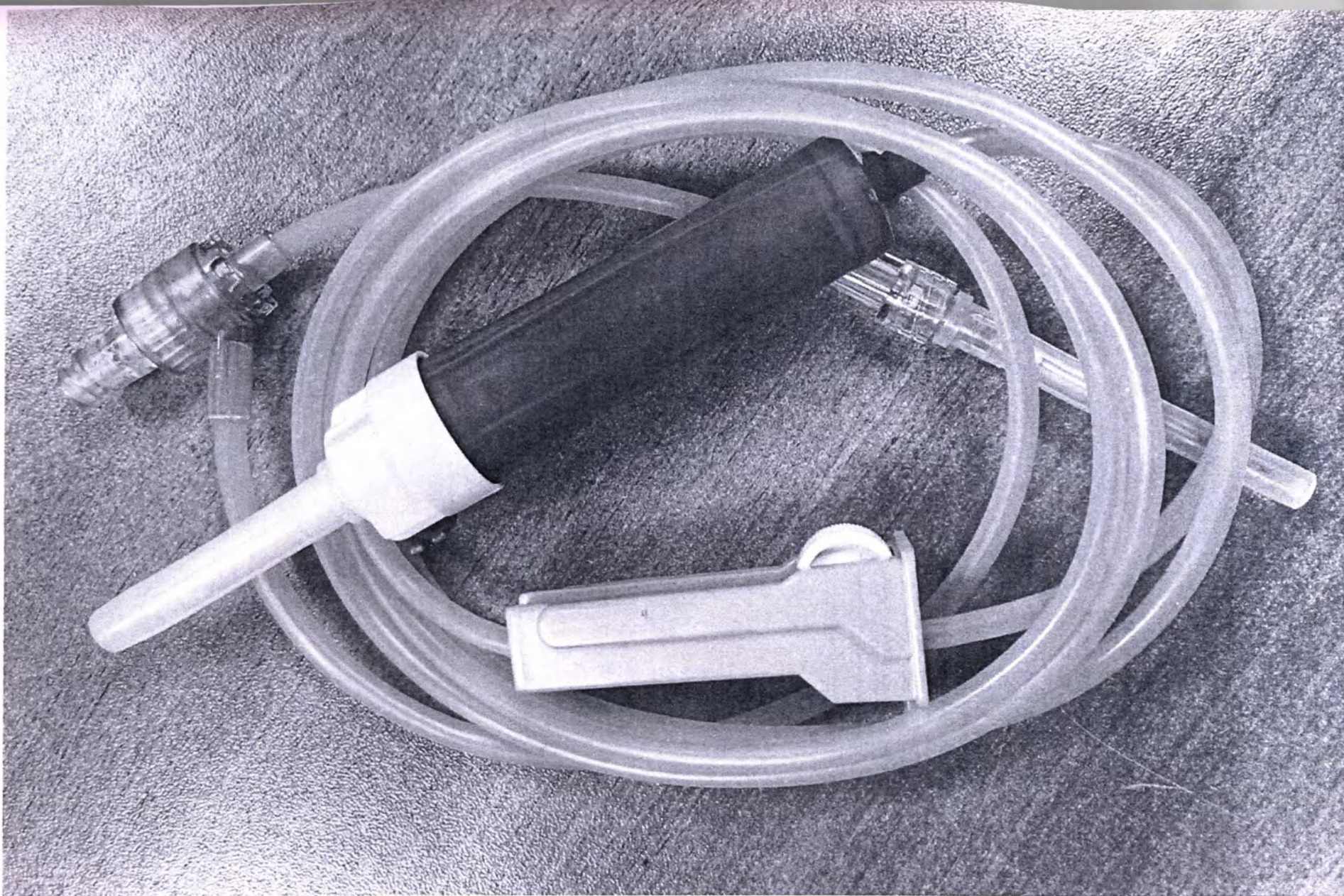
Устройство инфузионное с пластиковым шипом, с коннектором типа Луер-Лок, длина трубки 150 см, со встроенным воздуховодом и воздушным фильтром, с роликовым регулятором скорости потока, с одной стандартной инъекционной иглой 21G x 1½" (0,8мм x 40мм), со светозащитной трубкой, с портом безыгольного доступа, со средней капельной камерой. Изделие без упаковки.
