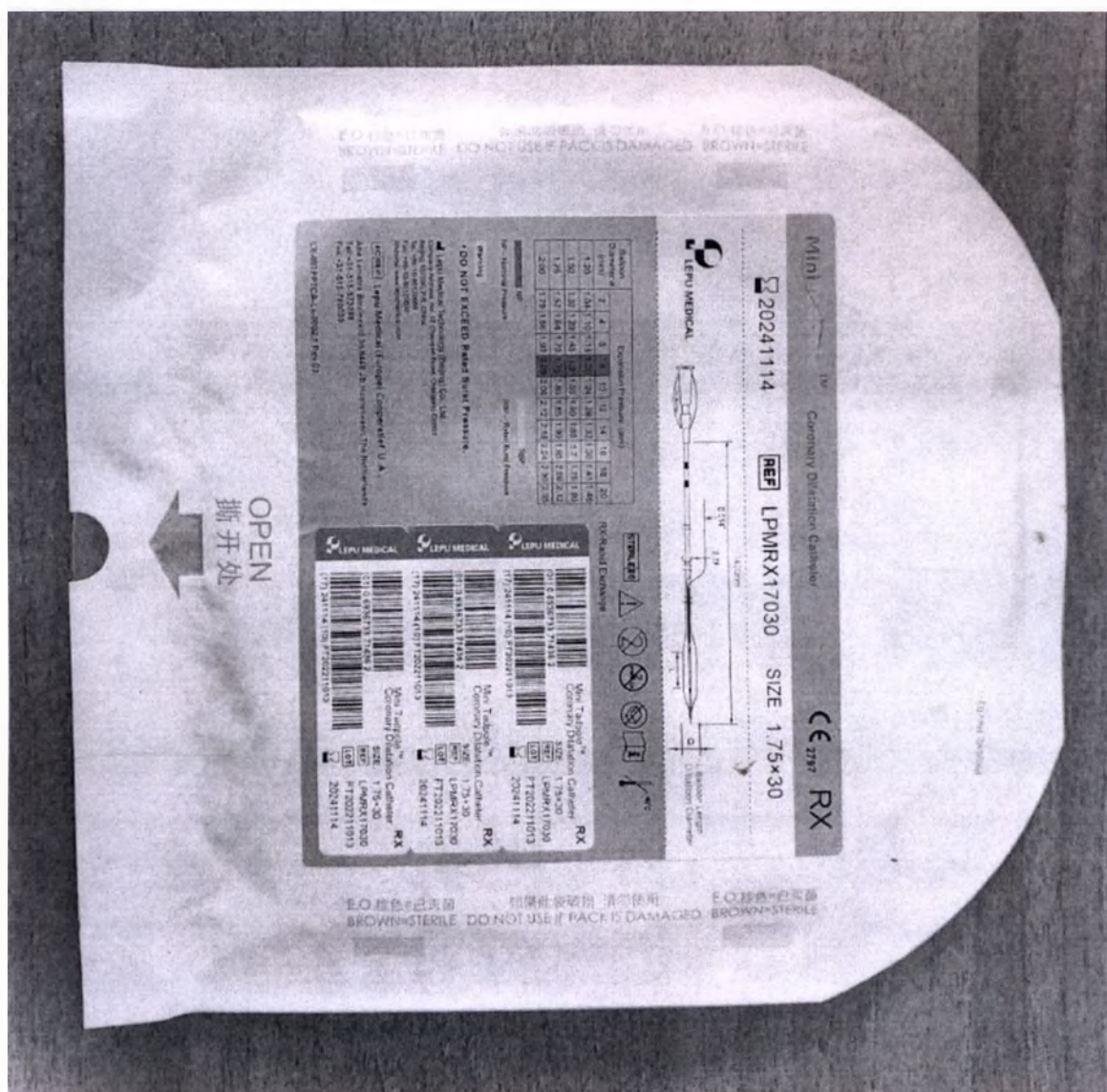
Фотографическое изображение 3 Катетер коронарный дилатационный Mini Tadpole Стерильная индивидуальная упаковка с маркировкой
