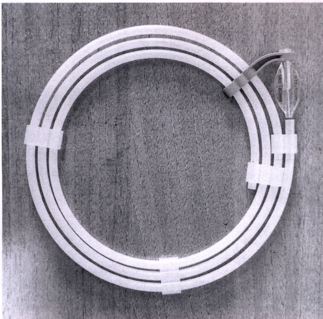
Фотографическое изображение 1 Катетер коронарный дилатационный Mini Tadpole в кольцевой защитной трубке
