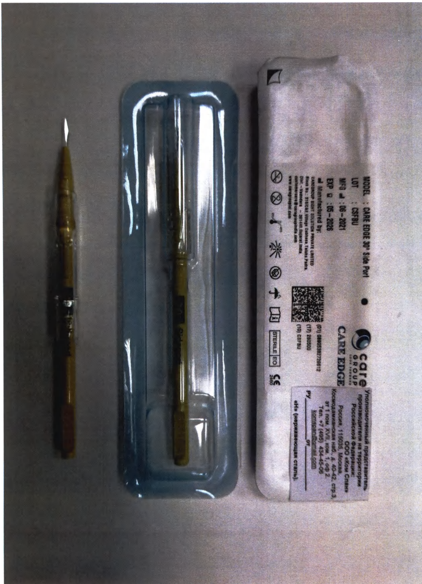
Нож офтальмологический одноразовый стерильный с одной режущей кромкой Care Edge Side Port, 30° (блистерная упаковка)
