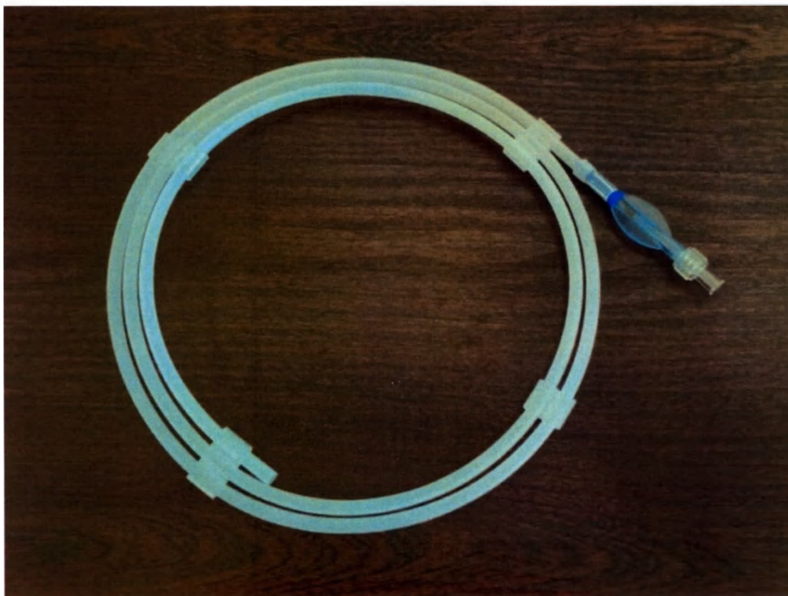
Фотографическое изображение 2. Катетер для аспирации тромбов THROMSWEEPER - в кольцевой защитной трубке
