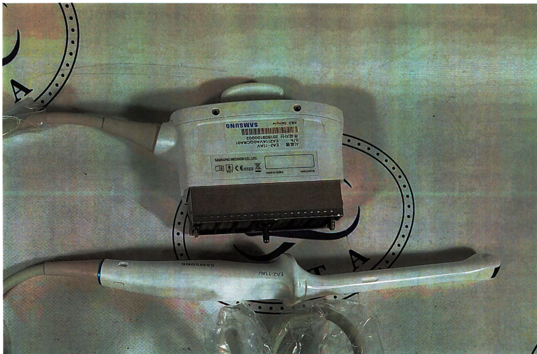
Датчик внутриматочной EA2-11AV
