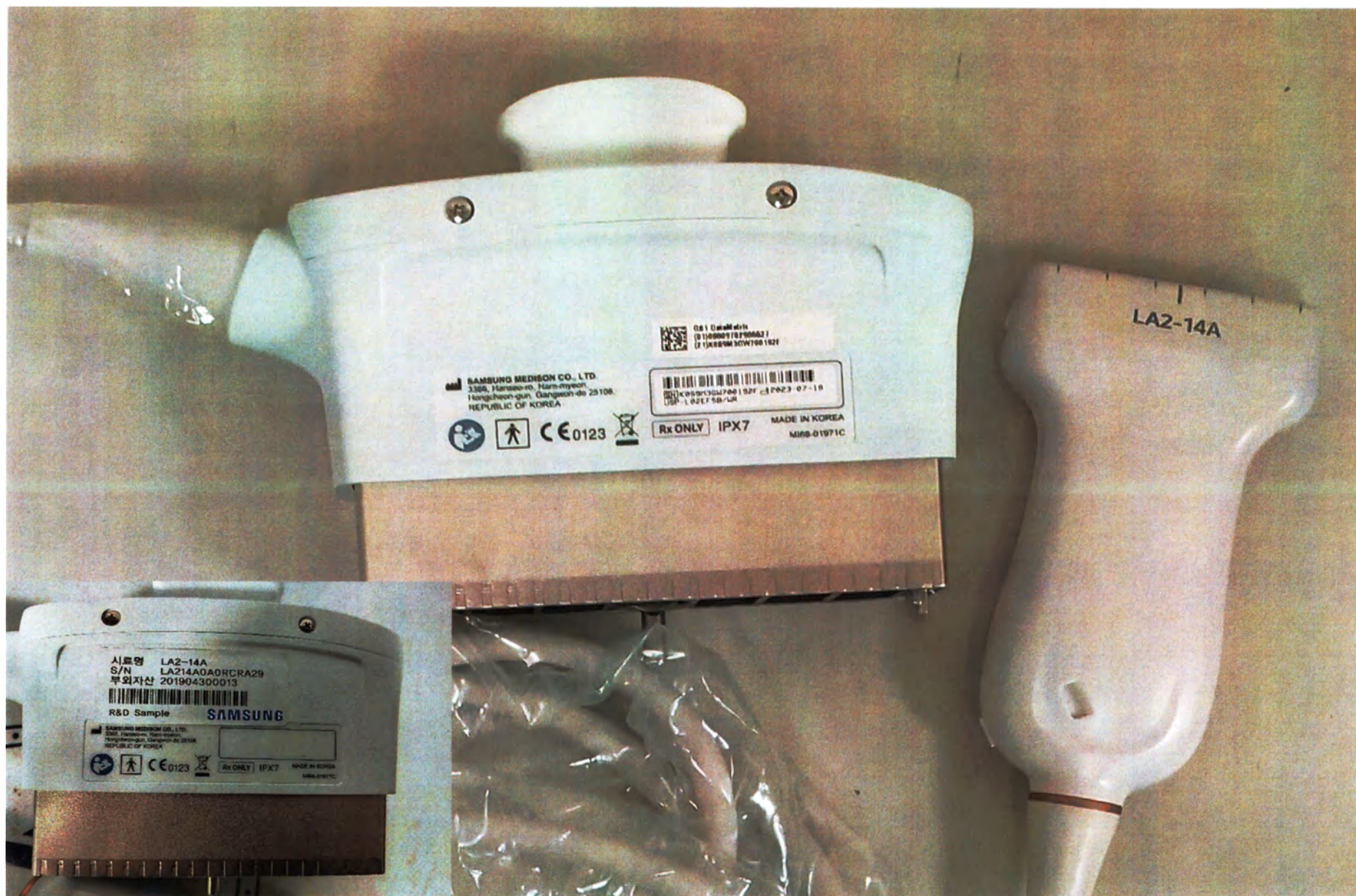
Датчик линейный LA2-14A
